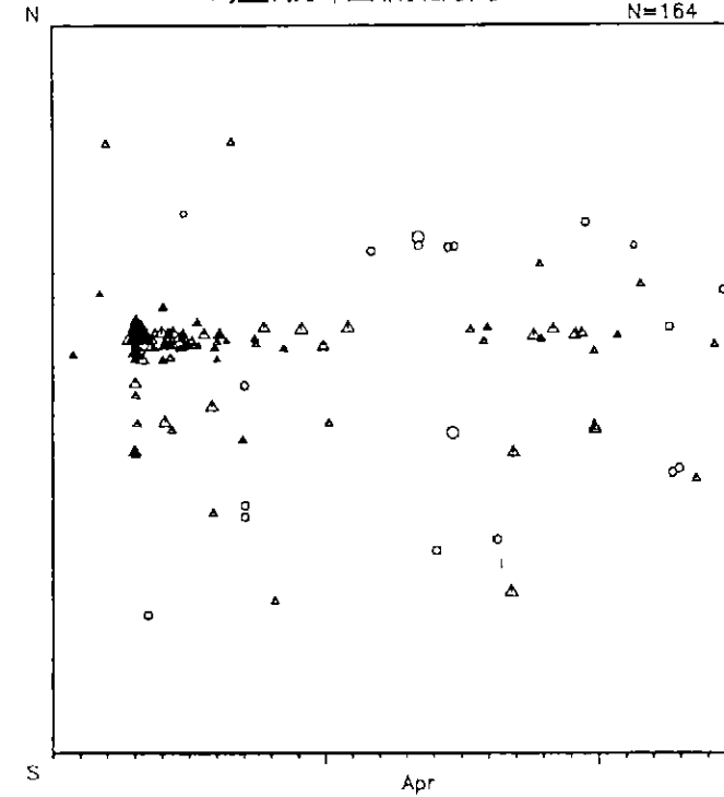
時空間分布図(南北方向)
