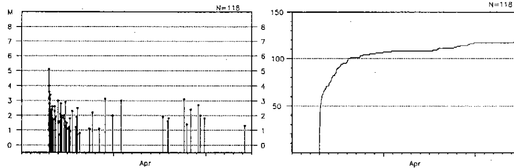
領域aの地震活動経過図(規模)
