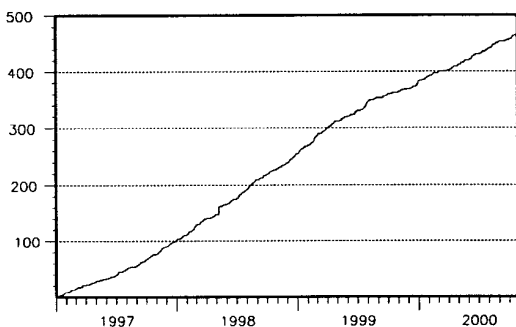
地震回数積算図
