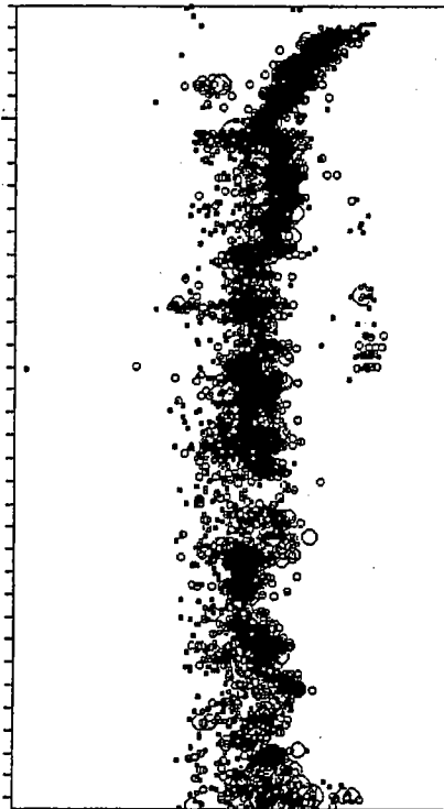
時空間分 布図(東 西方向)
