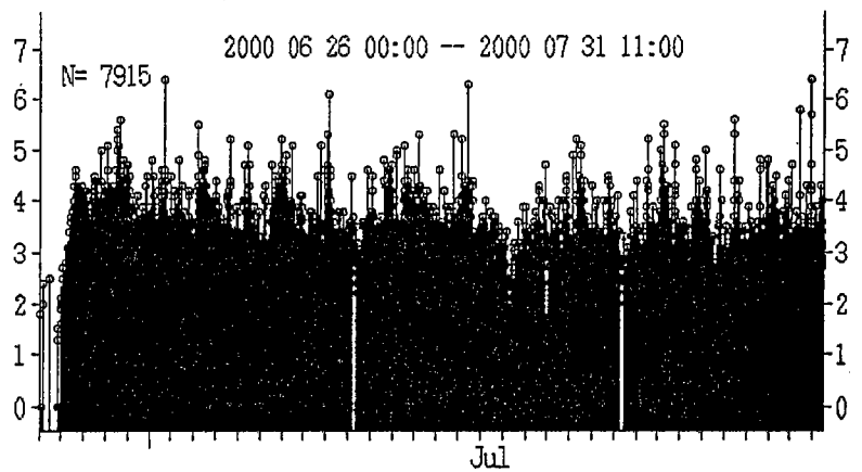
地震活動経過図(規模)
