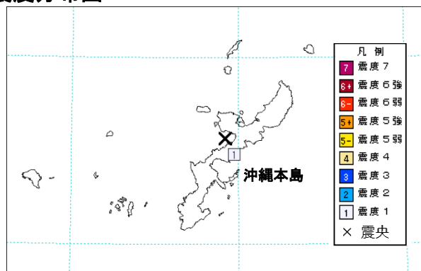
5月2日15時50分 沖縄本島近海 深さ12km M3.0
