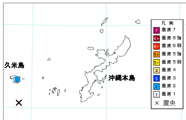
5月22日15時33分 沖縄本島近海 深さ59km M3.9
