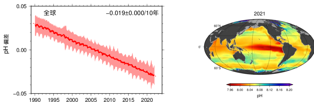
図 2.12-9 全球の表面海水中的の水素イオン濃度指数 (pH) 偏差の長期変化（左図）と 2021 年における pH 分布図（右図） 72
