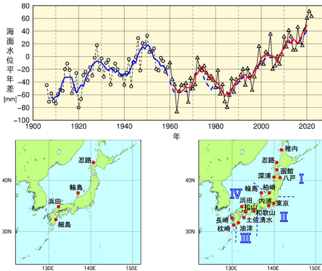
図 2.10-1 日本沿岸の年平均海面水位の経年変化（1906～2022 年、上图）と検潮所位置図（左下图、右下图）
