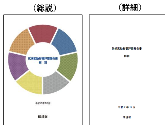
図 コラム 7.1 気候変動影響評価報告書 (2020（令和 2）年 12 月)
