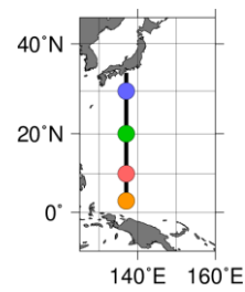
図 12-1.2 東経 137 度線における 表面海水 pH の長期変化
