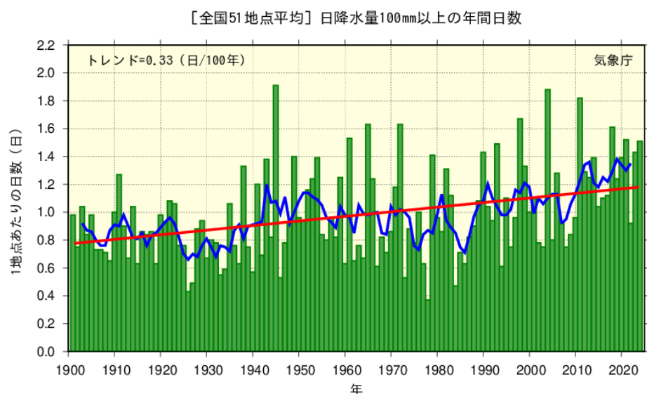
図 5-1.1 日降水量 100 mm 以上の年間日数の経年変化（1901～2024 年）
