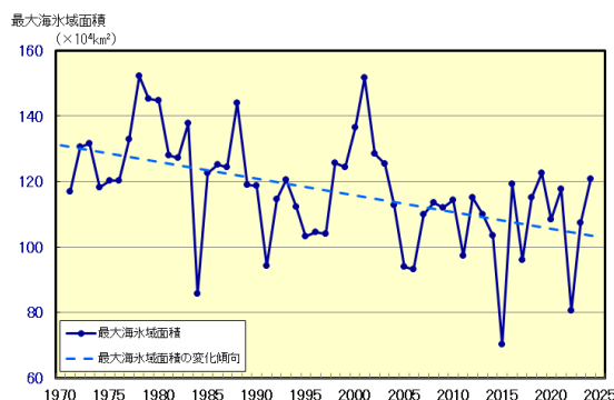
図 10-1.1 オホーツク海の水氷域面積の推移 (1971～2024 年)
