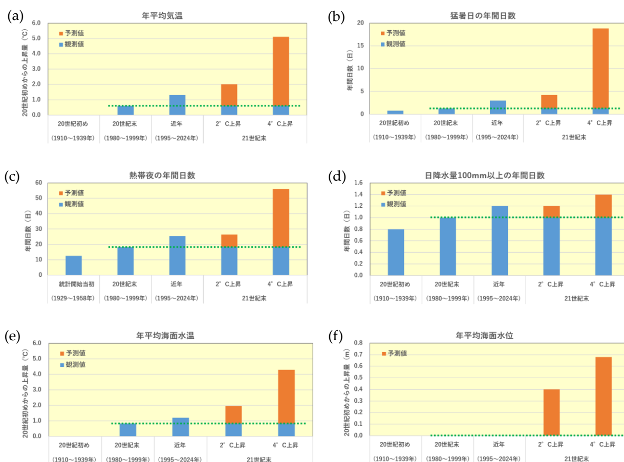
図 2.2 日本における (a) 年平均気温、(b) 猛暑日の年間日数、(c) 熱帯夜の年間日数、(d) 日降水量 100mm 以上の年間日数、(e) 年平均海面水温、(f) 年平均海面水位の過去から将来までの変化 青棒：観測値、橙棒：予測値、緑線：20 世紀末における観測値を示す。21 世紀末の値は、20 世紀末の観測値（緑線）に予測値を加算又は乗算したもの。
