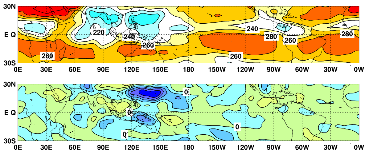
図 9 外向き長波放射量 (OLR) (上) 及び平年偏差 (下) の分布図 (2025 年 7 月)
