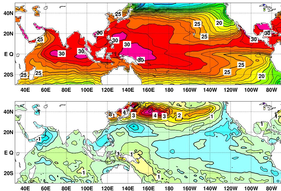
図4 2025年7月の海面水温図（上）及び平年偏差図（下）
