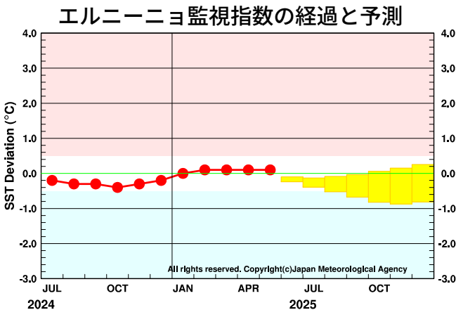
図 1 エルニーニョ監視海域の監視指数（海面水温の基準値との差）の 5 か月移動平均値の経過と予測 エルニーニョ監視海域の監視指数（海面水温の基準値との差）の 5 か月移動平均値について、5 月までの経過（観測値）を折れ線グラフで、大気海洋結合モデルによる予測結果（70%の確率で入ると予想される範囲）をボックスで示している。監視指数の 5 か月移動平均値が赤（+0.5°C 以上）／青（-0.5°C 以下）の範囲に入っている状態で 6 か月以上持続した場合に、エルニーニョ／ラニーニャ現象の発生としている。エルニーニョ監視海域の海面水温の基準値はその年の前年までの 30 年間の各月の平均値。
