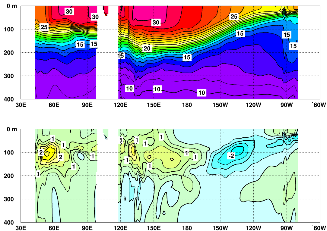
図5 2025年7月のインド洋から太平洋の赤道に沿った水温（上）及び平年偏差（下）の断面図
