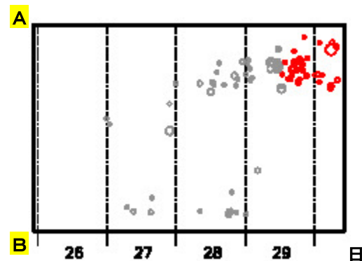
震央分布図の矩形内の時空間断面図
