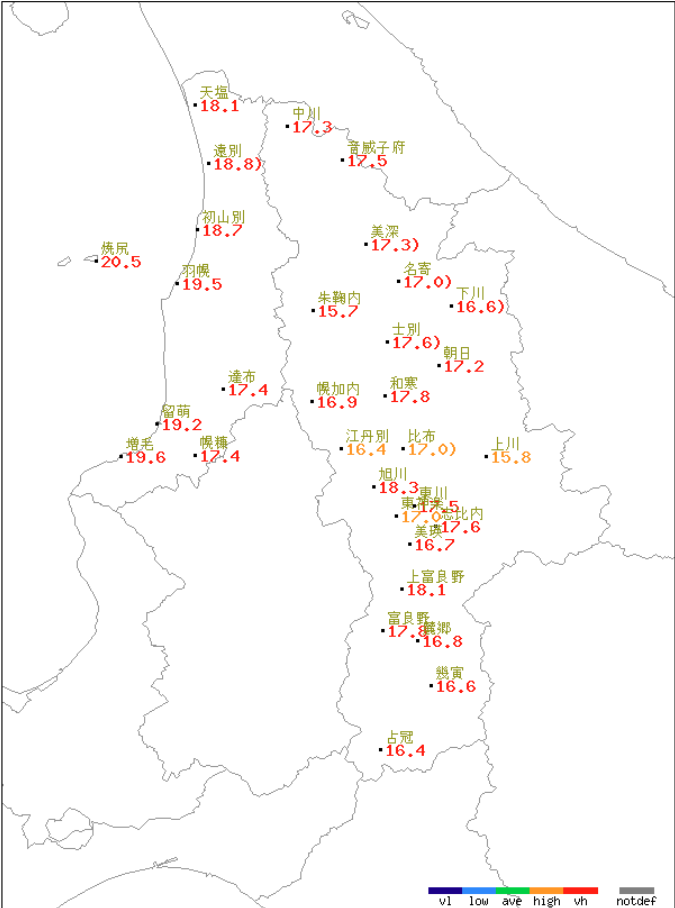
アメダス月別値 2025年9月 平均気温(℃)
