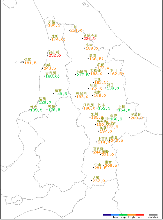
アメダス月別値 2025年9月 降水量(mm)
