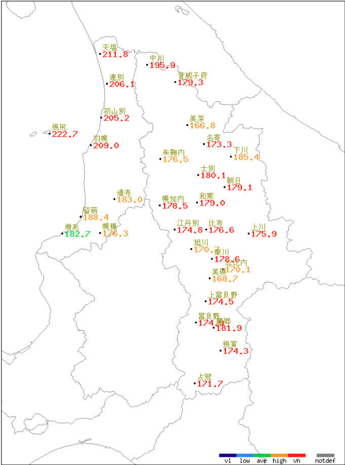
アメダス月別値 2025年9月 日照時間(h)
