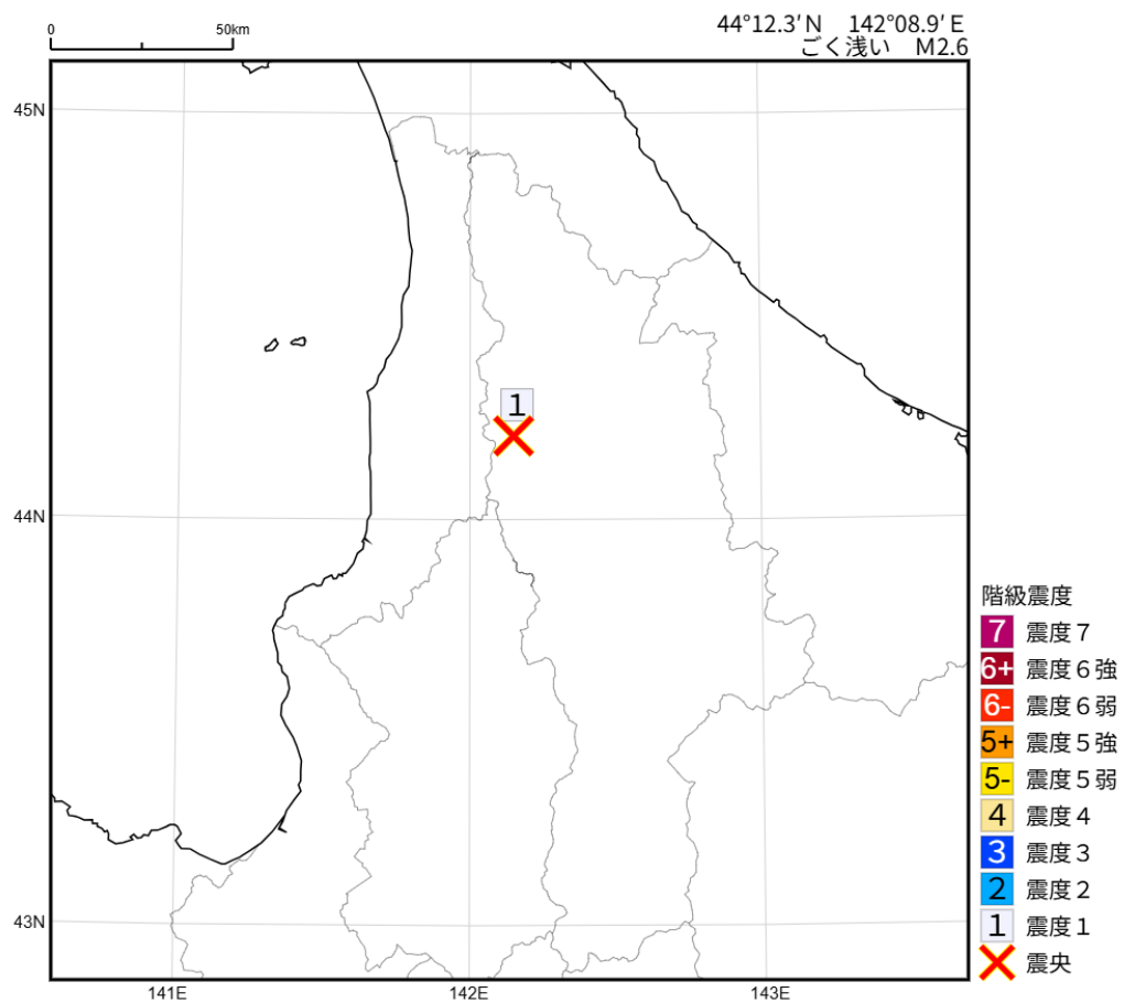
2026年 7月25日 22時52分 上川地方北部の地震の震度分布図
