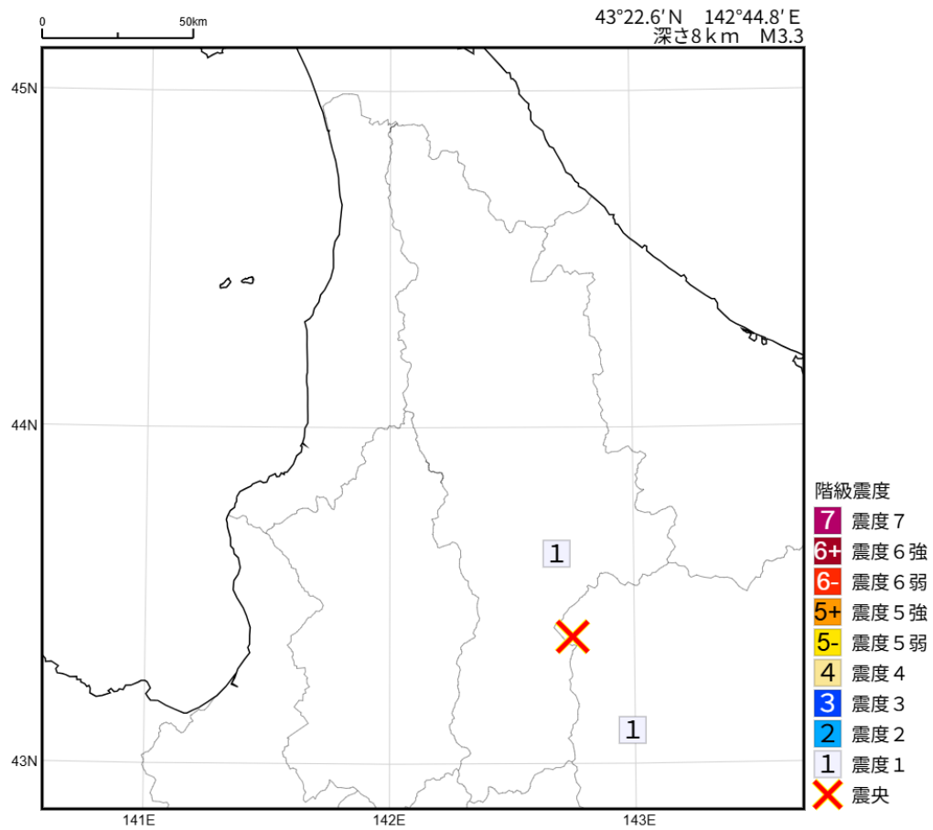
2026年 7月12日 23時13分 十勝地方北部の地震の震度分布図
