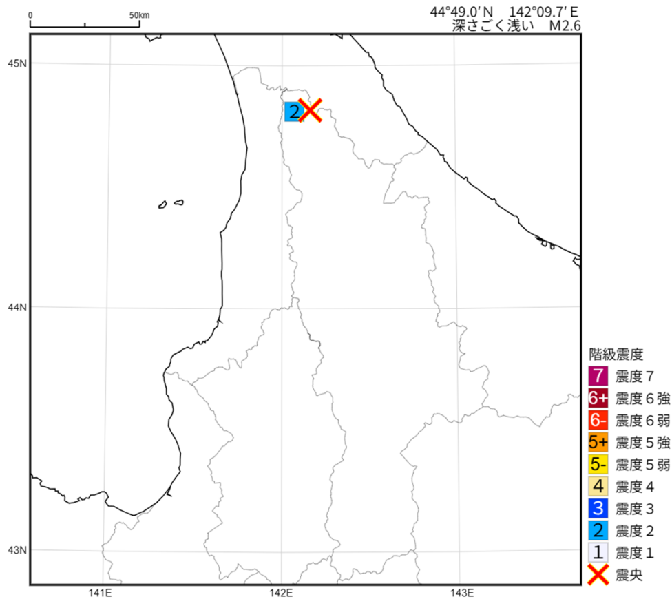
2025年11月19日 21時04分 上川地方北部の地震の震度分布図
