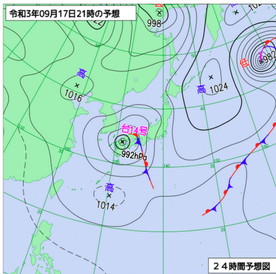
17日21時の予想図
