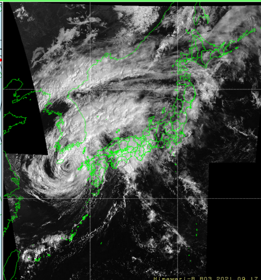
気象衛星ひまわり：画像 (17日9時)
