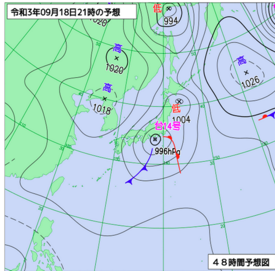
18日21時の予想図
