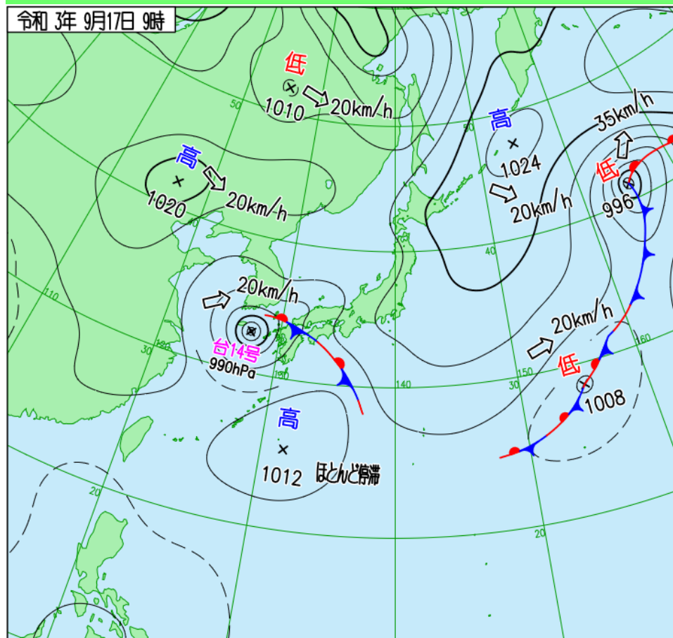
地上天気図 (17日9時)
