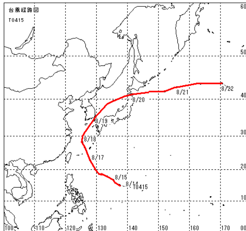
台風第15号の経路図
