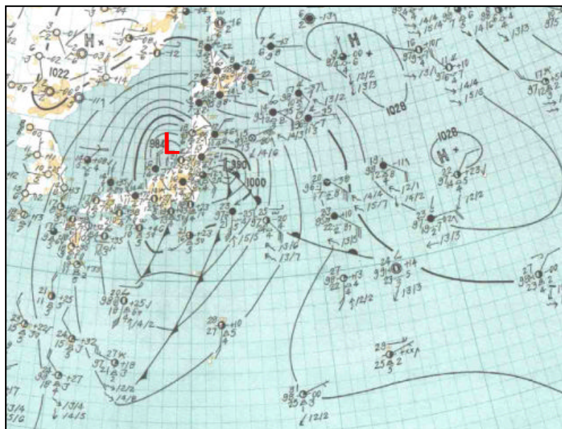
1967年10月28日09時の地上天気図
