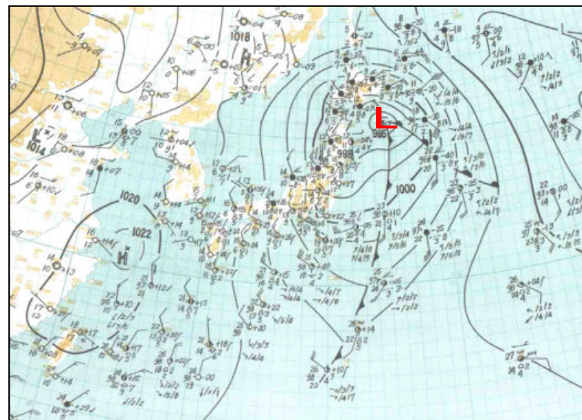
1967年10月28日21時の地上天気図
