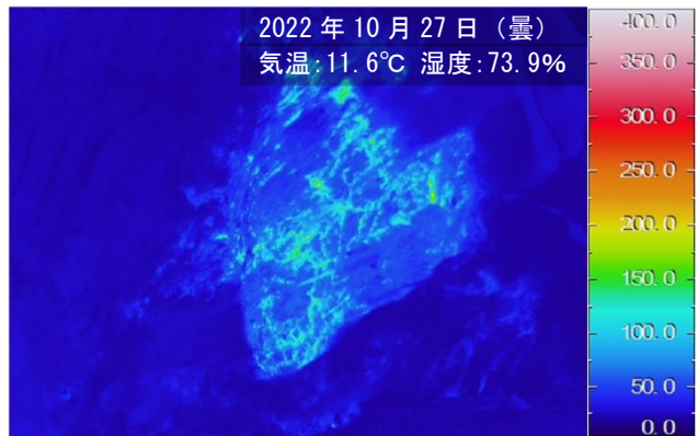
図4 阿蘇山 中岳第一火口内の南側火口壁の状況（火口南西側観測定点から観測）
