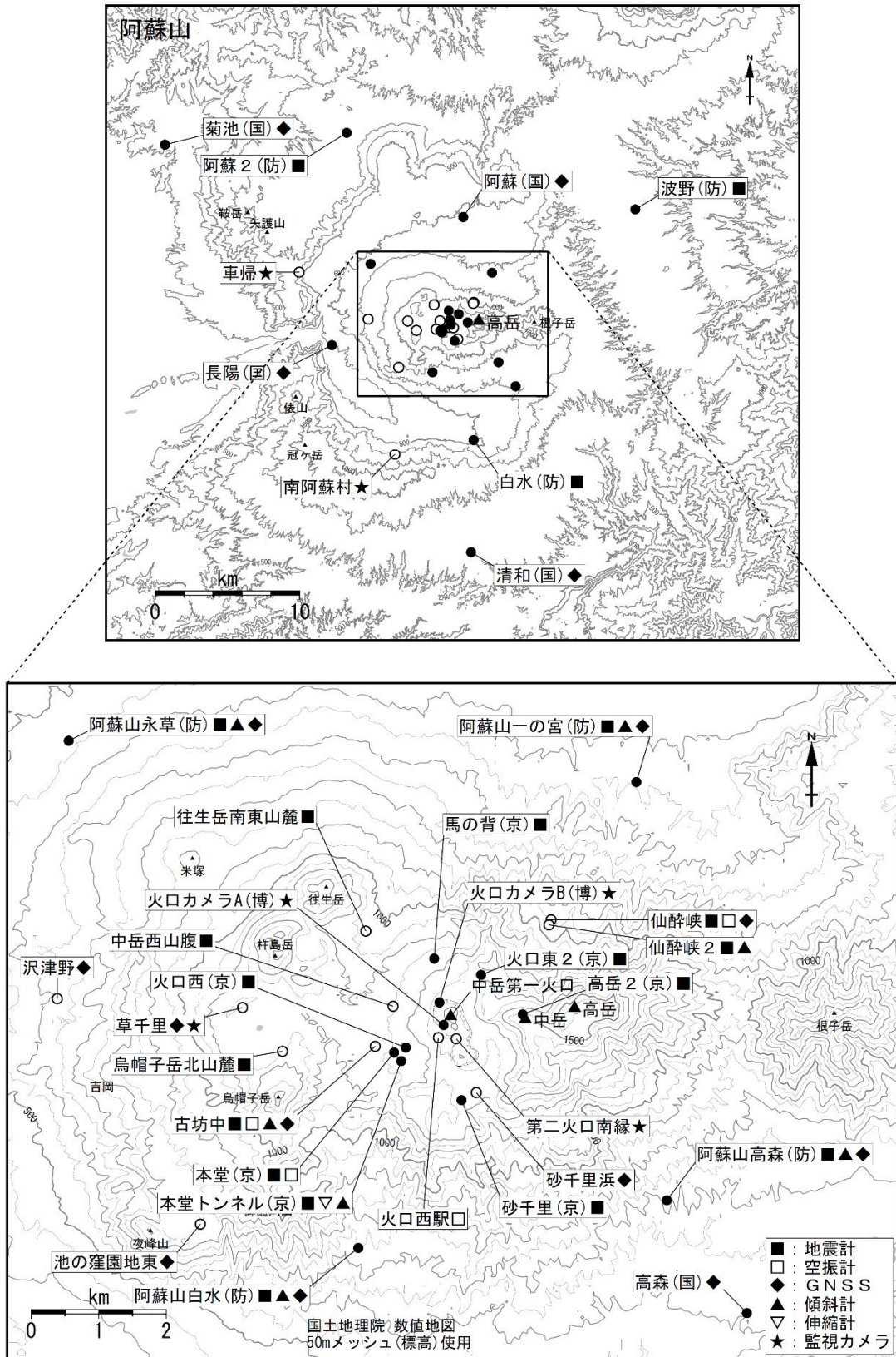
図12 阿蘇山 観測点配置図
