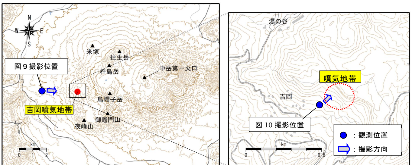
図11 阿蘇山 南阿蘇村吉岡の噴気地帯位置図
