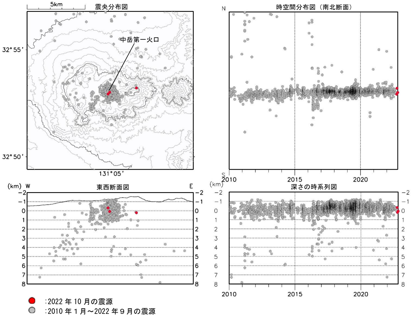
図6 阿蘇山 火山性地震の震源分布（2010年1月～2022年10月）
