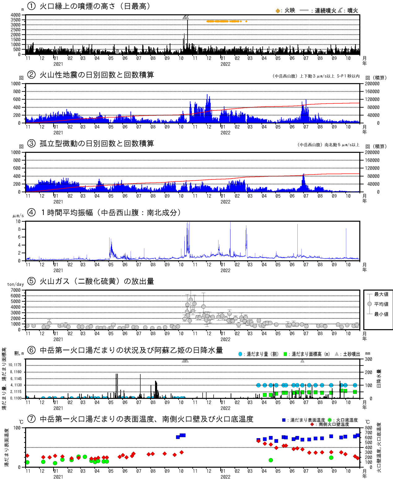
図5 阿蘇山 火山活動経過図（2020年11月～2022年10月）
