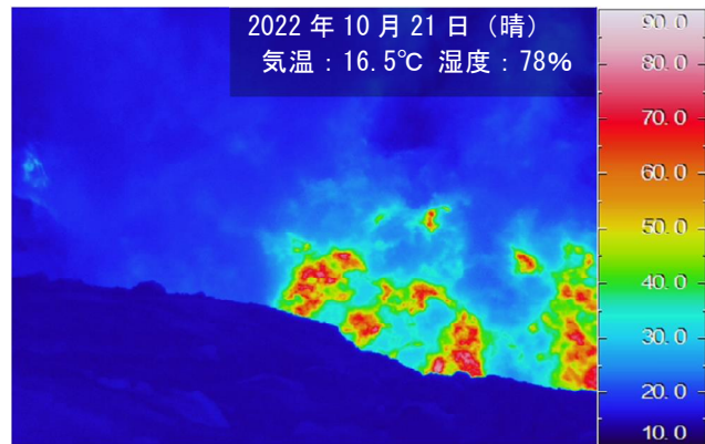
図3 阿蘇山 中岳第一火口内の湯だまりの状況（火口南西側観測定点から観測）
