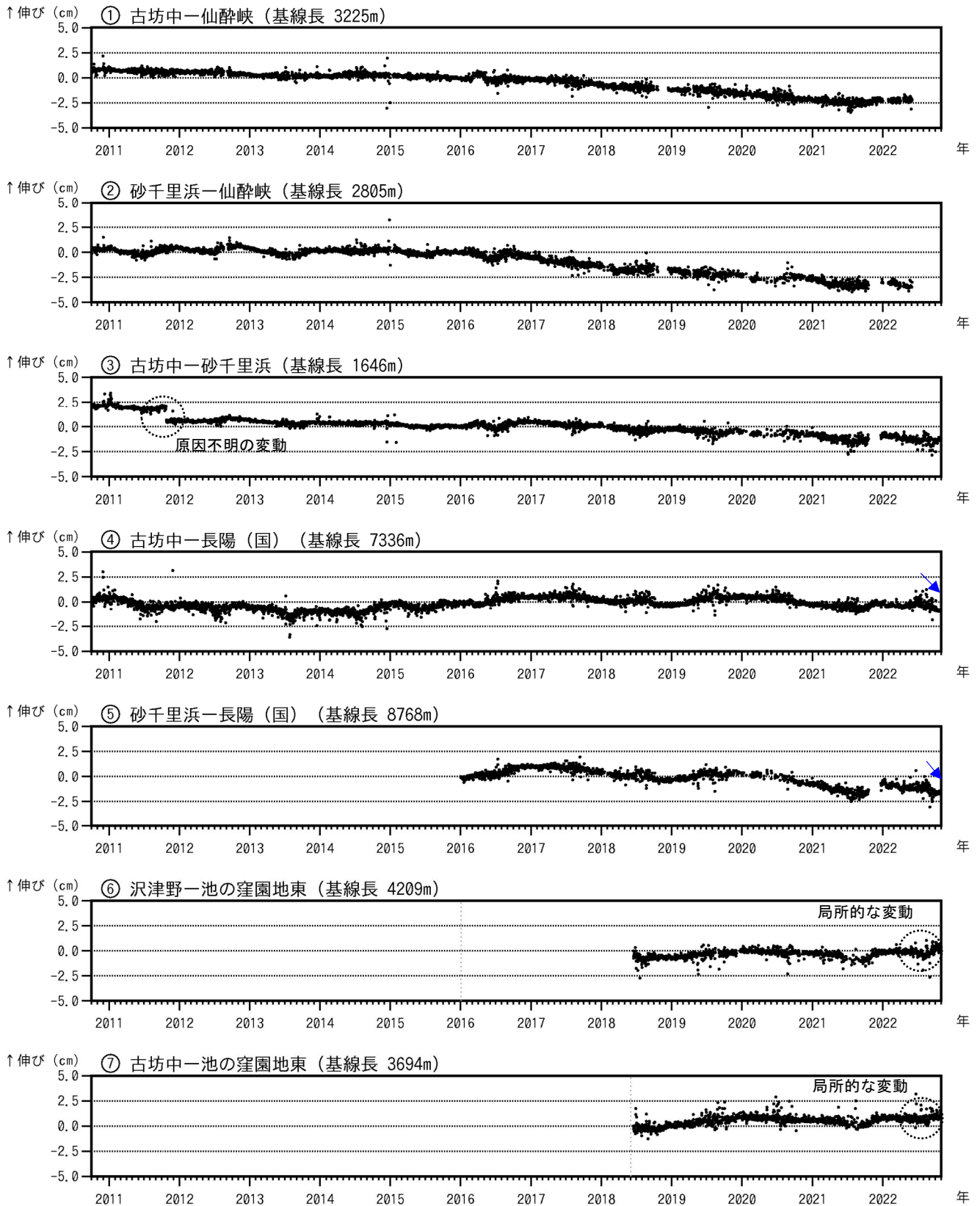
図7 阿蘇山 GNSS連続観測による基線長変化 (2010年10月~2022年10月)
