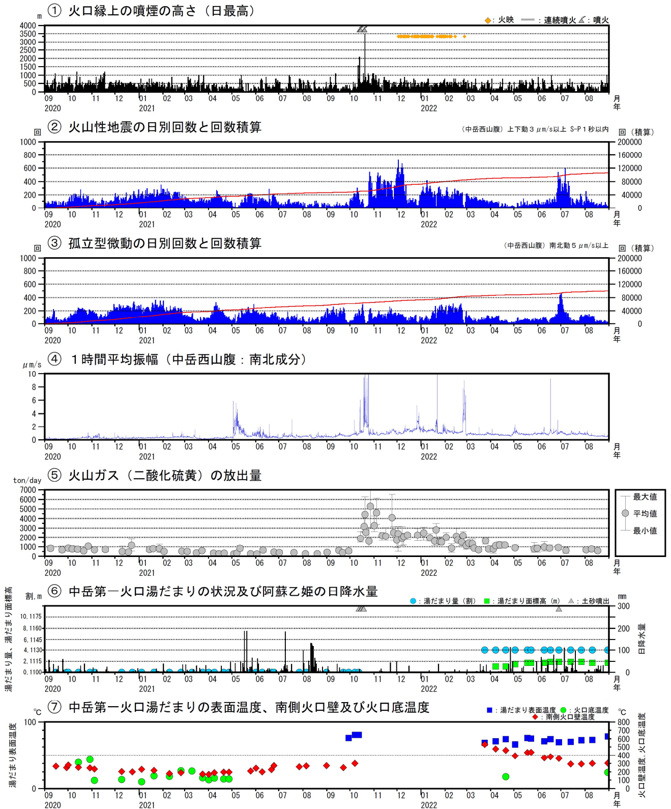
図6 阿蘇山 火山活動経過図（2020年9月～2022年8月）
