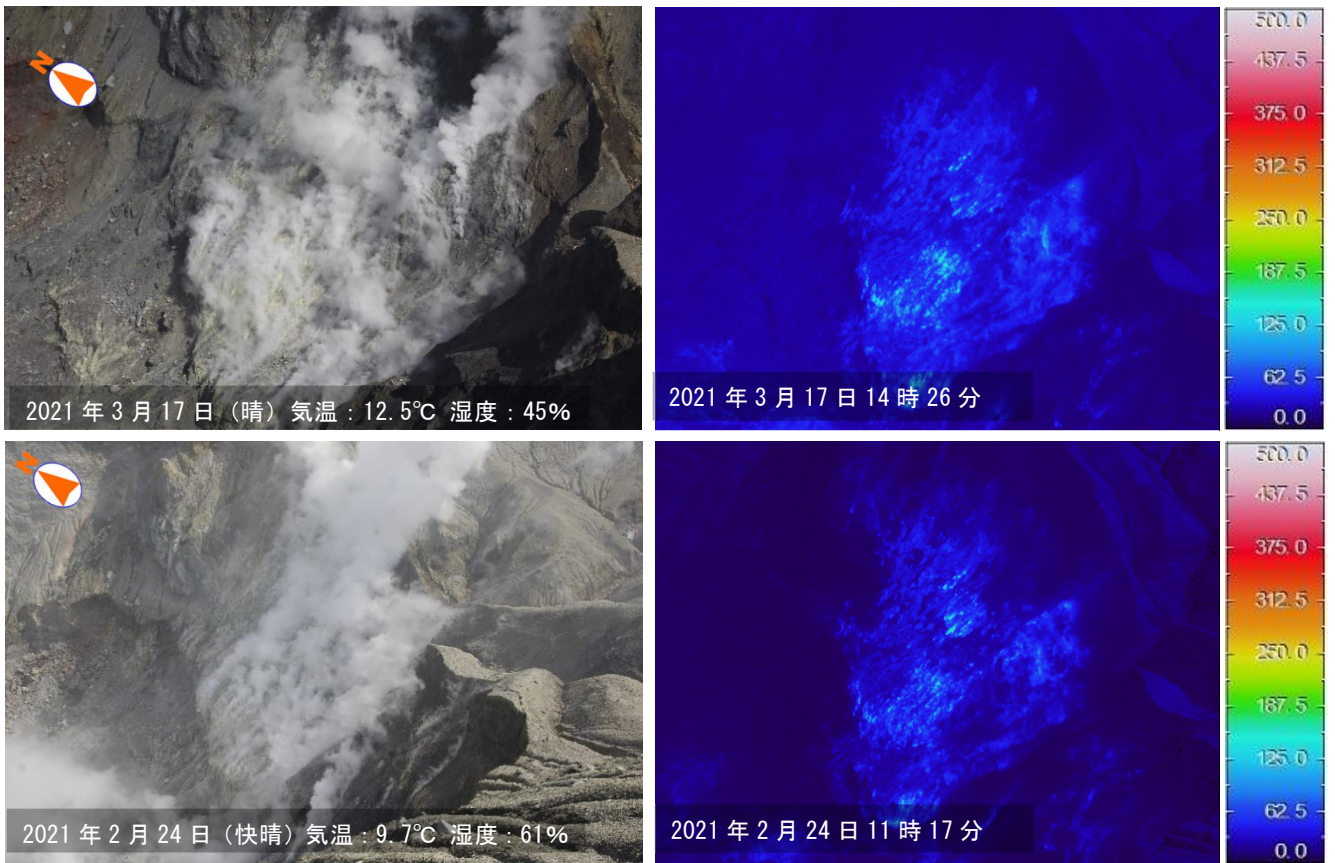
図6 阿蘇山 中岳第一火口内南側火口壁（火口南西側観測定点から観測） 赤外熱映像装置による観測では、火口壁の最高温度は176℃（2月：191℃）でした。
