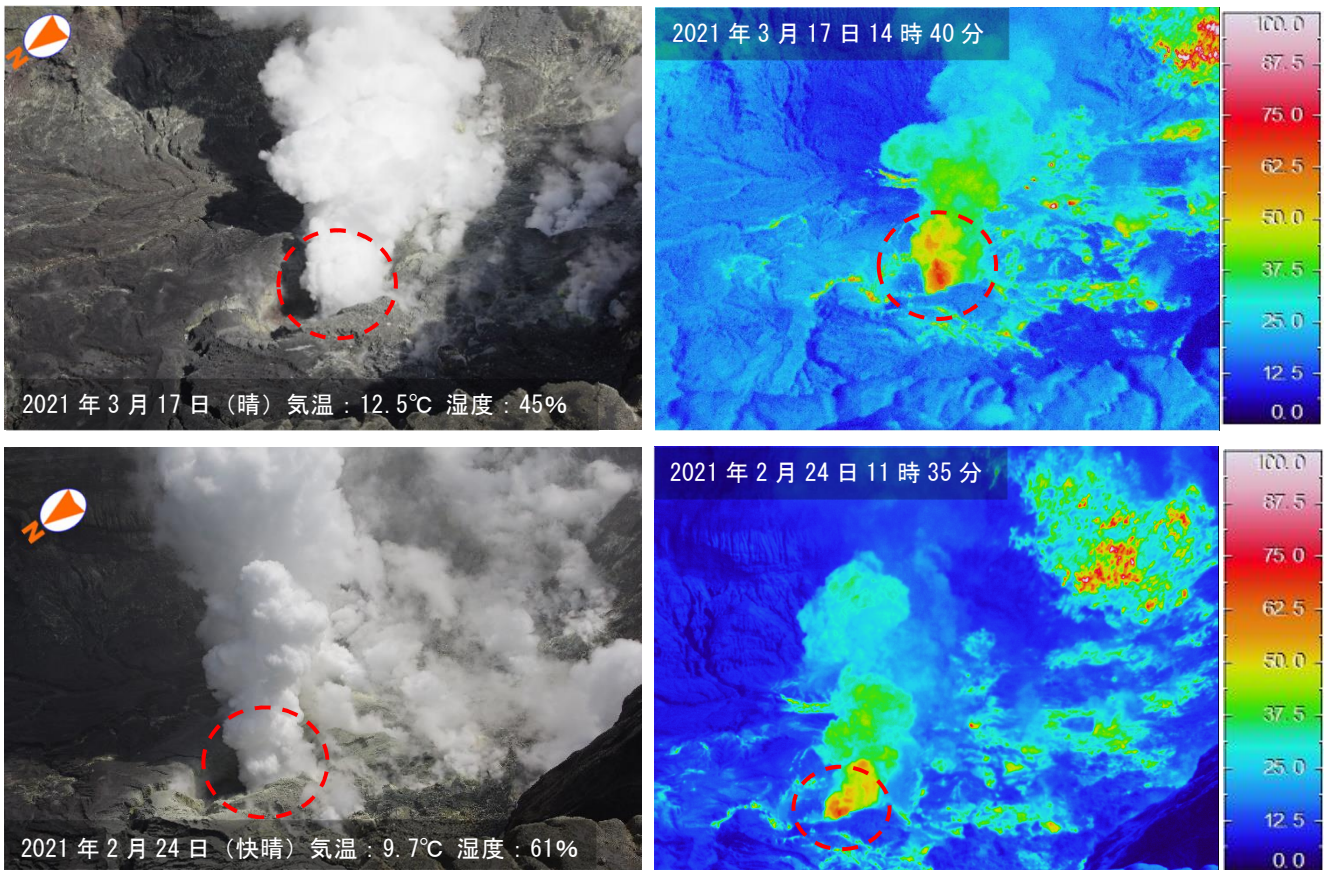
図4 阿蘇山 中岳第一火口内の状況（火口北西側観測定点から観測）
