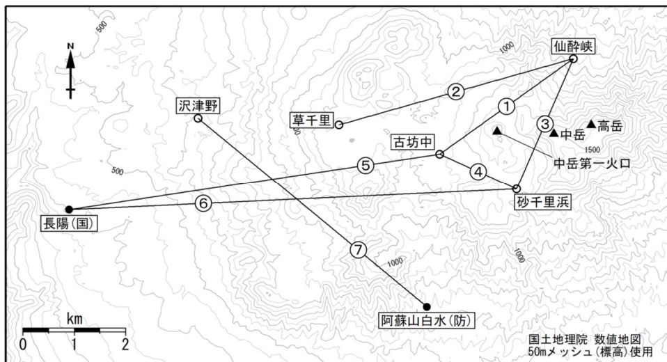
図10 阿蘇山 GNSS 連続観測点と基線番号
