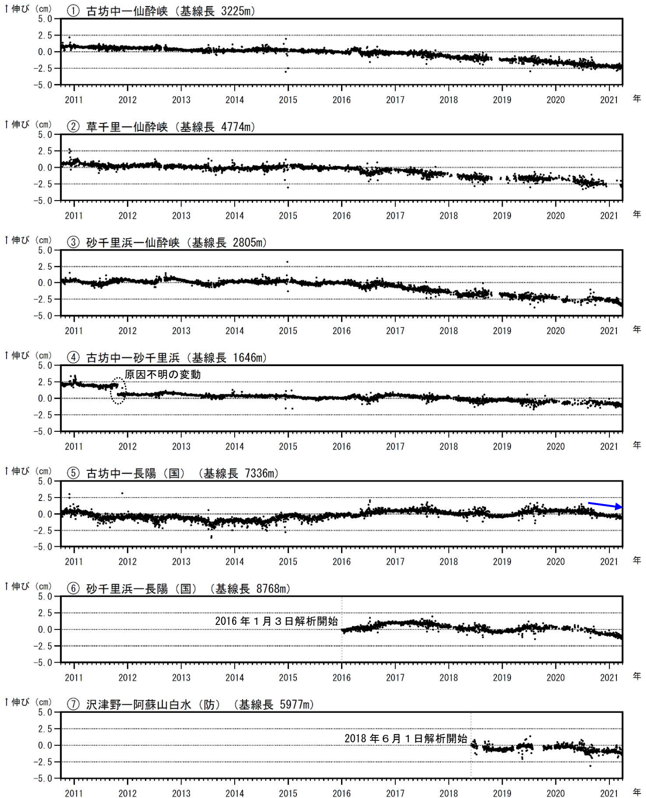
図 11 阿蘇山 GNSS 観測による基線長変化（2010年10月～2021年3月）
