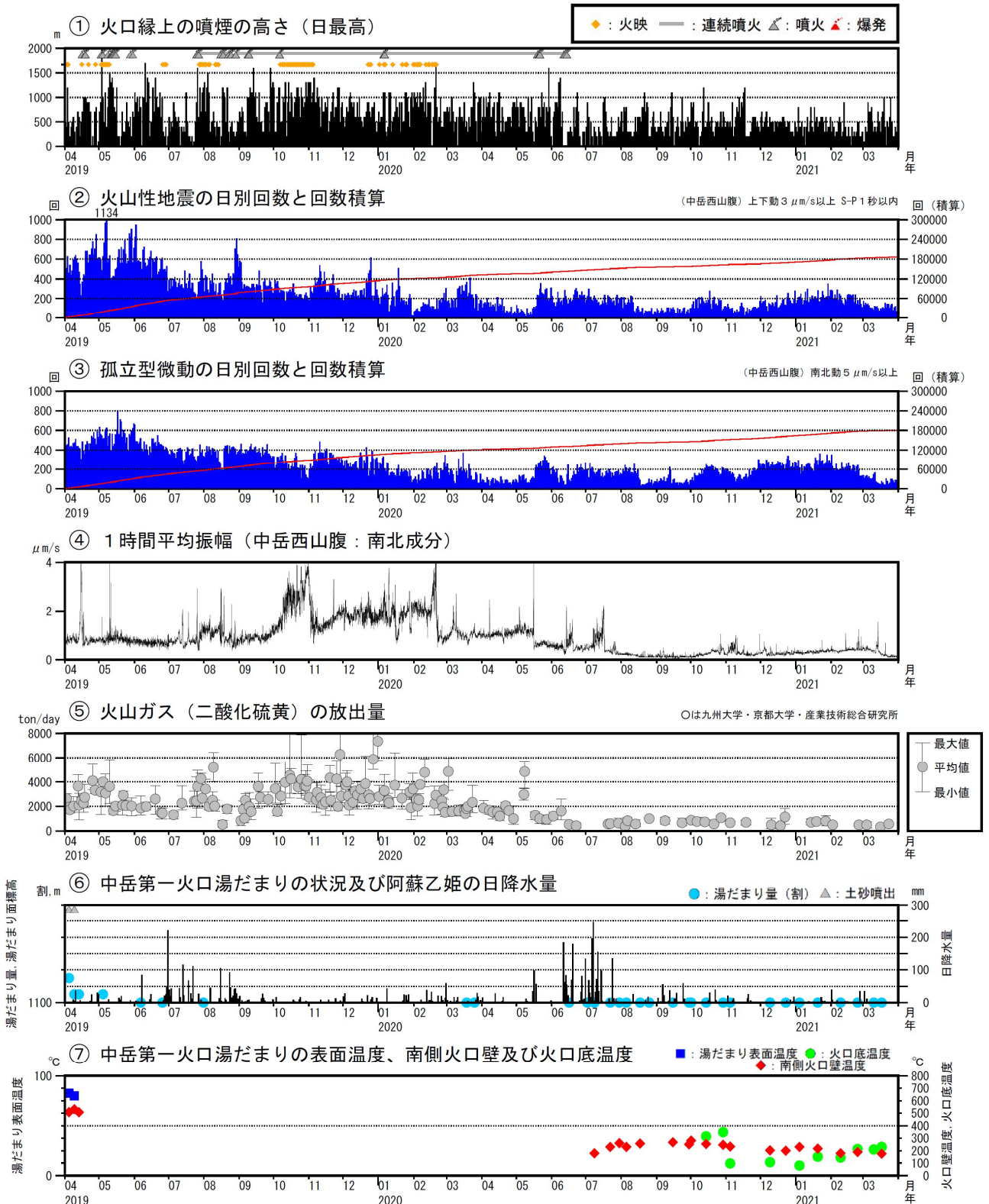
図7 阿蘇山 火山活動経過図（2019年4月～2021年3月）
