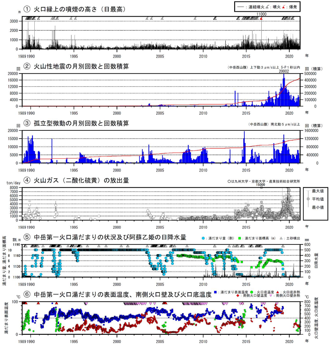
図8 阿蘇山 火山活動経過図（1989年1月～2021年3月）
