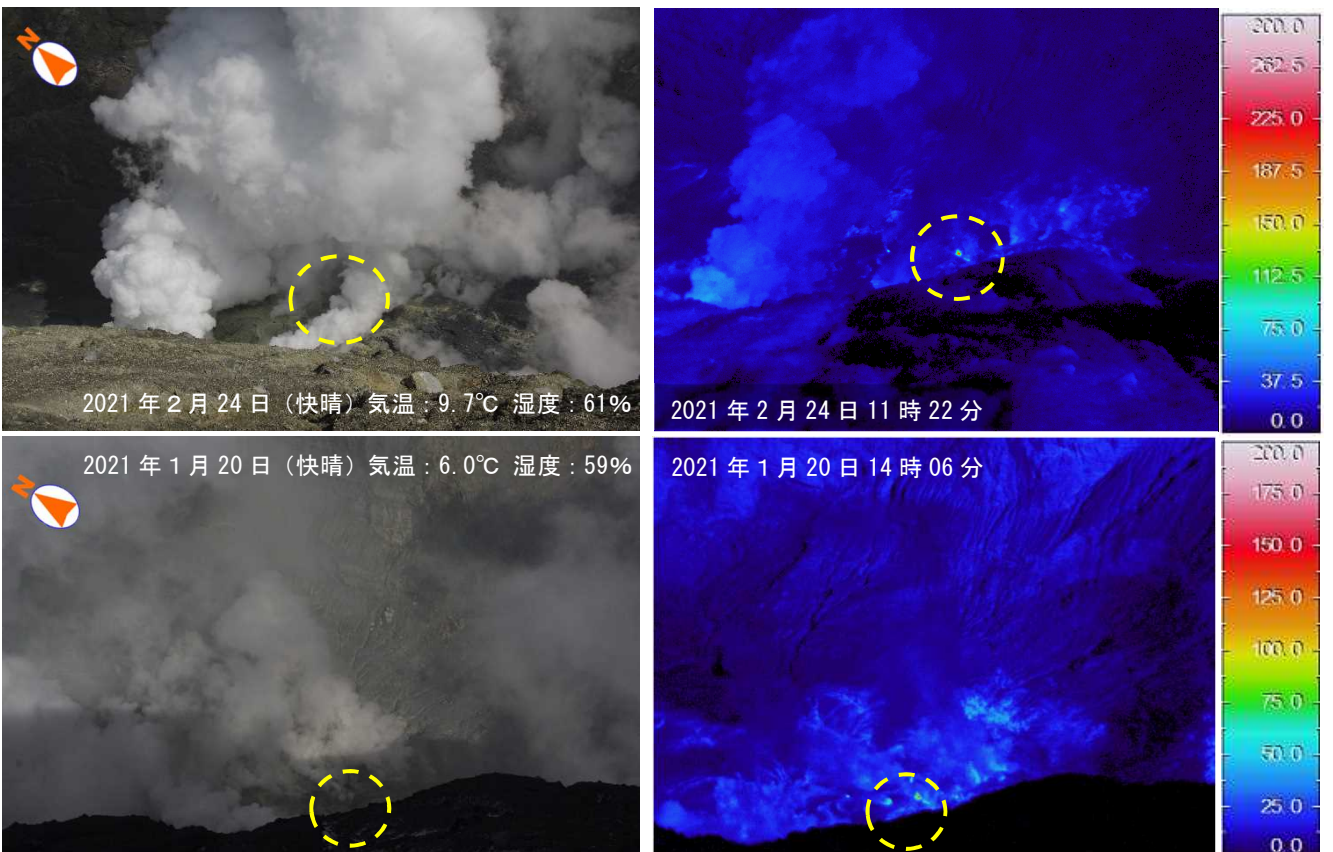
図5 阿蘇山 中岳第一火口内の状況（火口南西側観測定点から観測）
