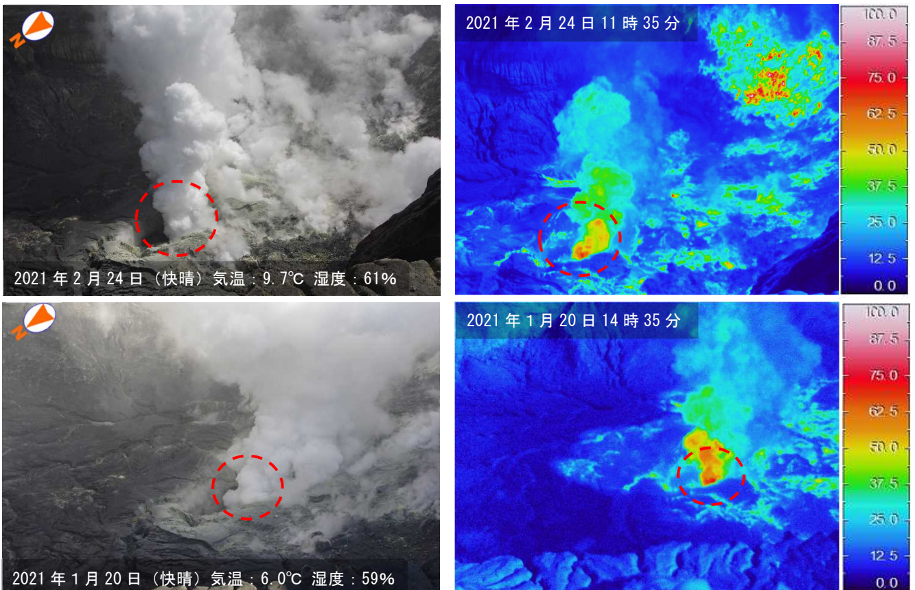
図4 阿蘇山 中岳第一火口内の状況（火口北西側観測定点から観測）
