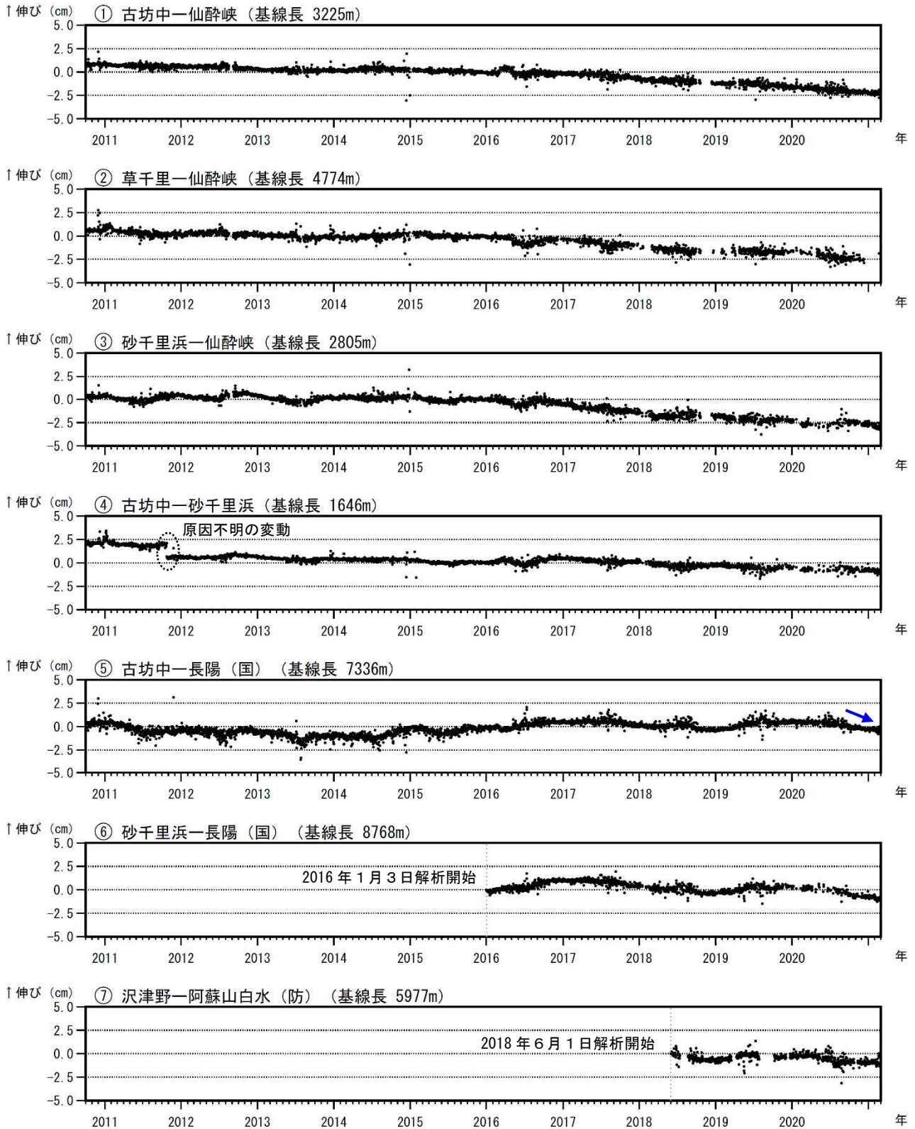
図 11 阿蘇山 GNSS 観測による基線長変化（2010年10月～2021年2月）
