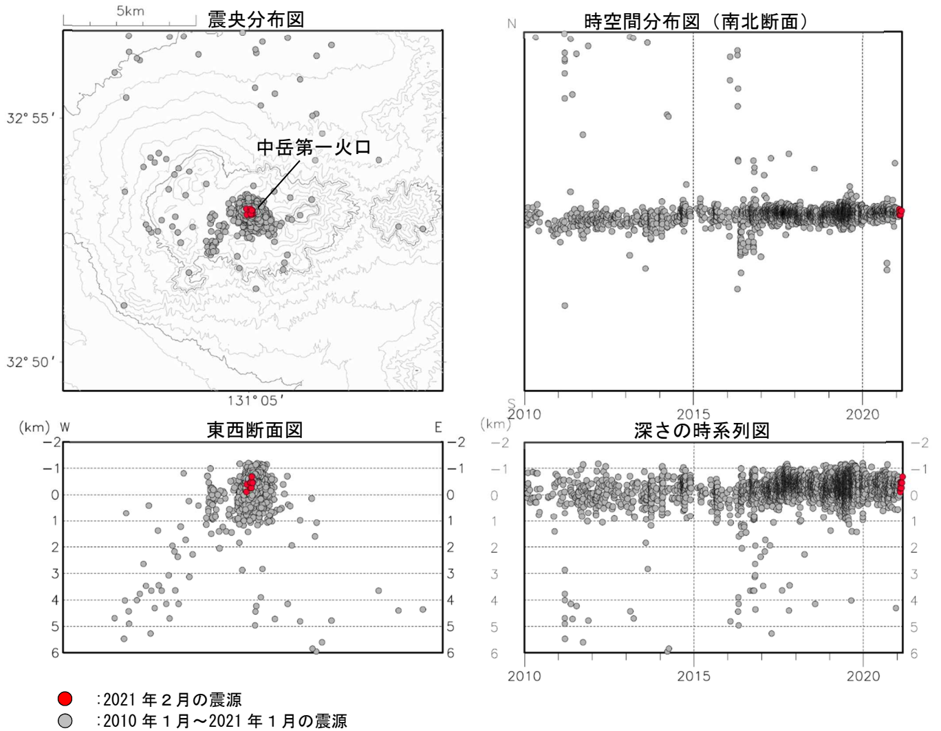
図10 阿蘇山 火山性地震の震源分布（2010年1月～2021年2月）
