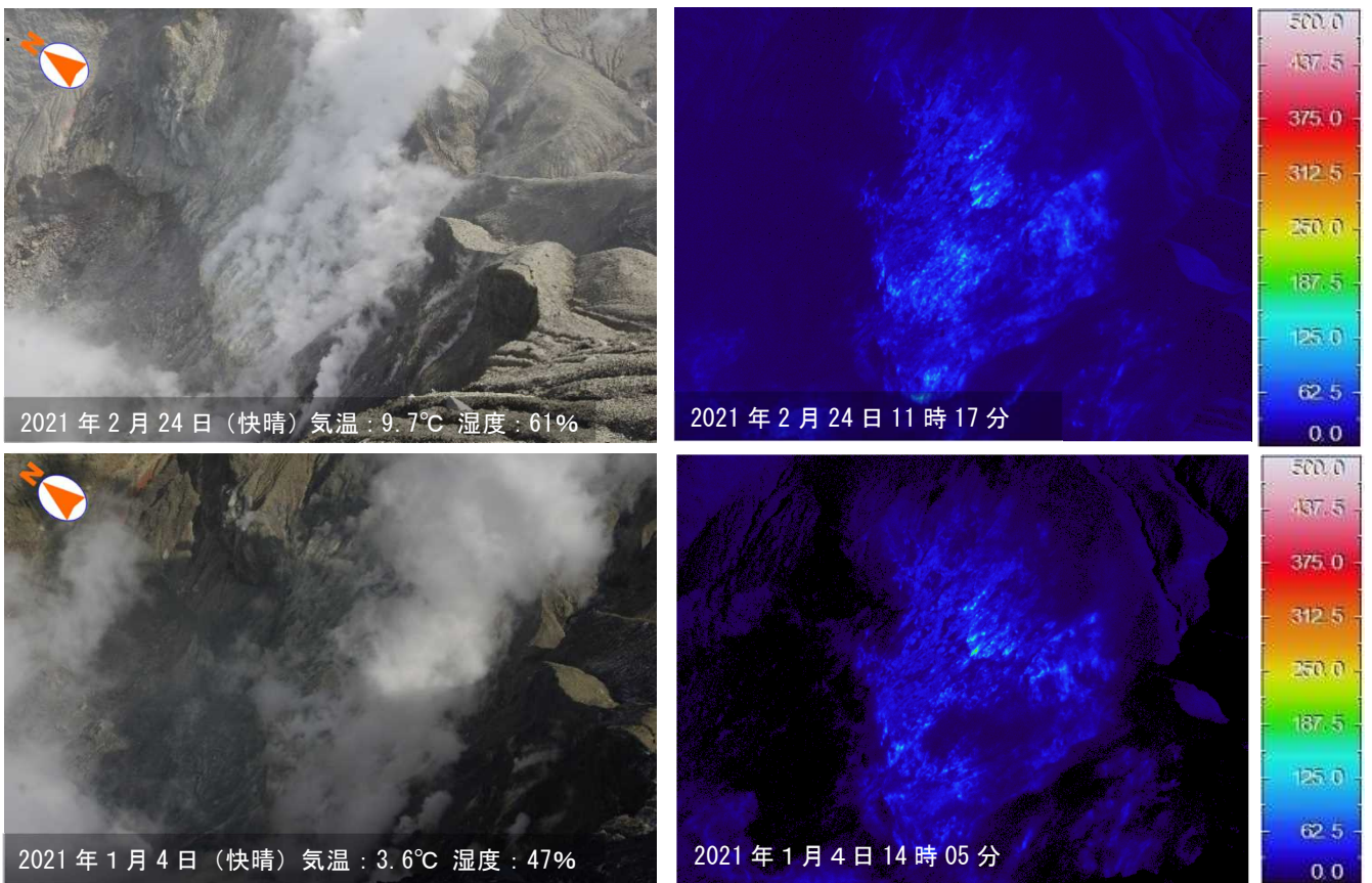
図6 阿蘇山 中岳第一火口内南側火口壁（火口南西側観測定点から観測）
