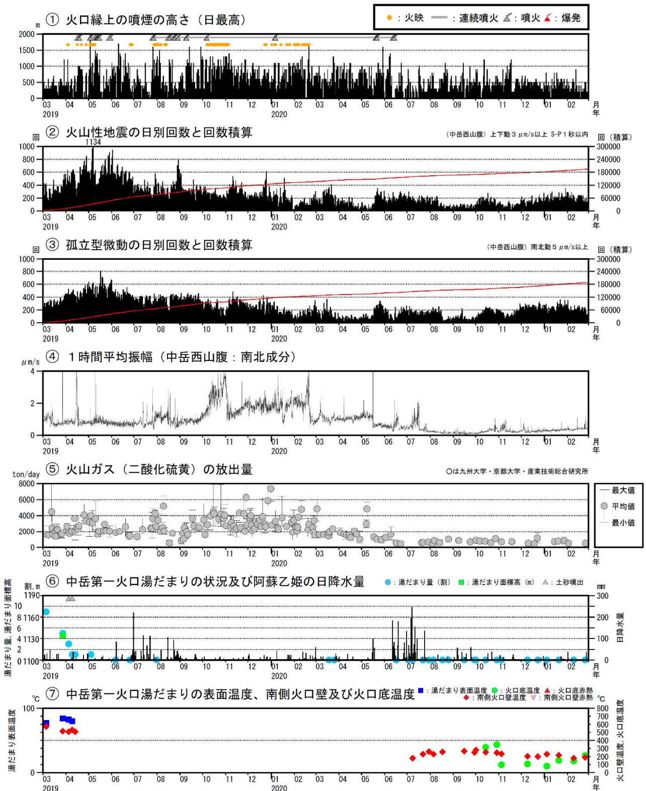
図7 阿蘇山 火山活動経過図（2019年2月～2021年2月）
