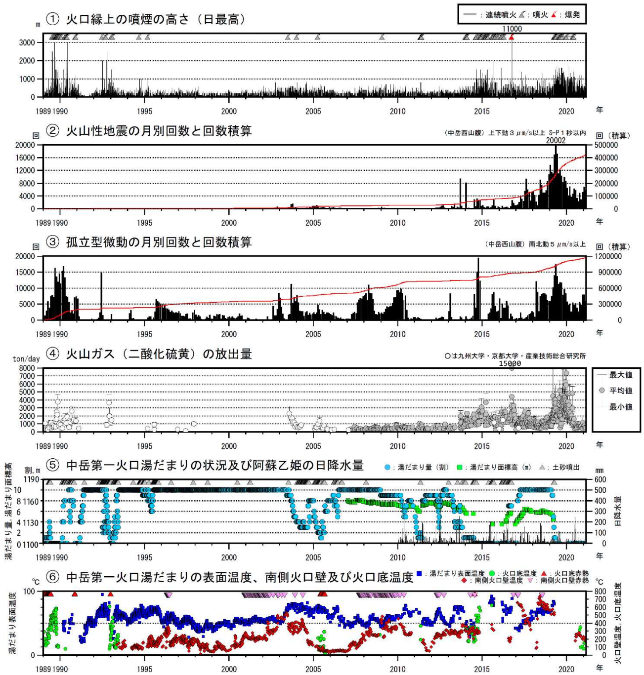
図8 阿蘇山 火山活動経過図（1989年1月～2021年2月）
