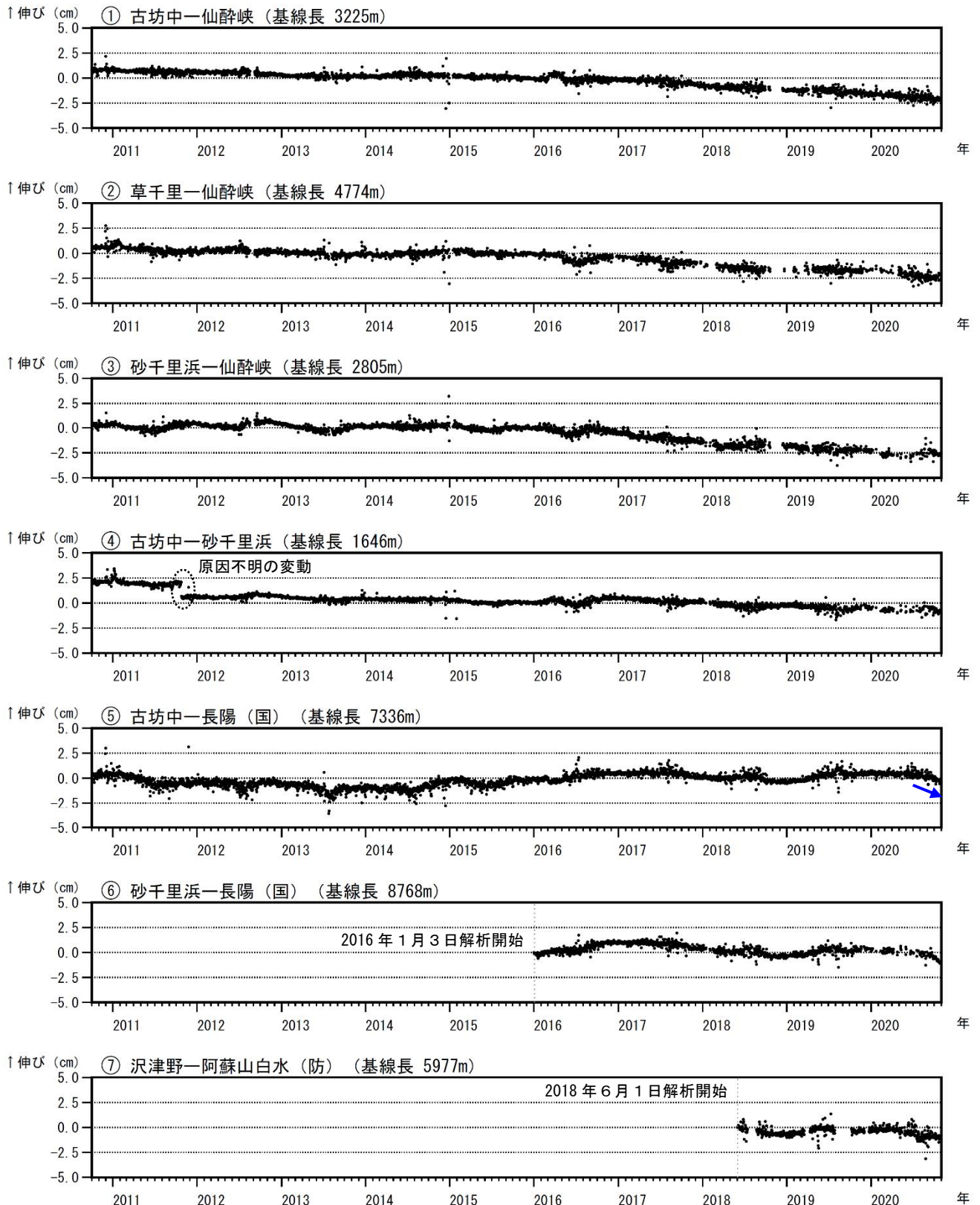
図12 阿蘇山 GNSS 観測による基線長変化（2010年10月～2020年10月）
