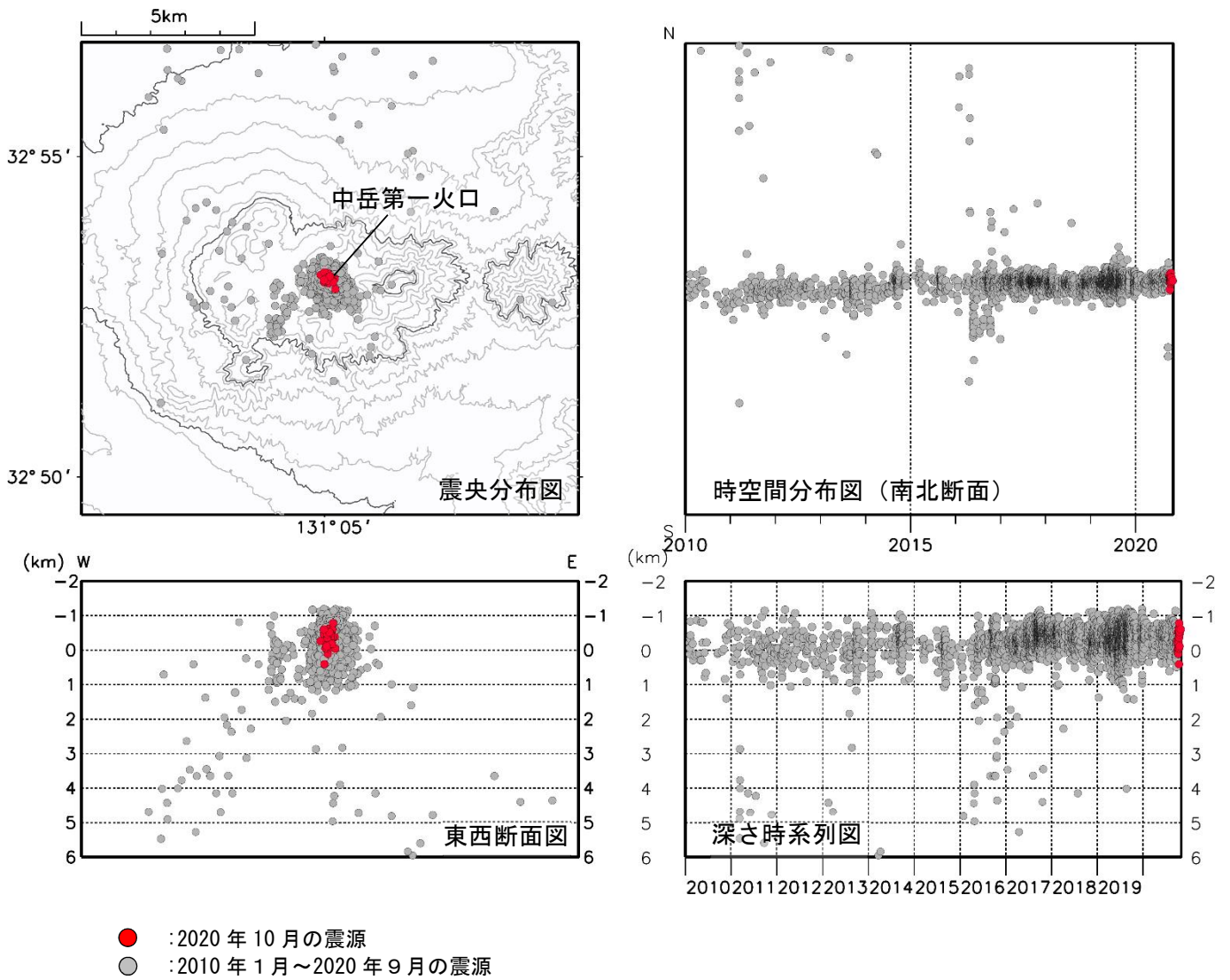
図11 阿蘇山 火山性地震の震源分布（2010年1月～2020年10月）
