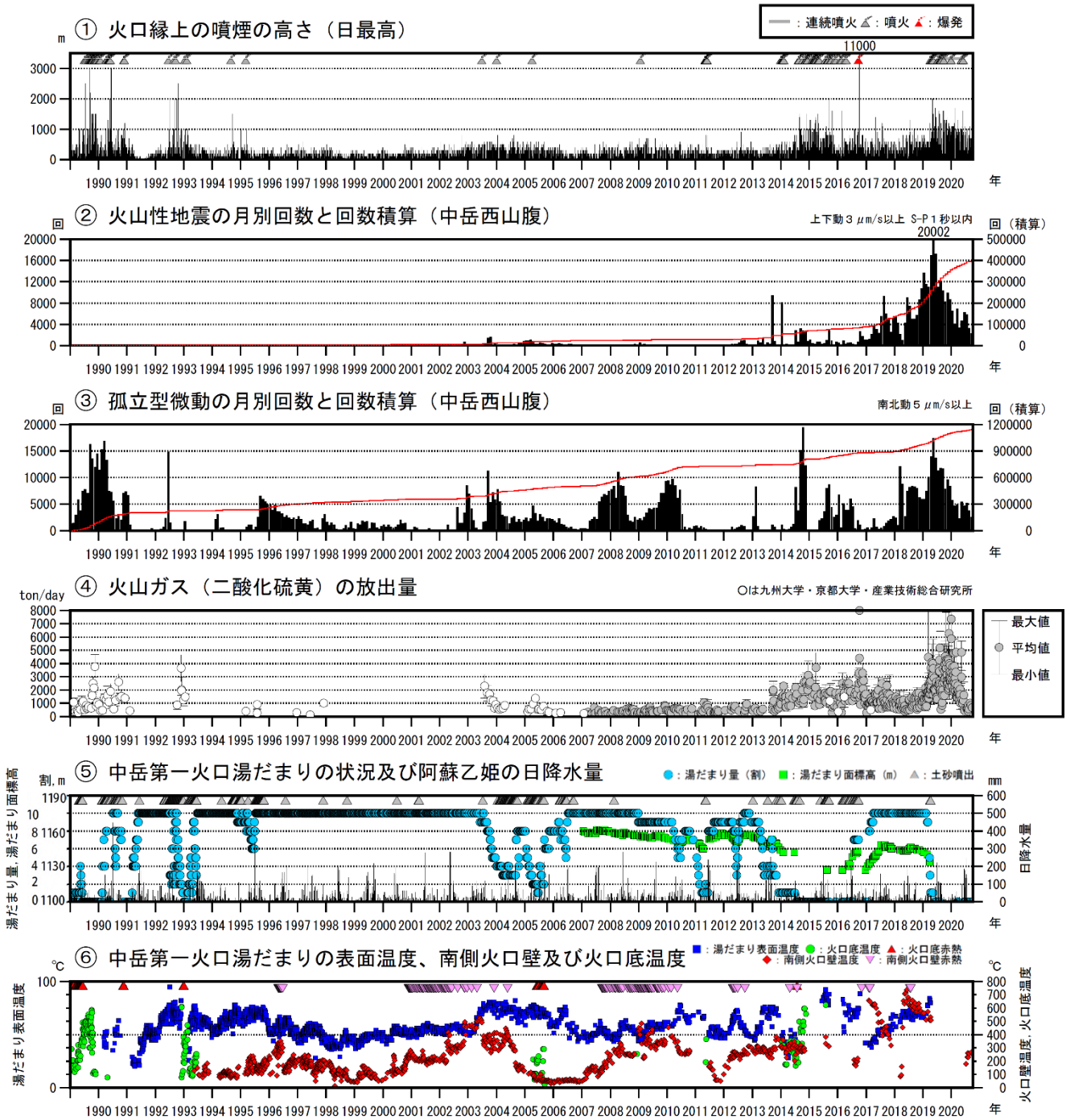
図8 阿蘇山 火山活動経過図（1989年1月～2020年9月）
