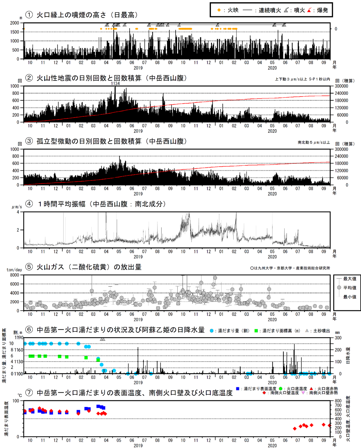
図7 阿蘇山 火山活動経過図（2018年9月～2020年9月）
