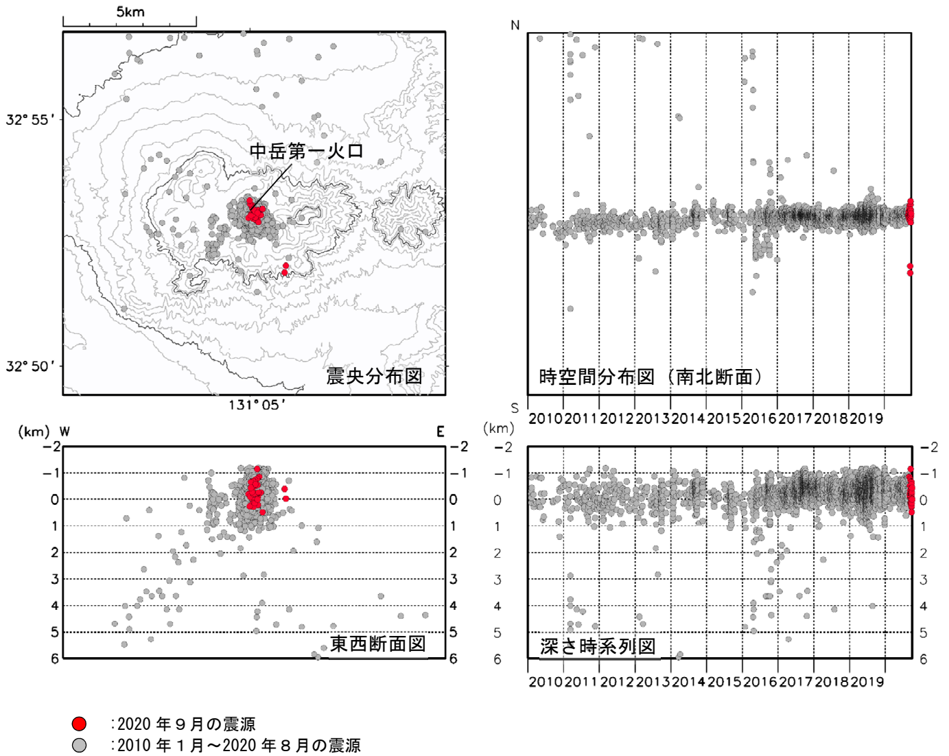
図10 阿蘇山 火山性地震の震源分布（2010年1月～2020年9月）
