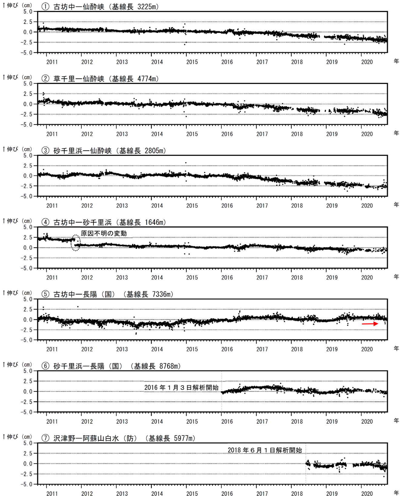
図 11 阿蘇山 GNSS 観測による基線長変化（2010年10月～2020年9月）
