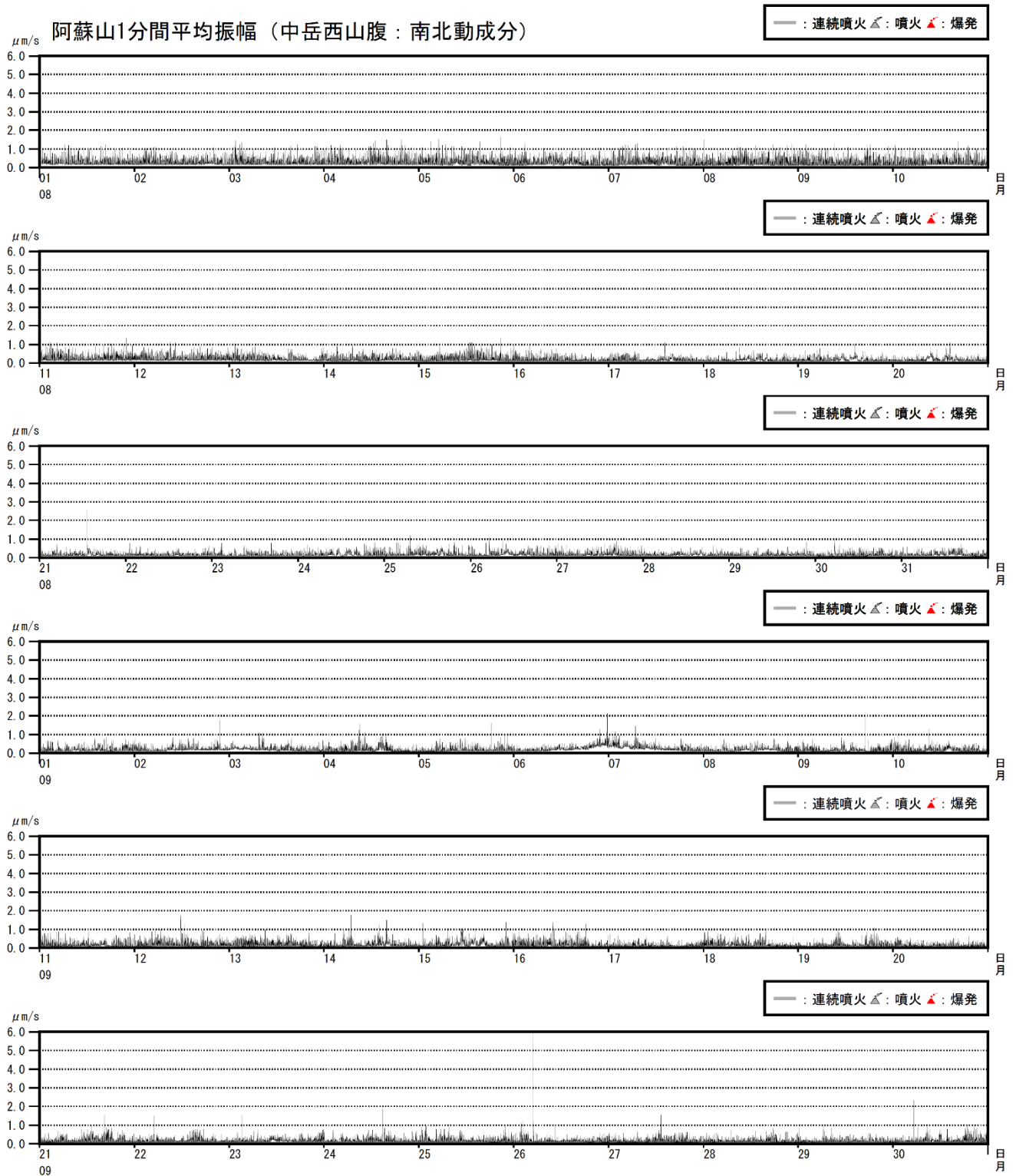
図9 阿蘇山 1分間平均振幅の時間変化（中岳西山腹観測点南北動成分、2020年8月～9月）
