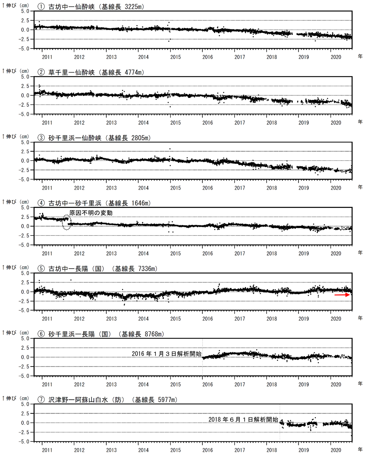
図 11 阿蘇山 GNSS 観測による基線長変化（2010年10月～2020年8月）
