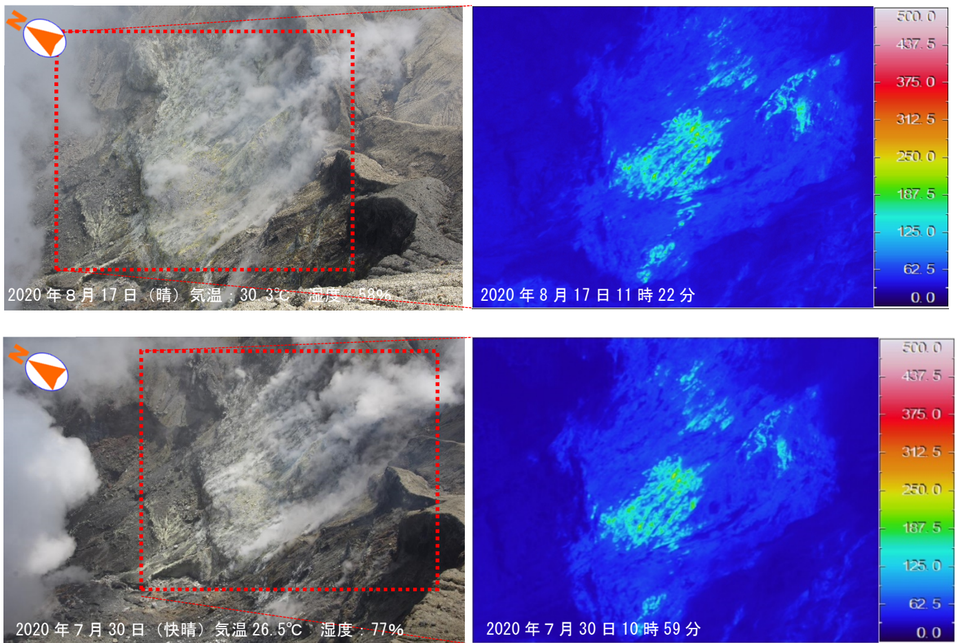
図6 阿蘇山 中岳第一火口内南側火口壁（中岳第一火口の南西側から観測）
