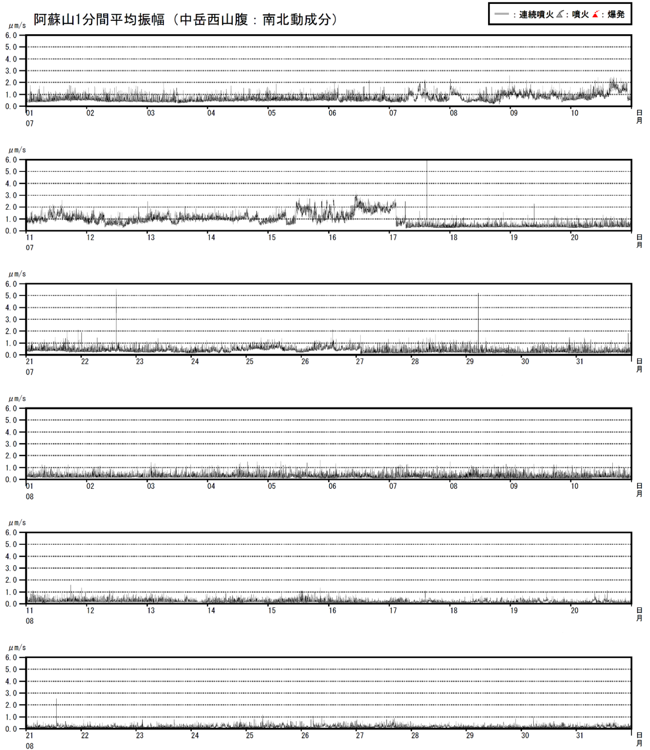
図9 阿蘇山 1分間平均振幅の時間変化（中岳西山腹観測点南北動成分、2020年7月～8月）
