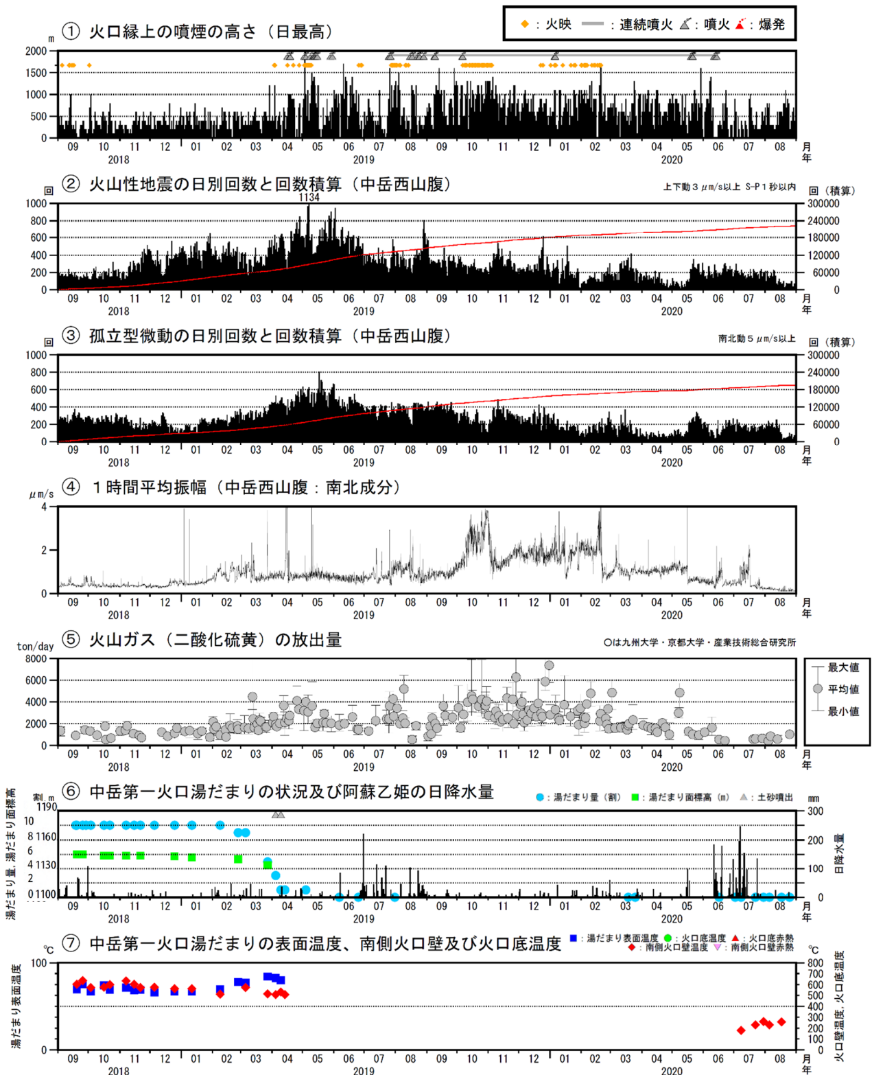
図7 阿蘇山 火山活動経過図（2018年9月～2020年8月）
