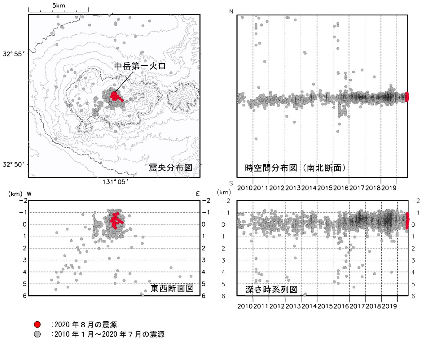
図10 阿蘇山 火山性地震の震源分布（2010年1月～2020年8月）
