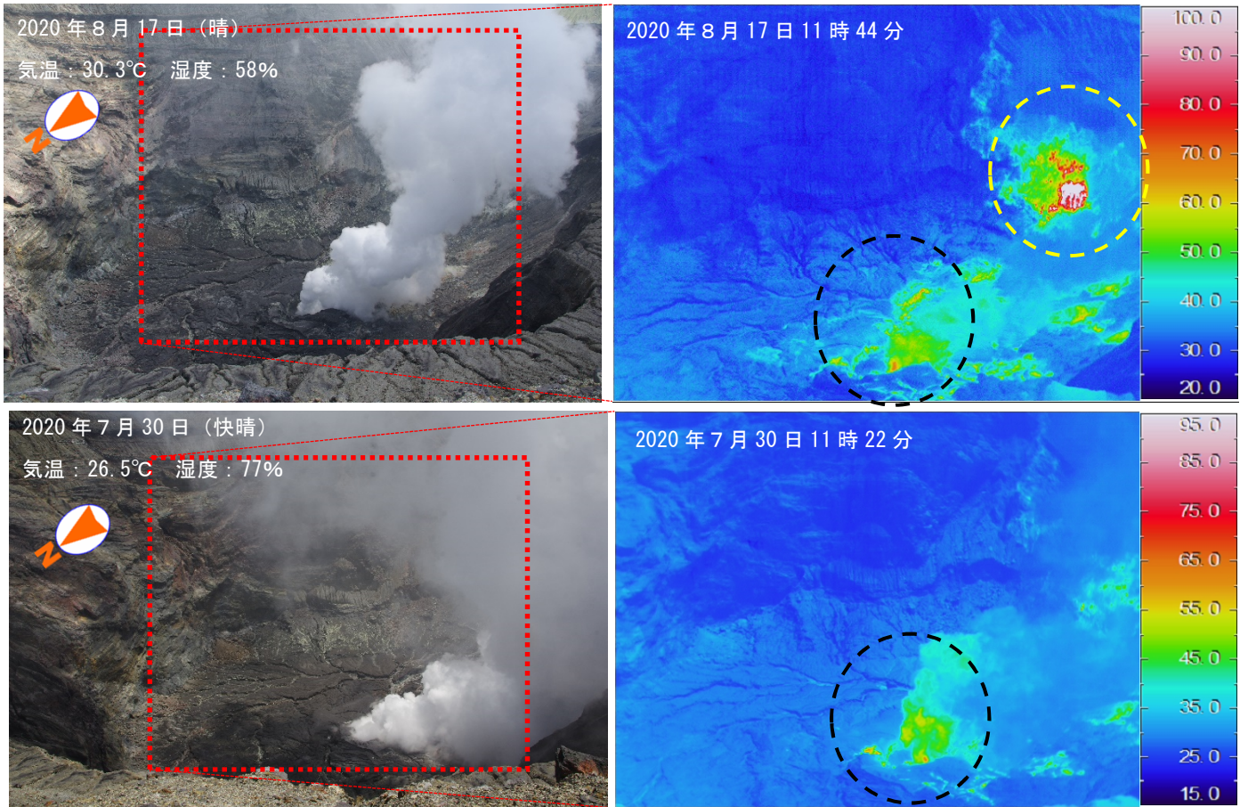
図5 阿蘇山 中岳第一火口内の状況（中岳第一火口の北西側から観測）
