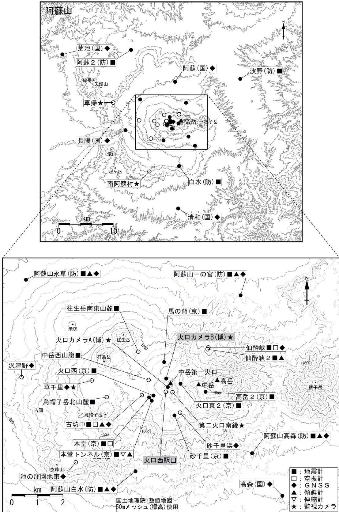
図13 阿蘇山 観測点配置図
