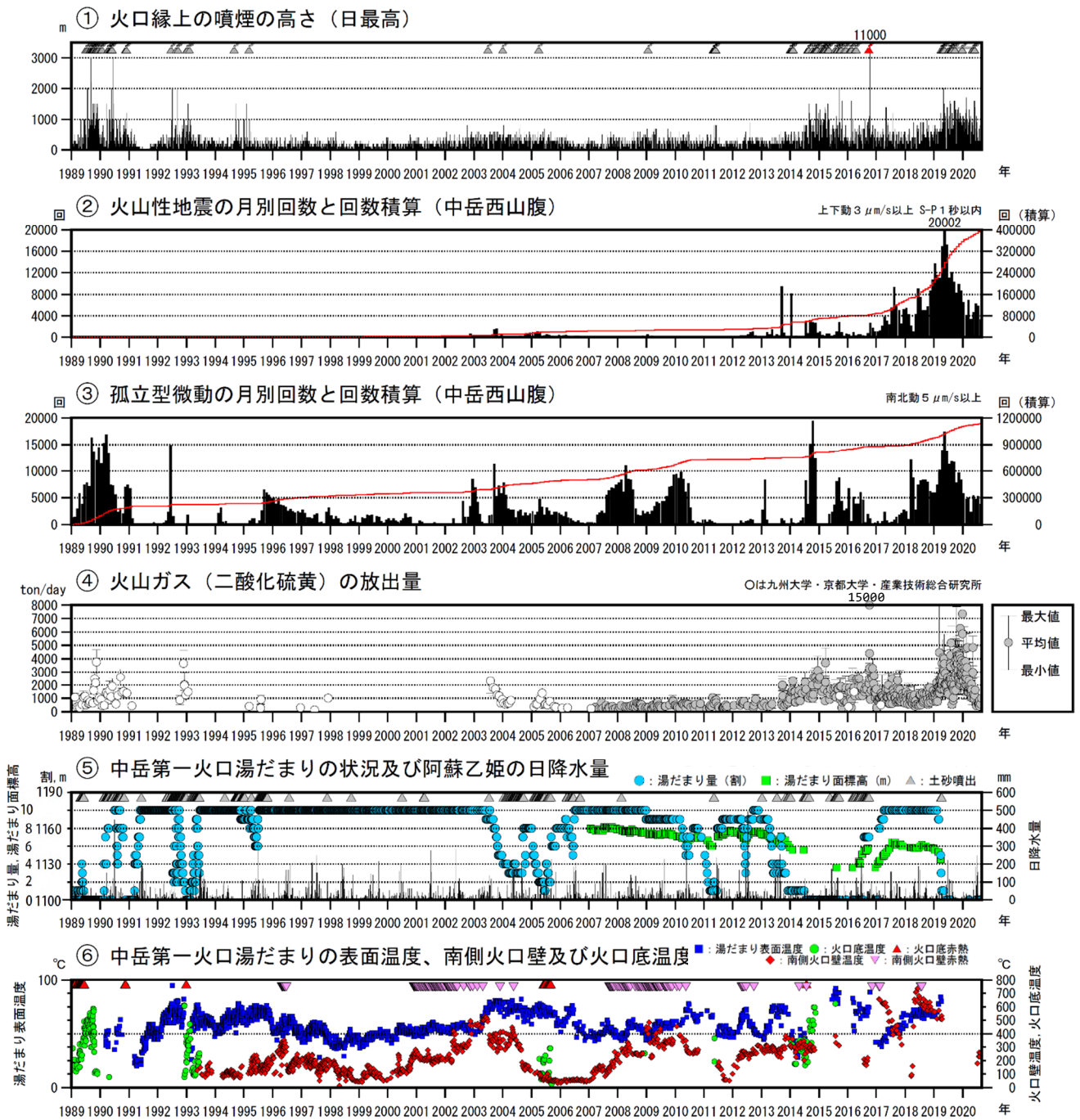
図8 阿蘇山 火山活動経過図（1989年1月～2020年8月）
