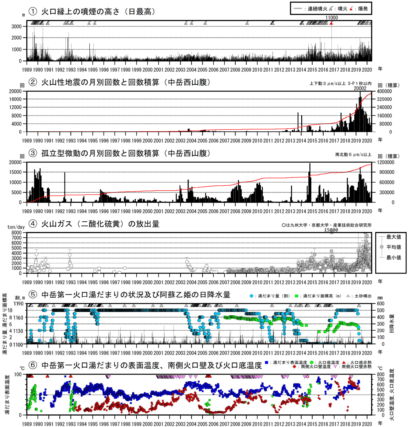
図4 阿蘇山 火山活動経過図（1989年1月～2020年5月）
