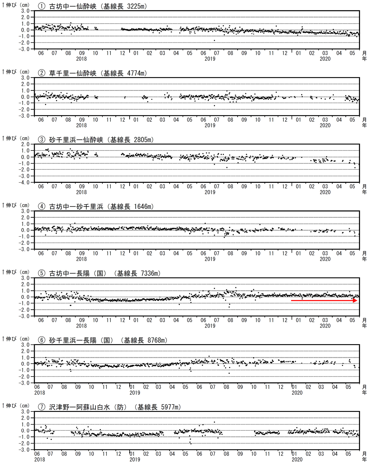
図 7-2 阿蘇山 GNSS 観測による基線長変化（2018年6月～2020年5月）
