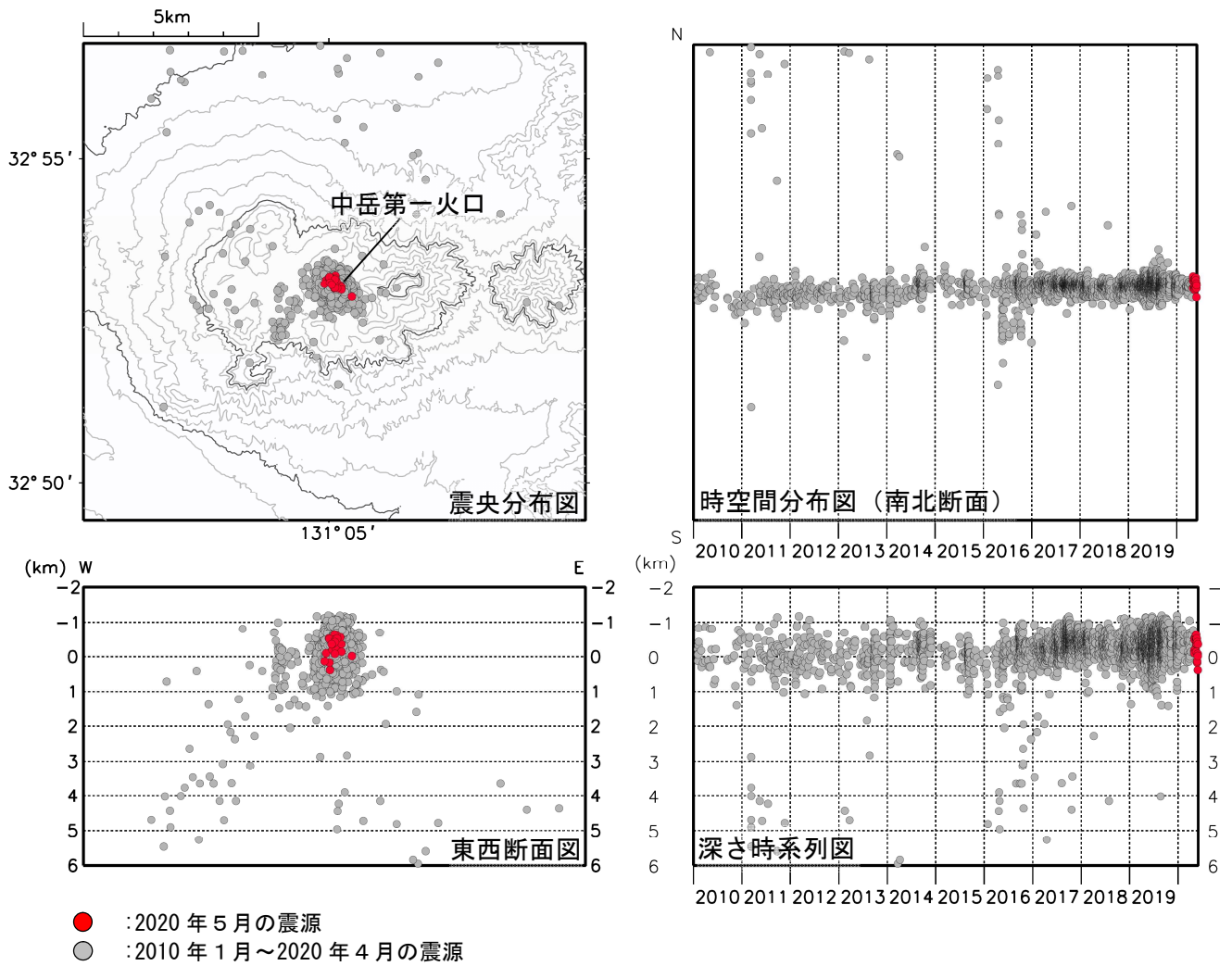
図6 阿蘇山 火山性地震の震源分布（2010年1月～2020年5月）
