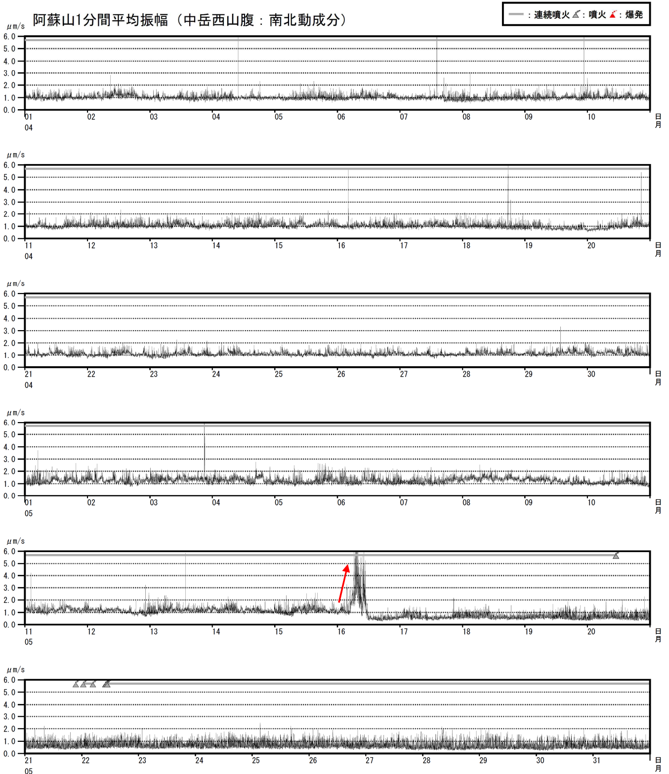
図5 阿蘇山 1分間平均振幅の時間変化（中岳西山腹観測点南北動成分、2020年4月～5月）
