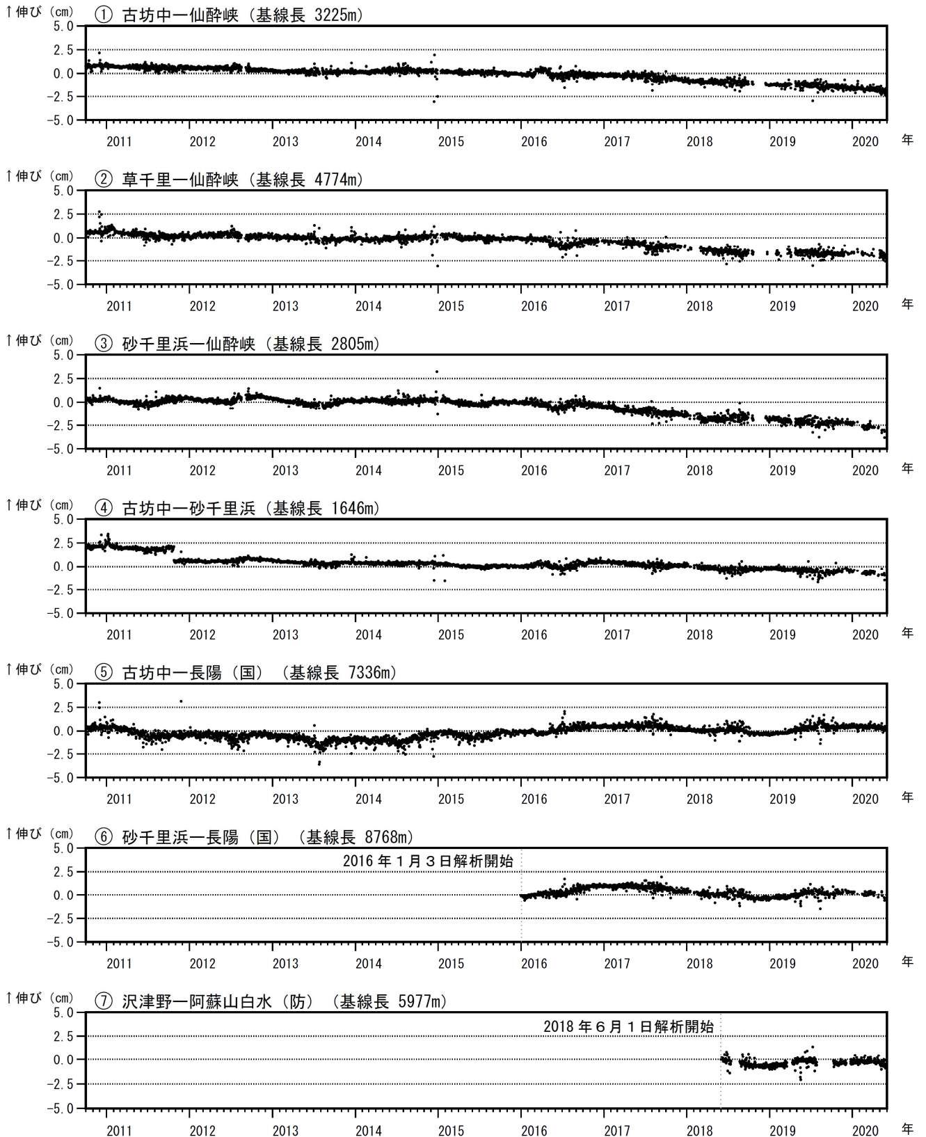
図7-1 阿蘇山 GNSS 観測による基線長変化（2010年10月～2020年5月）
