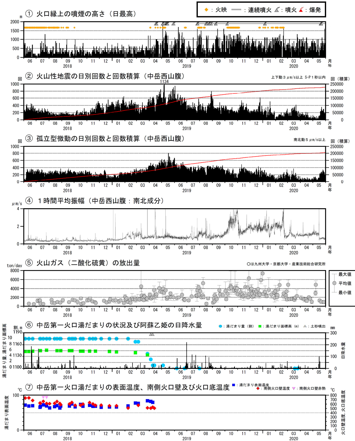
図3 阿蘇山 火山活動経過図（2018年6月～2020年5月）
