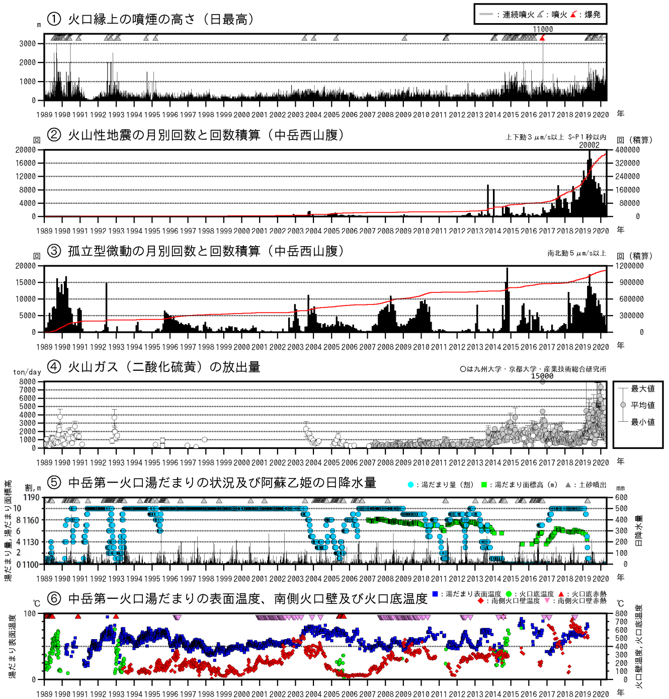
図4 阿蘇山 火山活動経過図（1989年1月～2020年4月）
