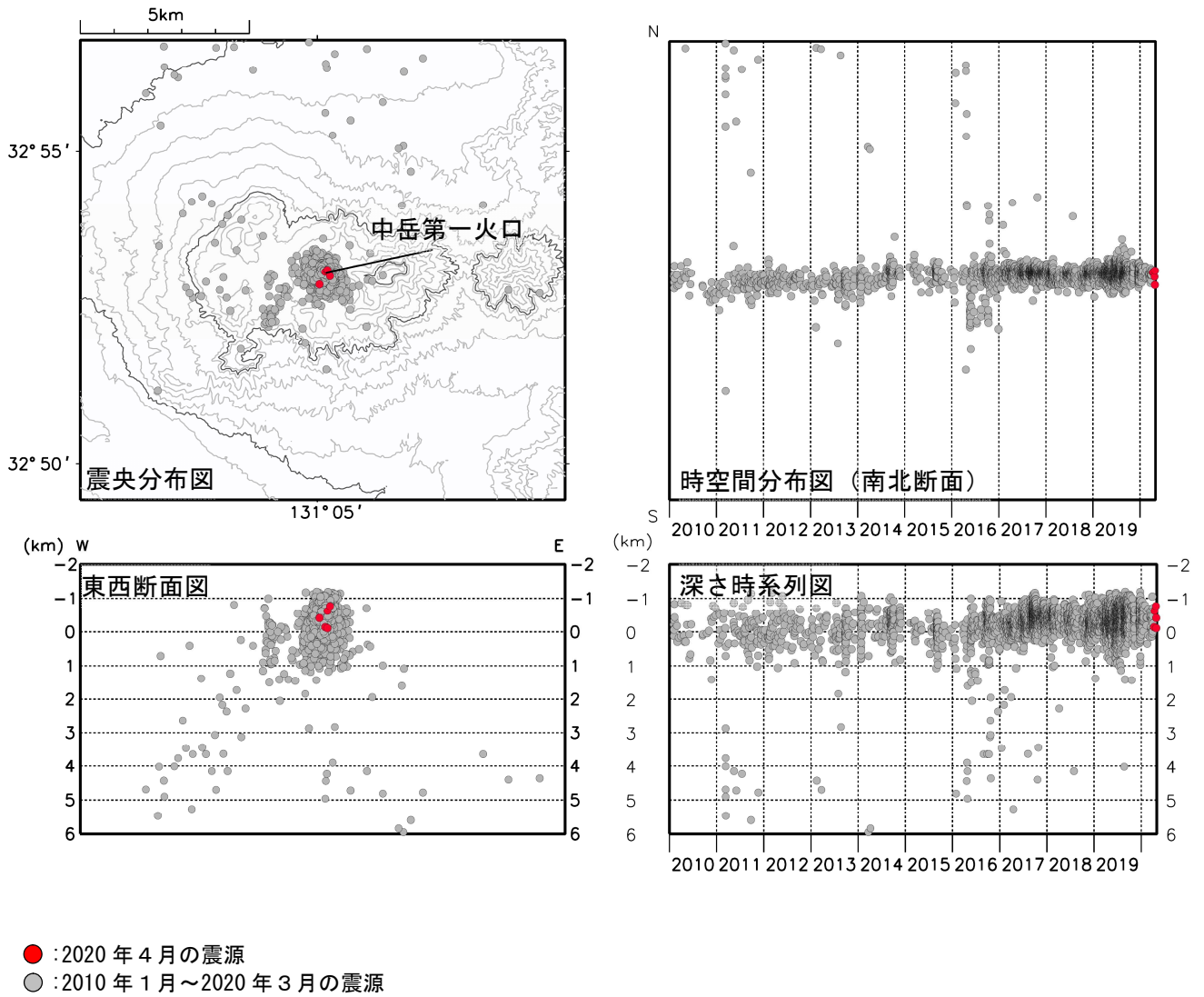
図6 阿蘇山 火山性地震の震源分布（2010年1月～2020年4月）
