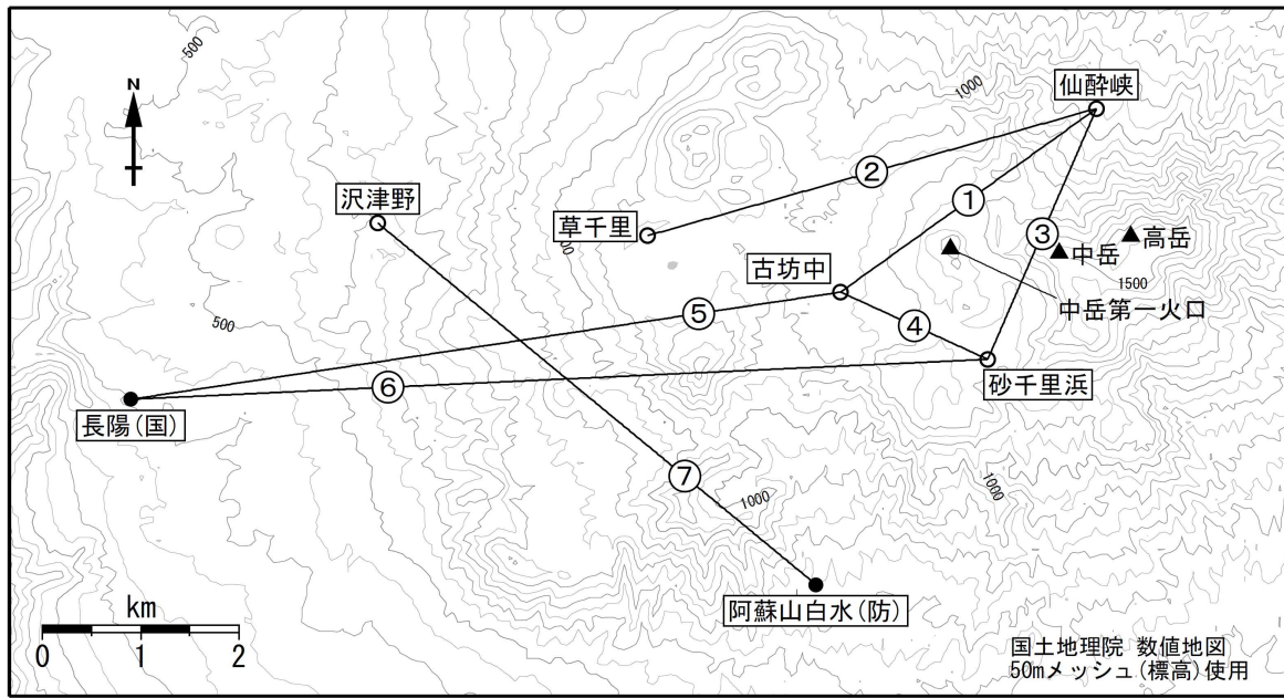
図8 阿蘇山 GNSS 連続観測点と基線番号
