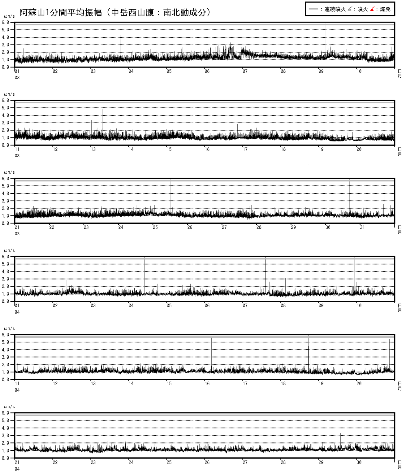
図5 阿蘇山 1分間平均振幅の時間変化（中岳西山腹観測点南北動成分、2020年3月～4月）
