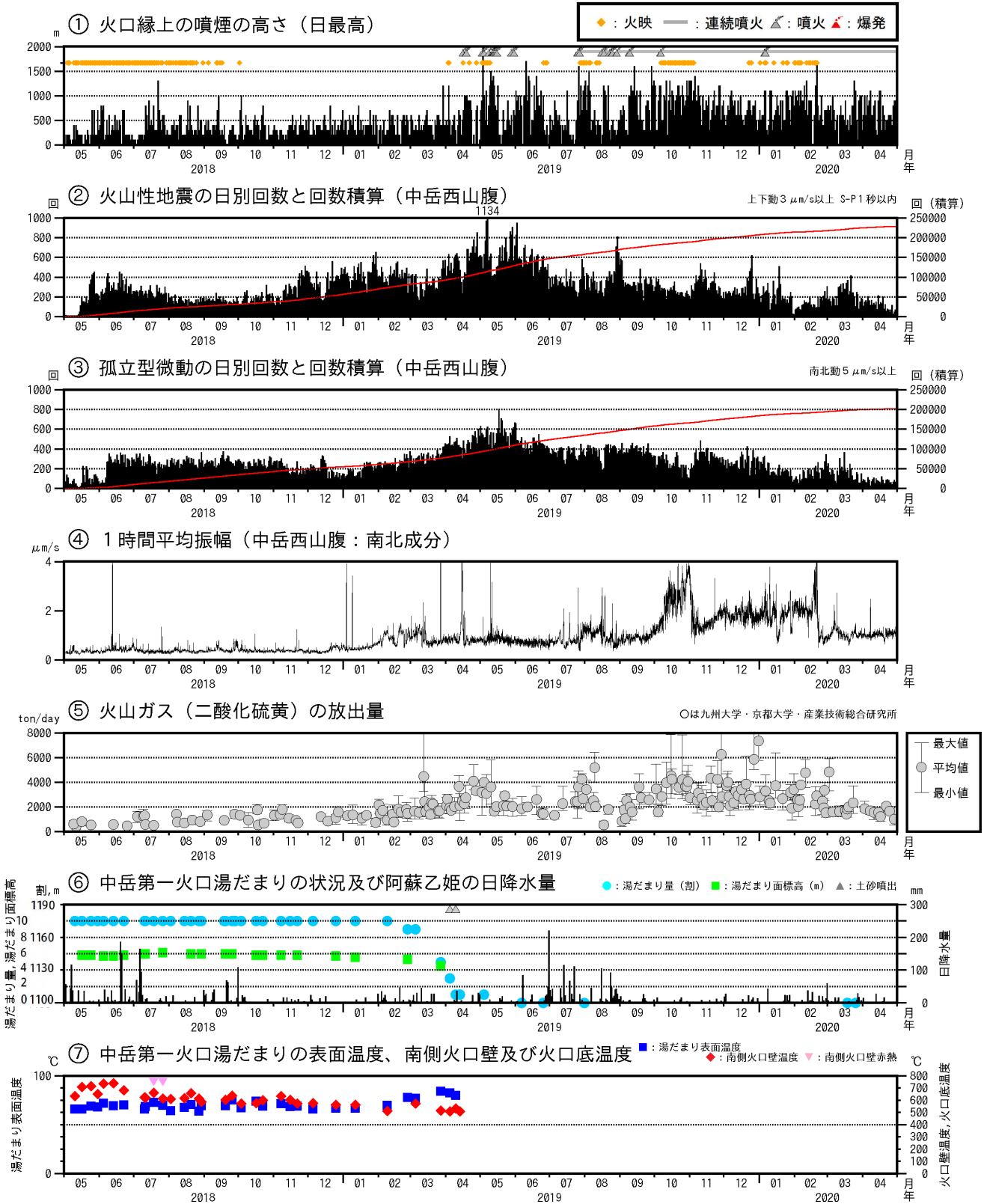
図3 阿蘇山 火山活動経過図（2018年5月～2020年4月）
