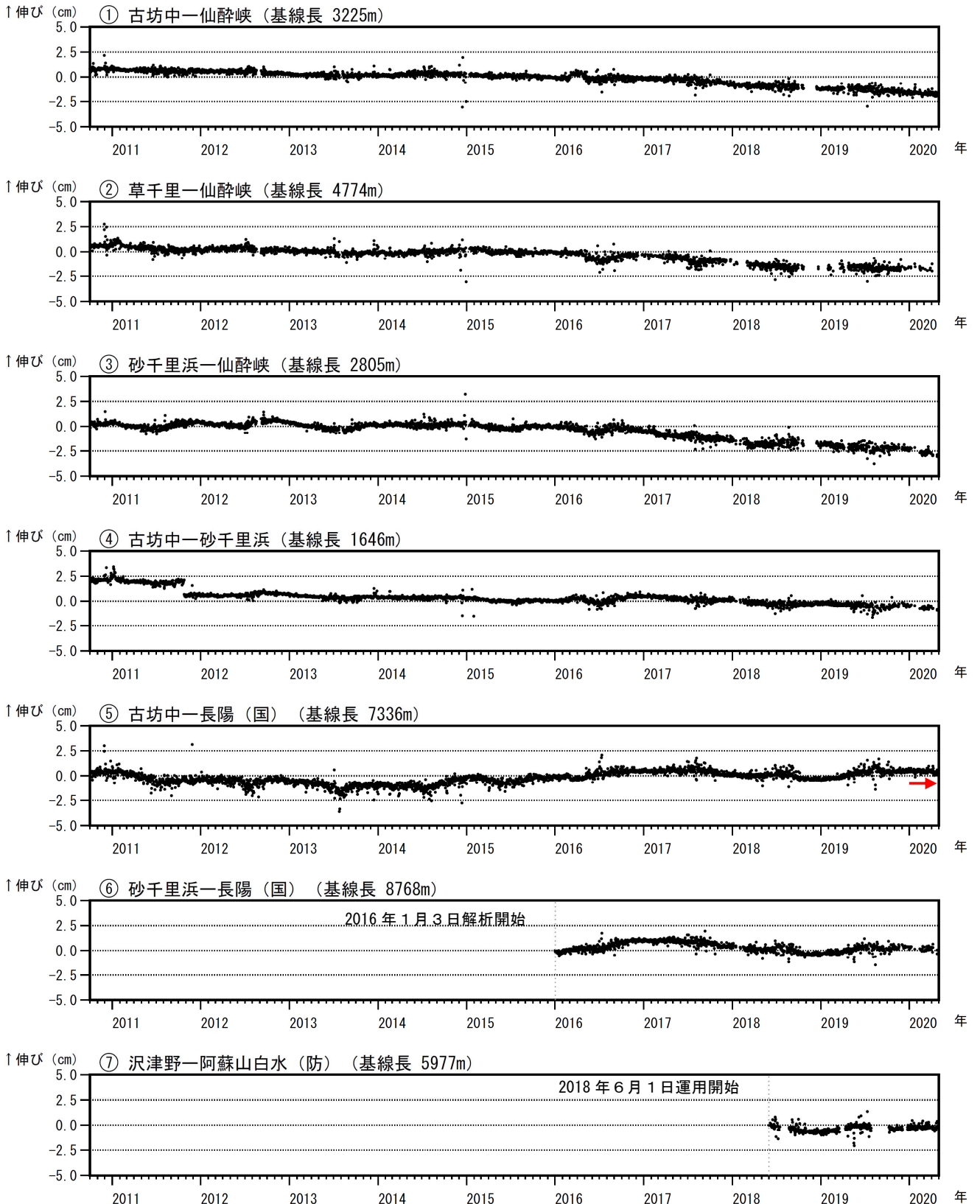
図7 阿蘇山 GNSS 観測による基線長変化（2010年10月～2020年4月）
