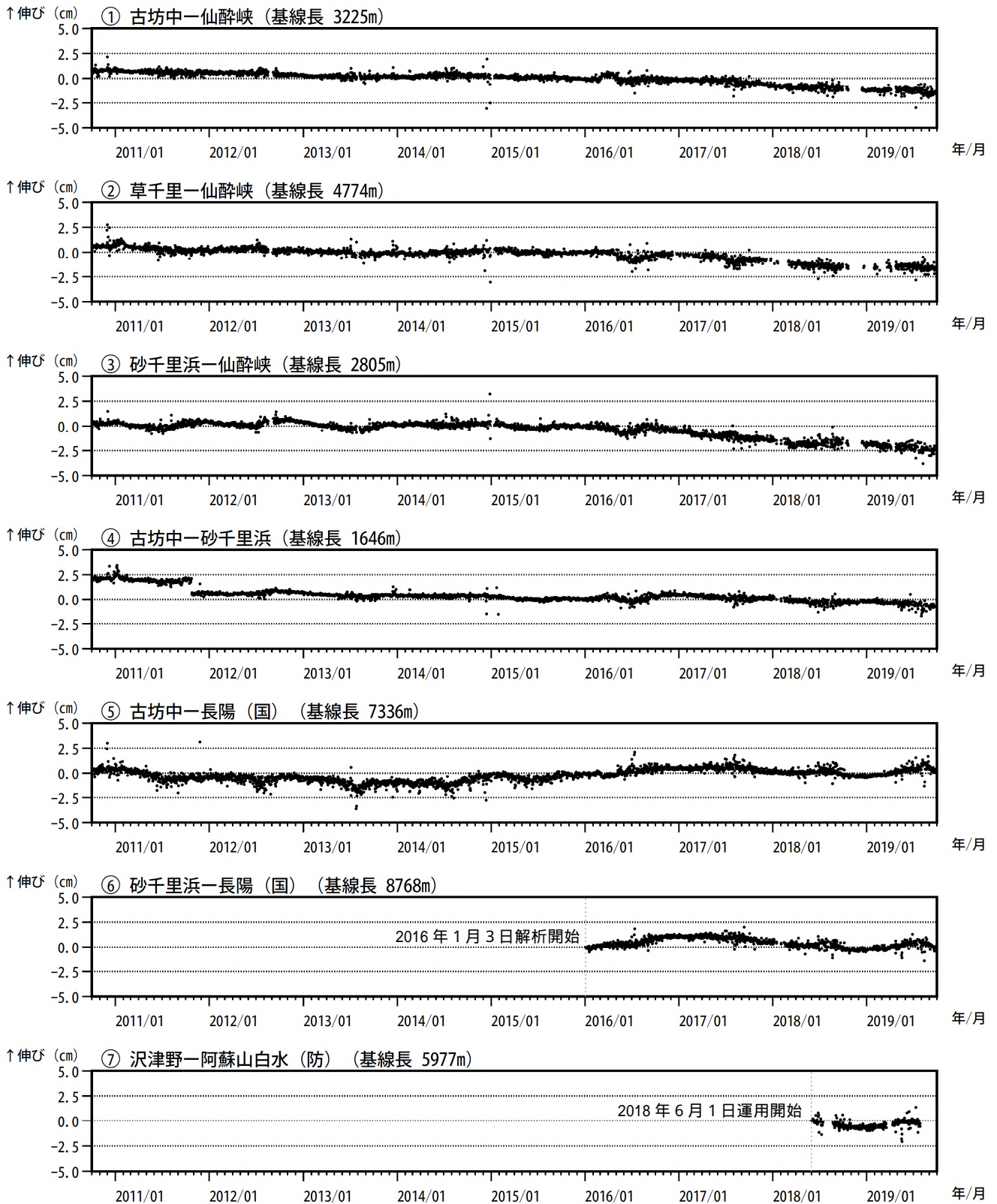
図10 阿蘇山 GNSS 観測による基線長変化（2010年10月～2019年9月）
