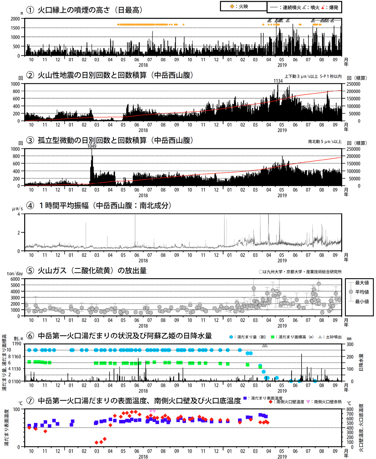
図4 阿蘇山 火山活動経過図（2017年10月～2019年9月）
