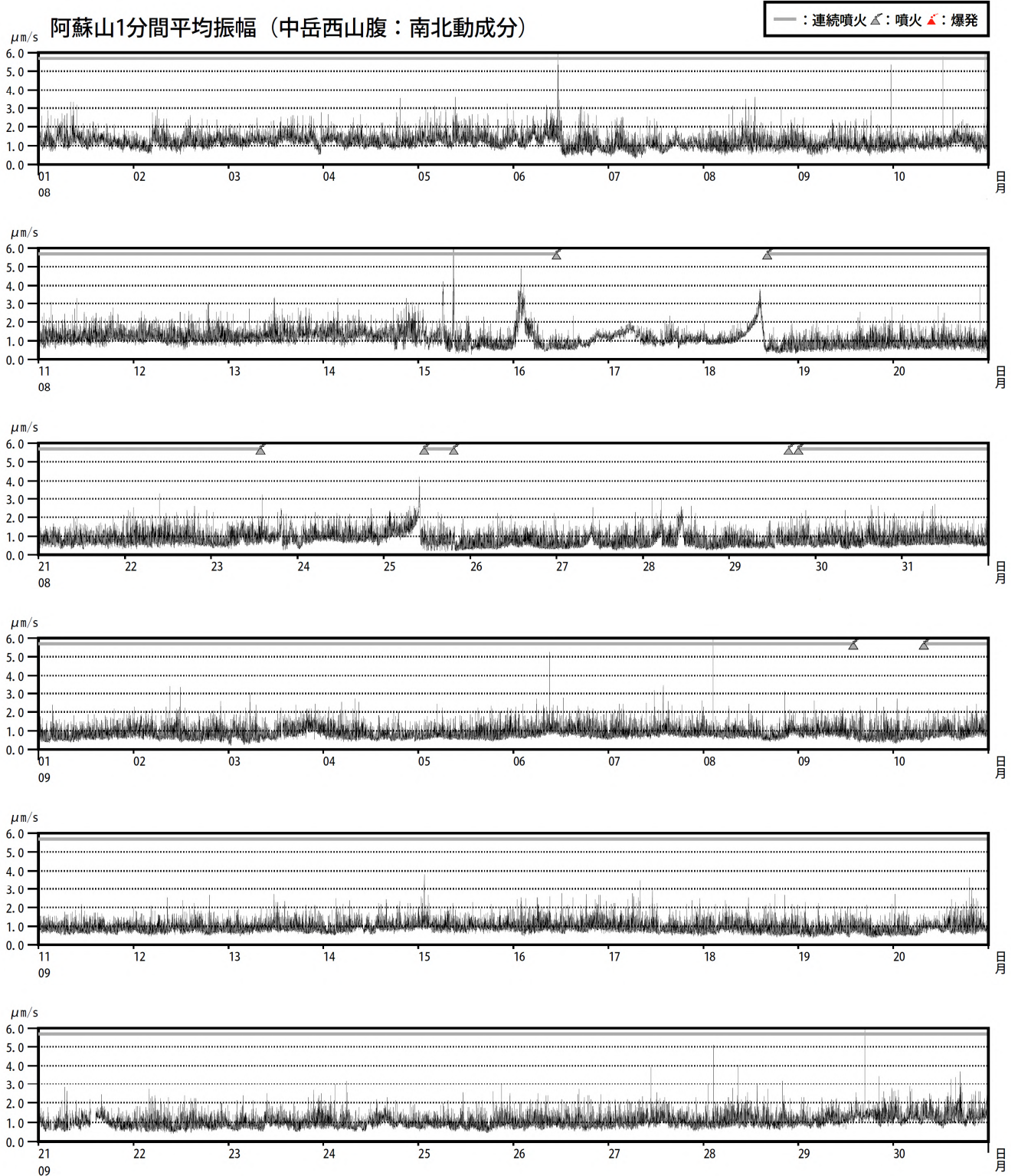
図6 阿蘇山 1分間平均振幅の時間変化（中岳西山腹観測点南北動成分、2019年8月～9月）
