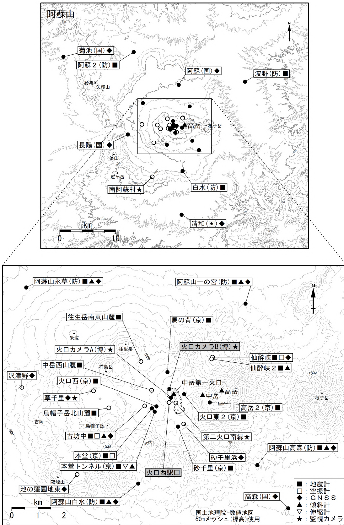
図11 阿蘇山 観測点配置図
