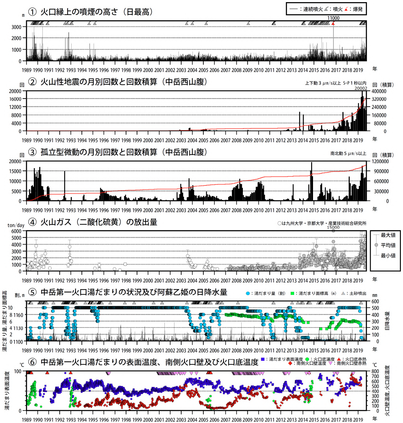
図5 阿蘇山 火山活動経過図（1989年1月～2019年9月）
