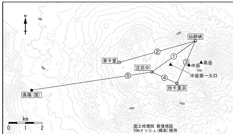
図13 阿蘇山 GNSS 連続観測点と基線番号
