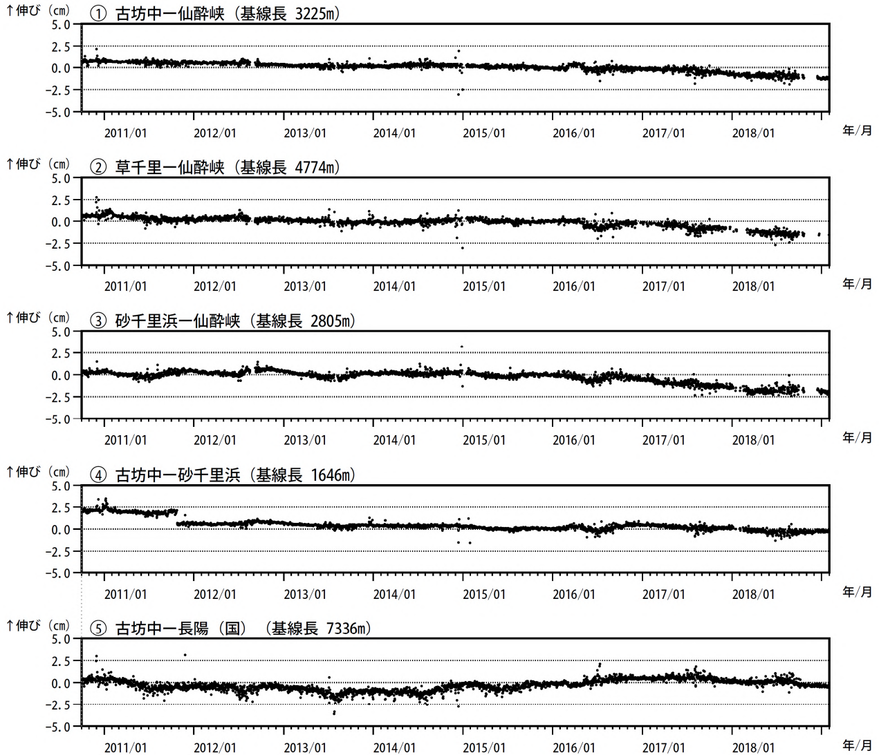
図12 阿蘇山 GNSS 観測による基線長変化(2010年10月~2019年1月)
