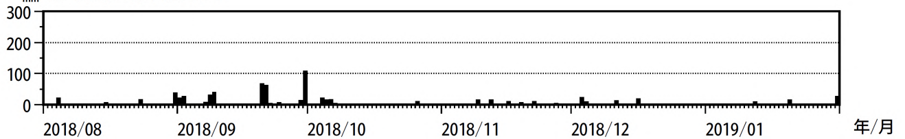
図 11 阿蘇山 古坊中観測点の傾斜変動及び阿蘇乙姫地域気象観測所の日降水量 (2018年8月~2019年1月)
