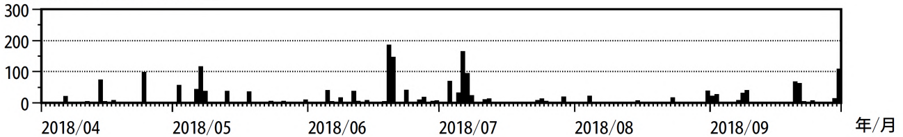
図 12 阿蘇山 古坊中観測点の傾斜変動及び阿蘇乙姫地域気象観測所の日降水量 (2018年4月～2018年9月)
