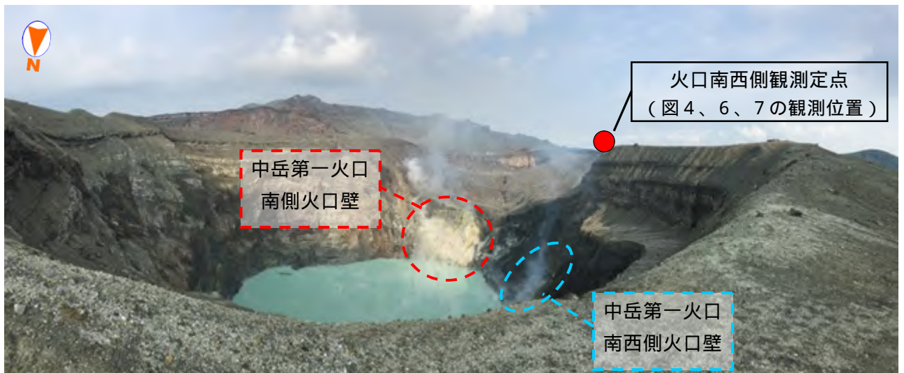
図3 阿蘇山 中岳第一火口北側観測定点からの火口全景
