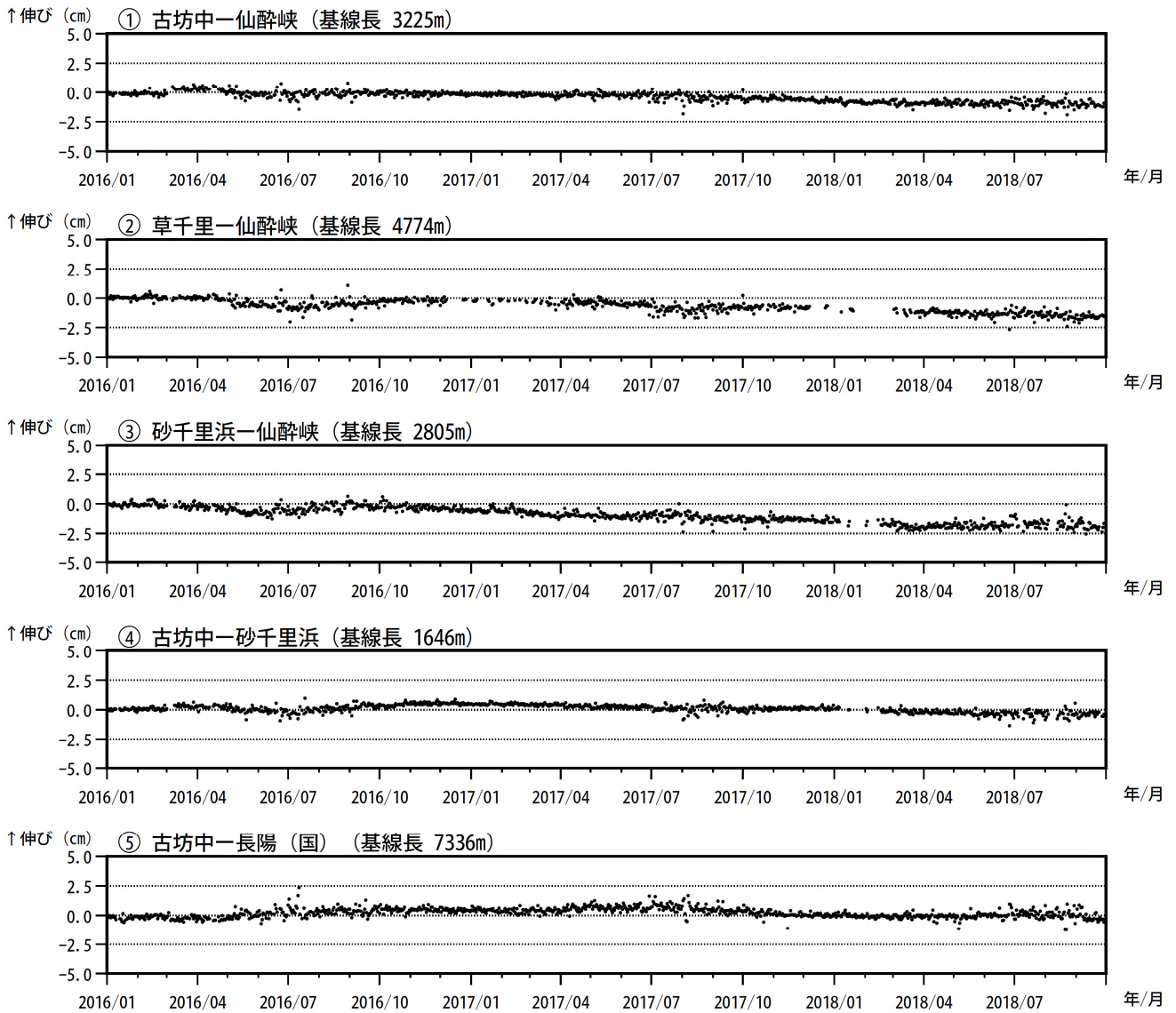
図 13-2 阿蘇山 GNSS 観測による短期の基線長変化（2016 年 1 月～2018 年 9 月）
