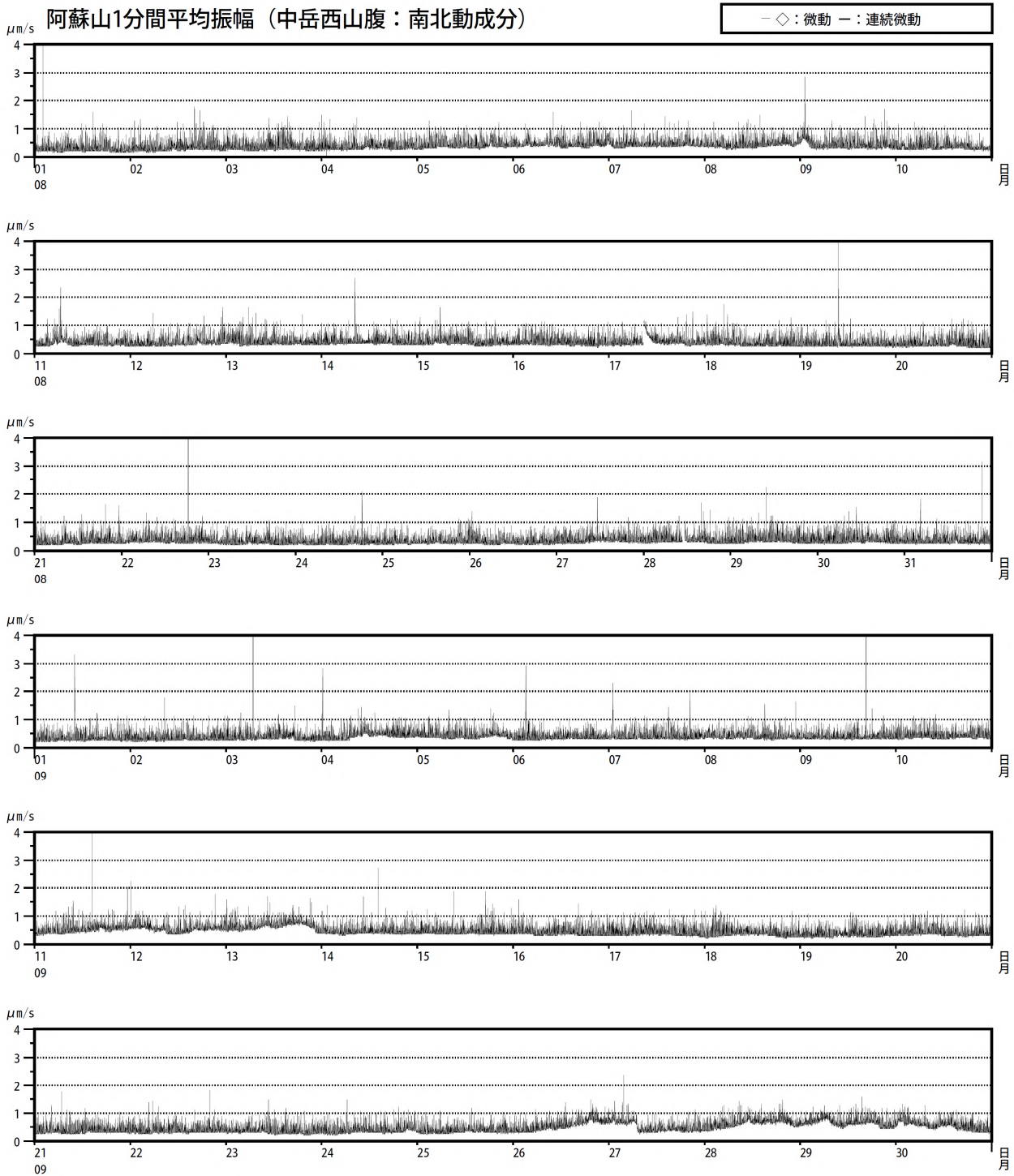
図11 阿蘇山 1分間平均振幅の時間変化（中岳西山腹観測点南北動成分、2018年8月～9月）
