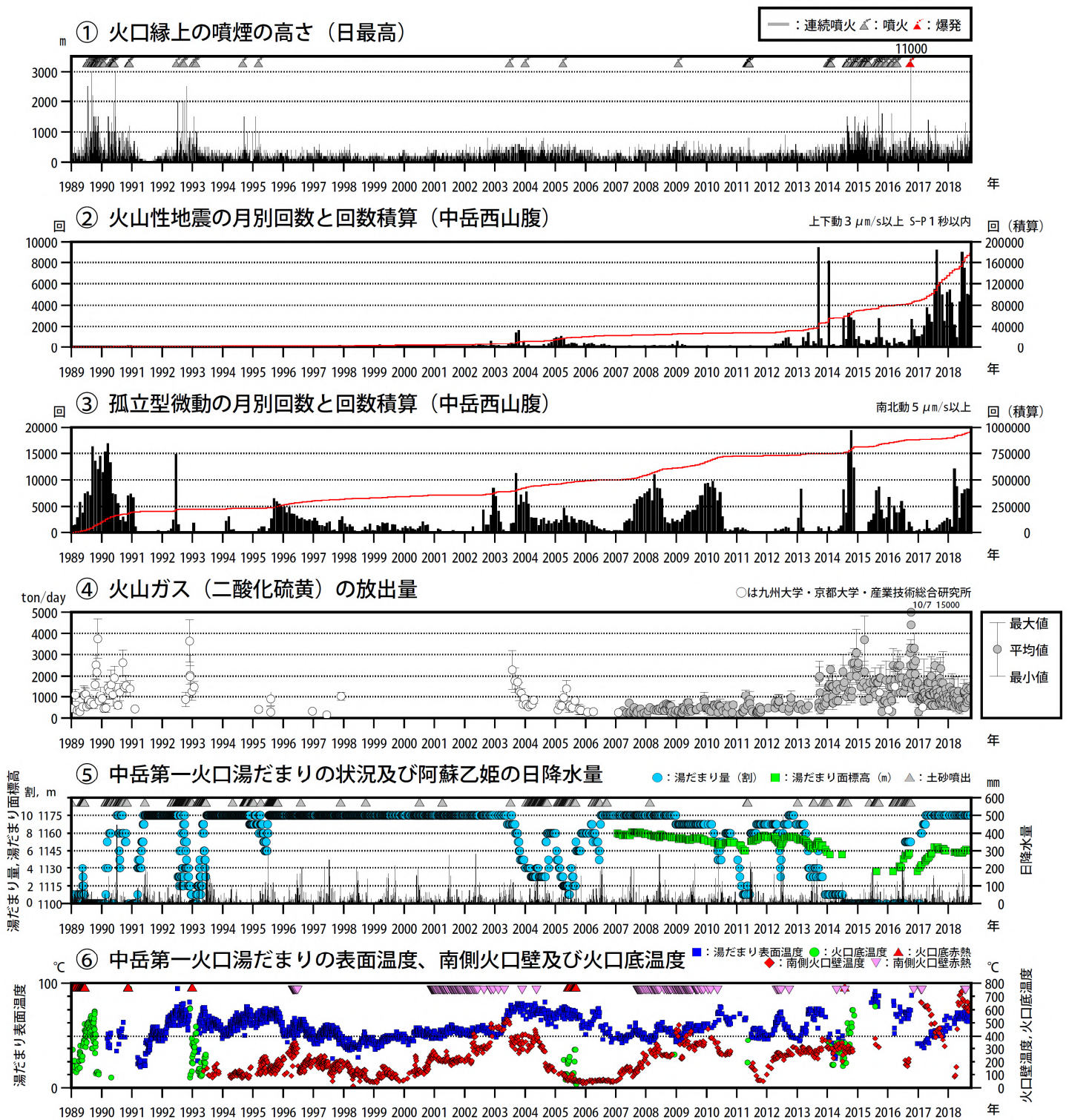
図 9 阿蘇山 火山活動経過図（1989 年 1 月～2018 年 9 月）
