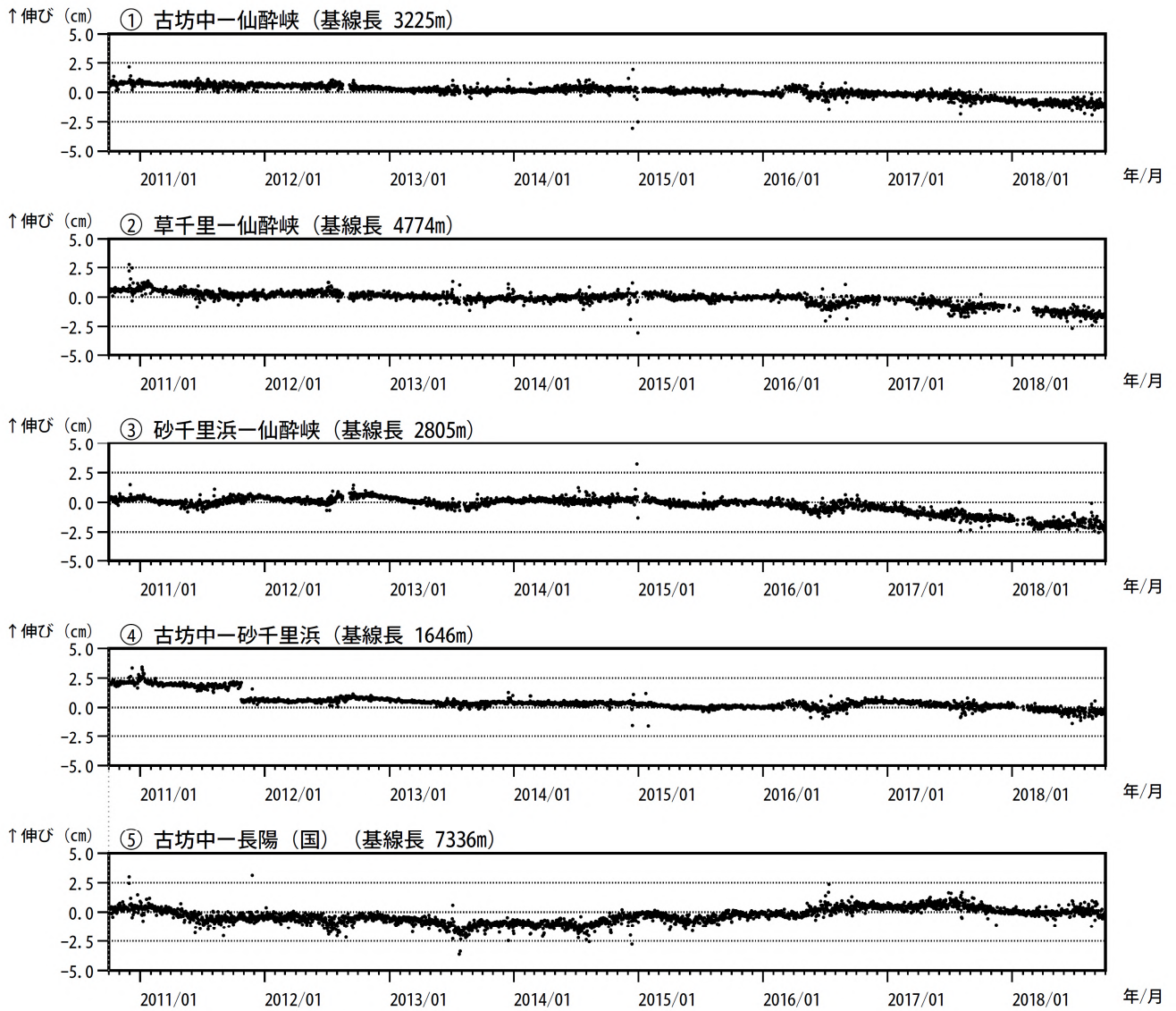
図 13-1 阿蘇山 GNSS連続観測による長期の基線長変化（2010 年 10 月～2018 年 9 月）
