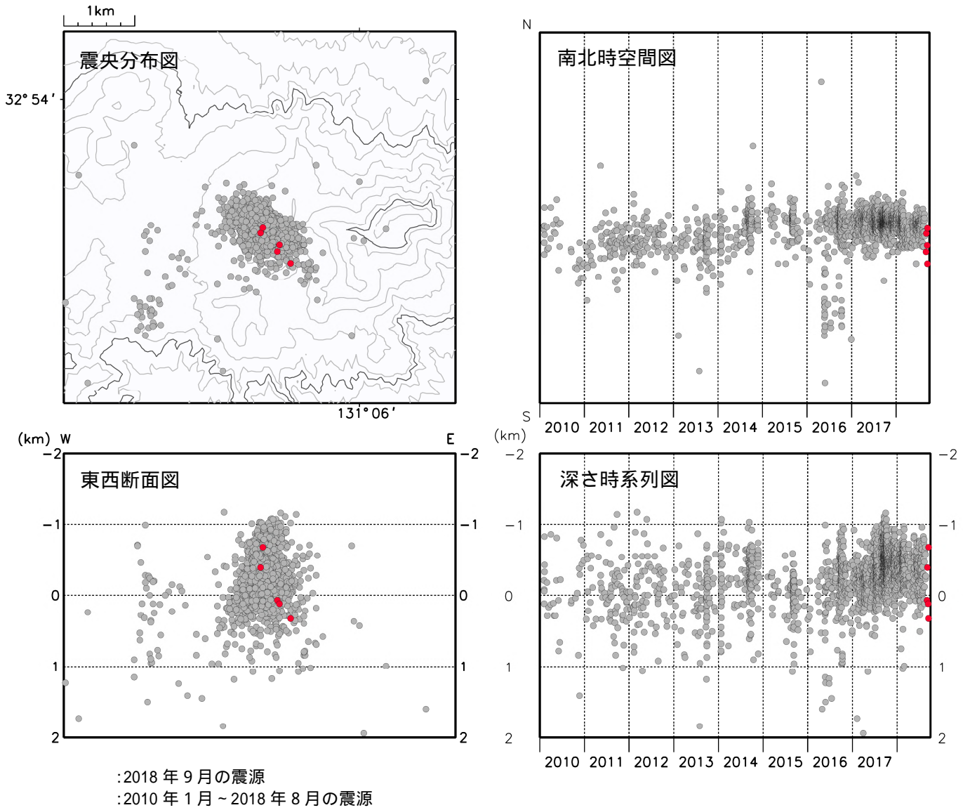
図 10 阿蘇山 火山性地震の震源分布（2010 年 1 月～2018 年 9 月）
