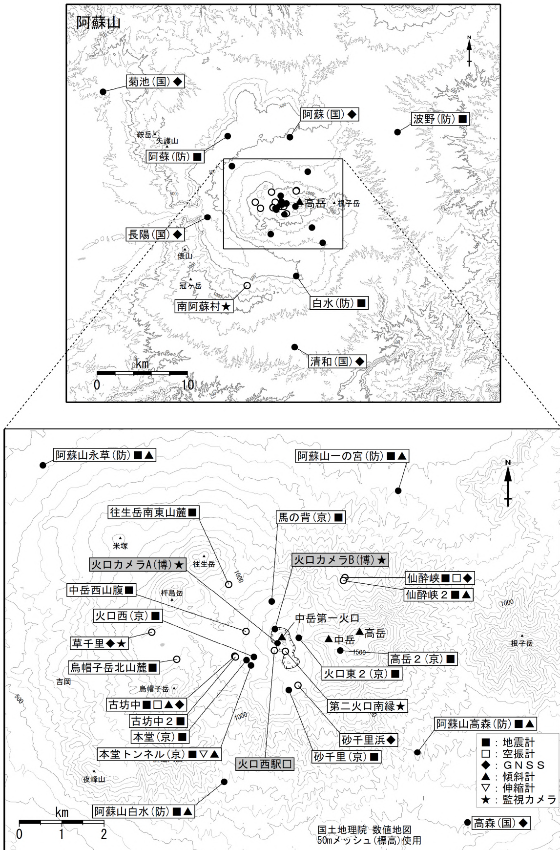
図15 阿蘇山 観測点配置図
