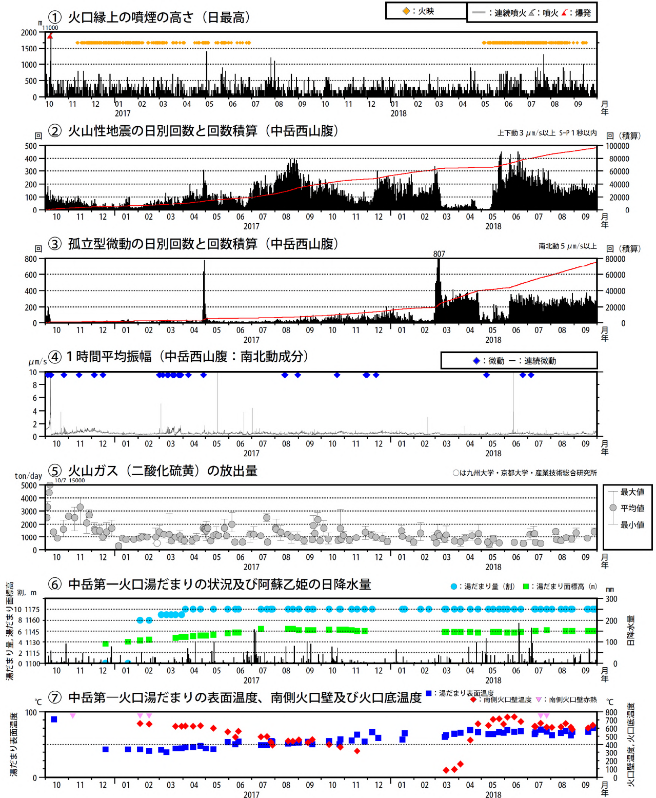
図 8 阿蘇山 火山活動経過図（2016 年 10 月～2018 年 9 月）
