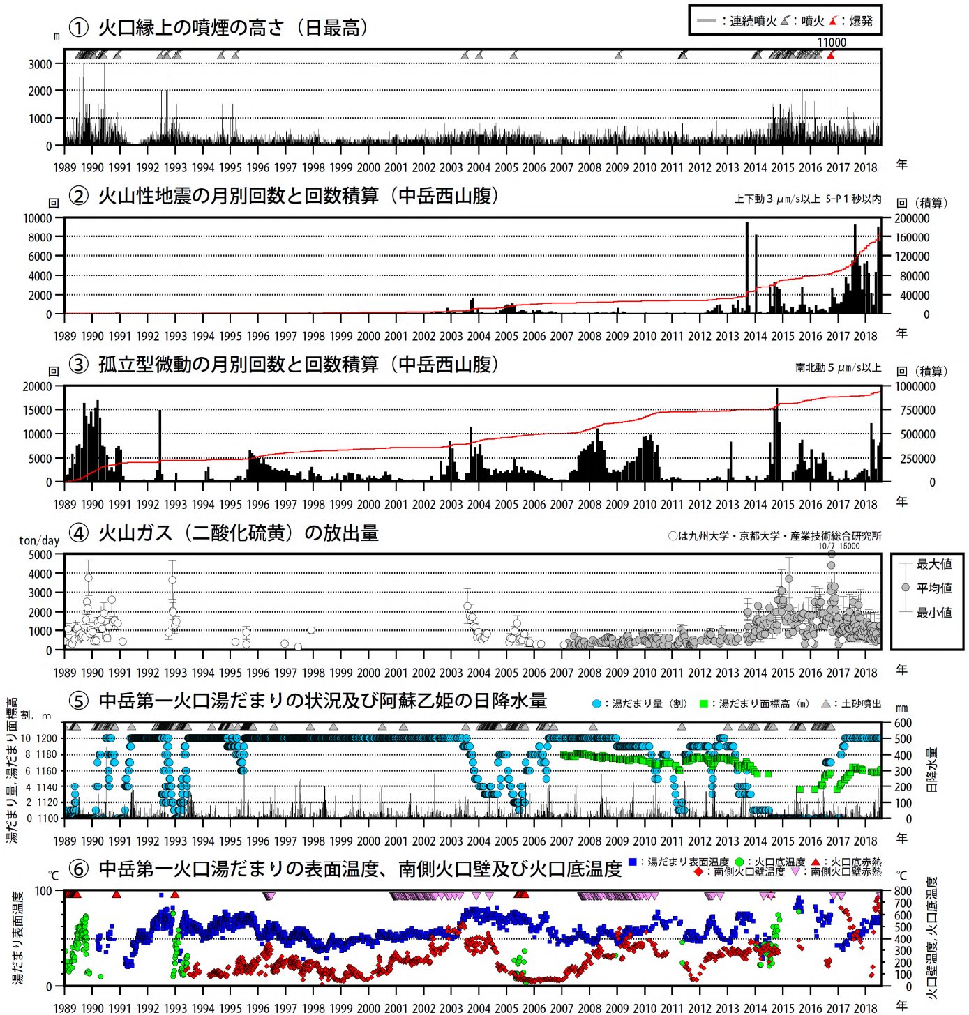
図 9 阿蘇山 火山活動経過図（1989 年 1 月～2018 年 7 月）
