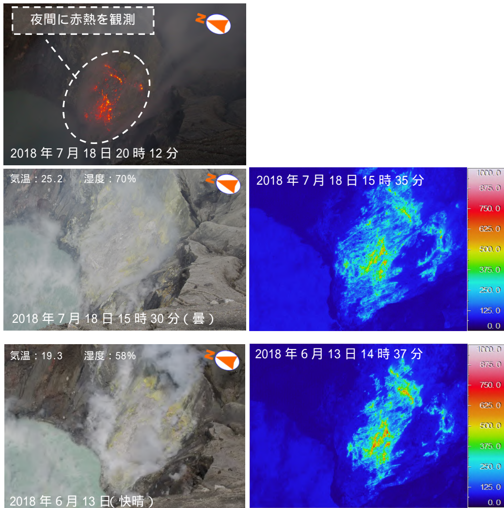
図7 阿蘇山 中岳第一火口南側火口壁の状況(中岳第一火口南西側から観測)
