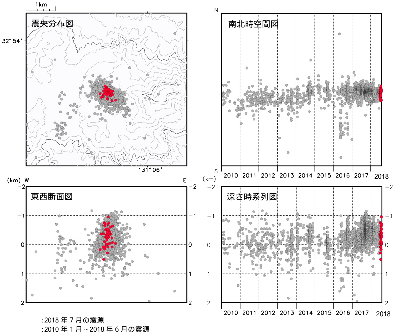
図10 阿蘇山 火山性地震の震源分布(2010年1月~2018年7月)
