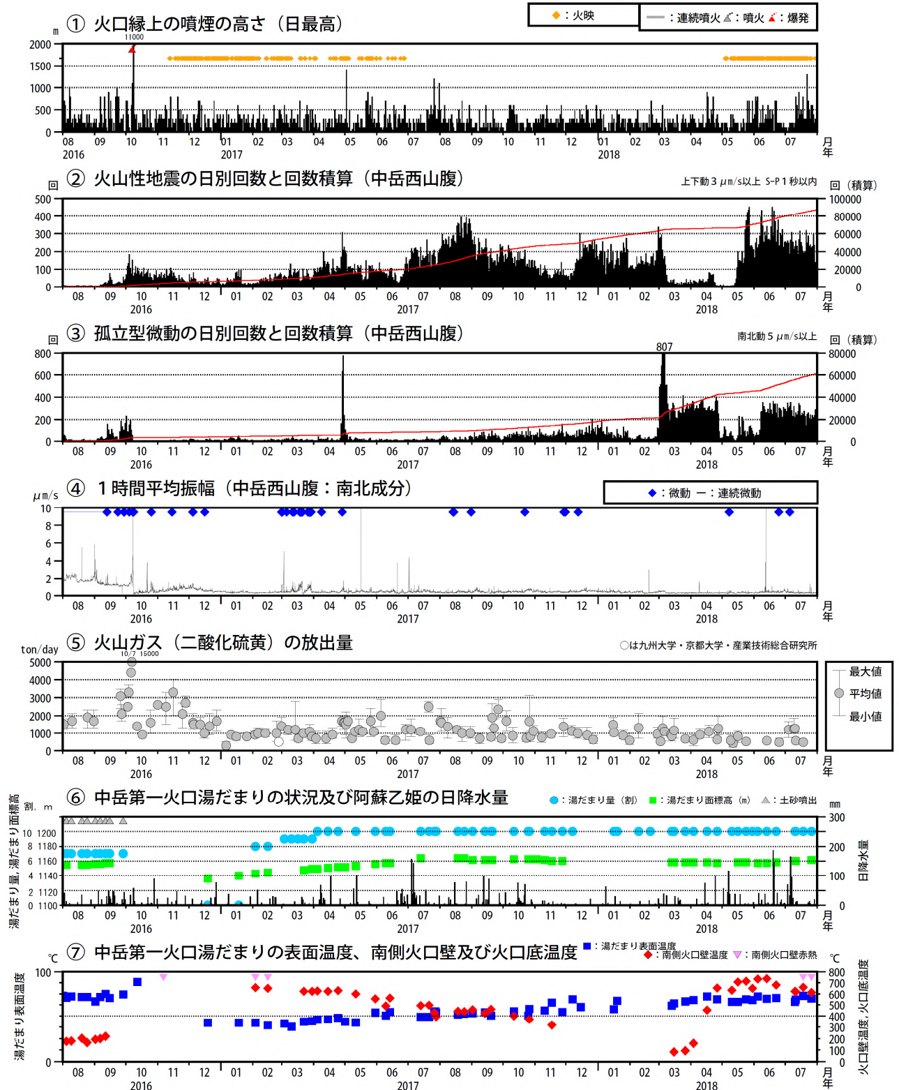
図8 阿蘇山 火山活動経過図(2016年8月~2018年7月)
