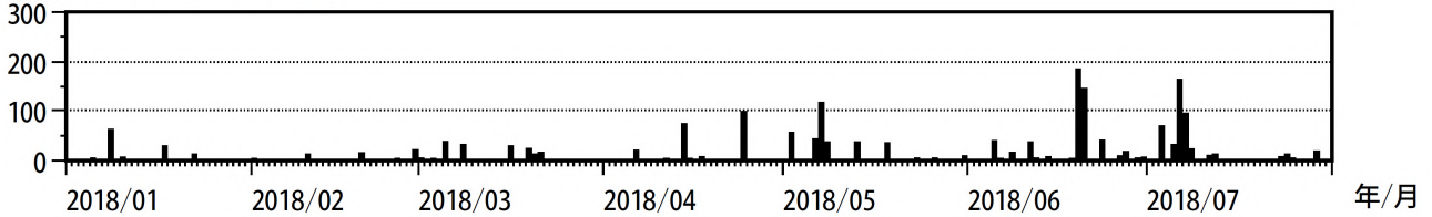
図 11 阿蘇山 古坊中観測点の傾斜変動及び阿蘇乙姫地域気象観測所の日降水量 (2018年1月～2018年7月)
