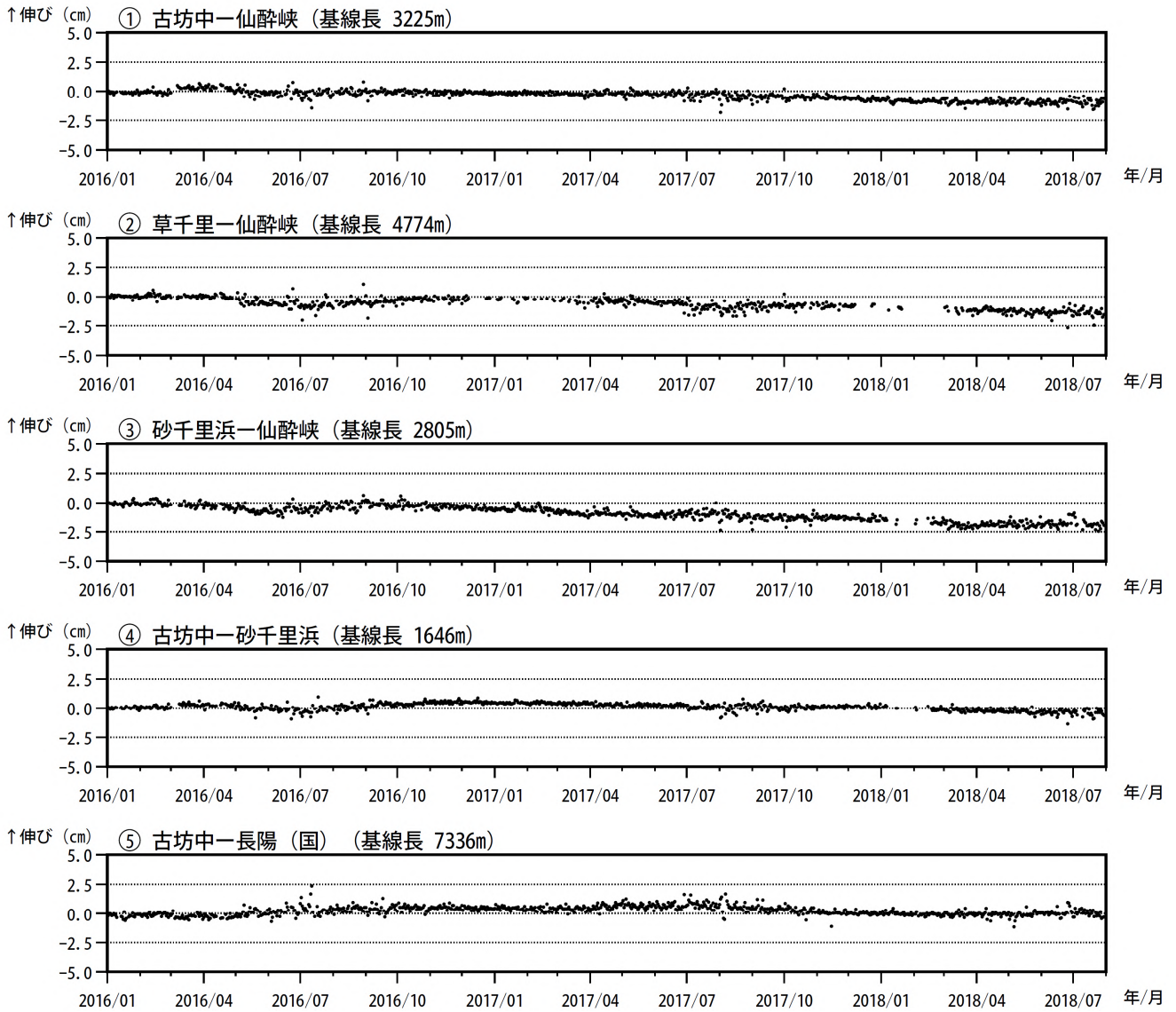
図 12-2 阿蘇山 GNSS 観測による短期の基線長変化（2016 年 1 月～2018 年 7 月）
