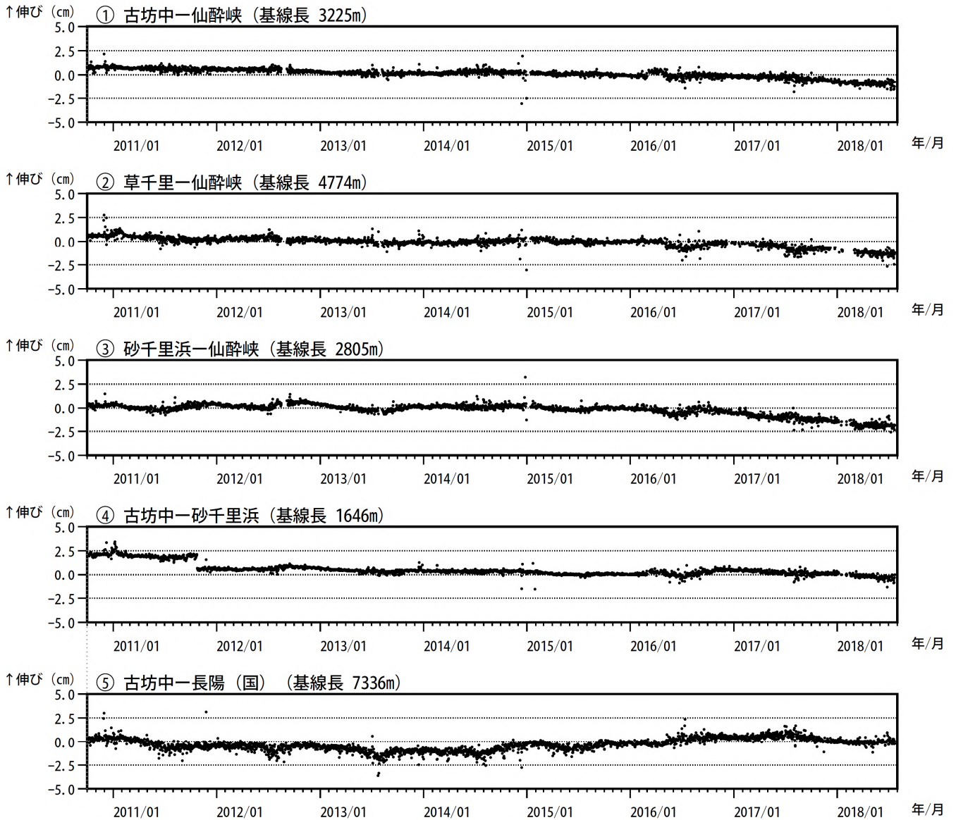
図 12-1 阿蘇山 GNSS連続観測による長期の基線長変化（2010 年 10 月～2018 年 7 月）
