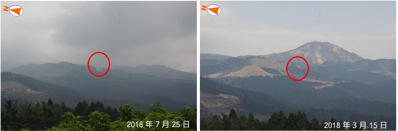
図 14 阿蘇山 南阿蘇村吉岡の噴気（赤丸内）（南阿蘇村長陽から撮影） 前回（3月15日）と同様に白色の噴気を確認しました。
