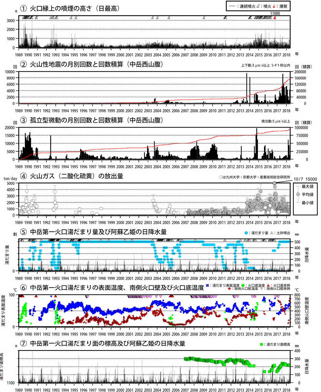
図 6 阿蘇山 火山活動経過図（1989 年 1 月～2018 年 5 月）
