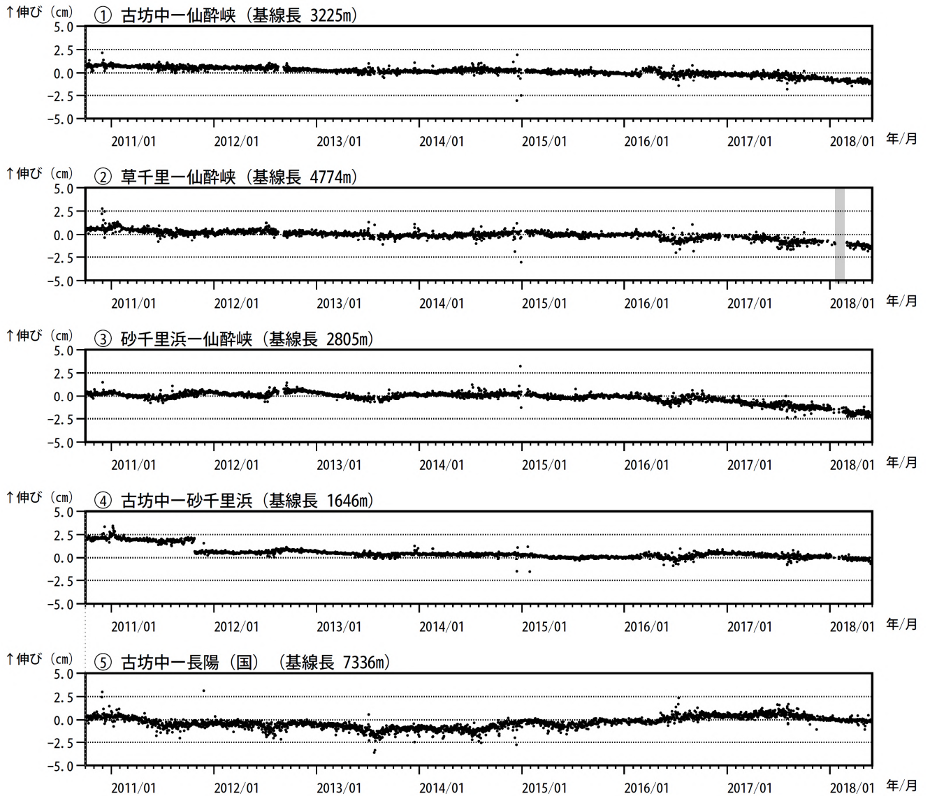
図 9-1 阿蘇山 GNSS連続観測による長期の基線長変化（2010 年 10 月～2018 年 5 月）
