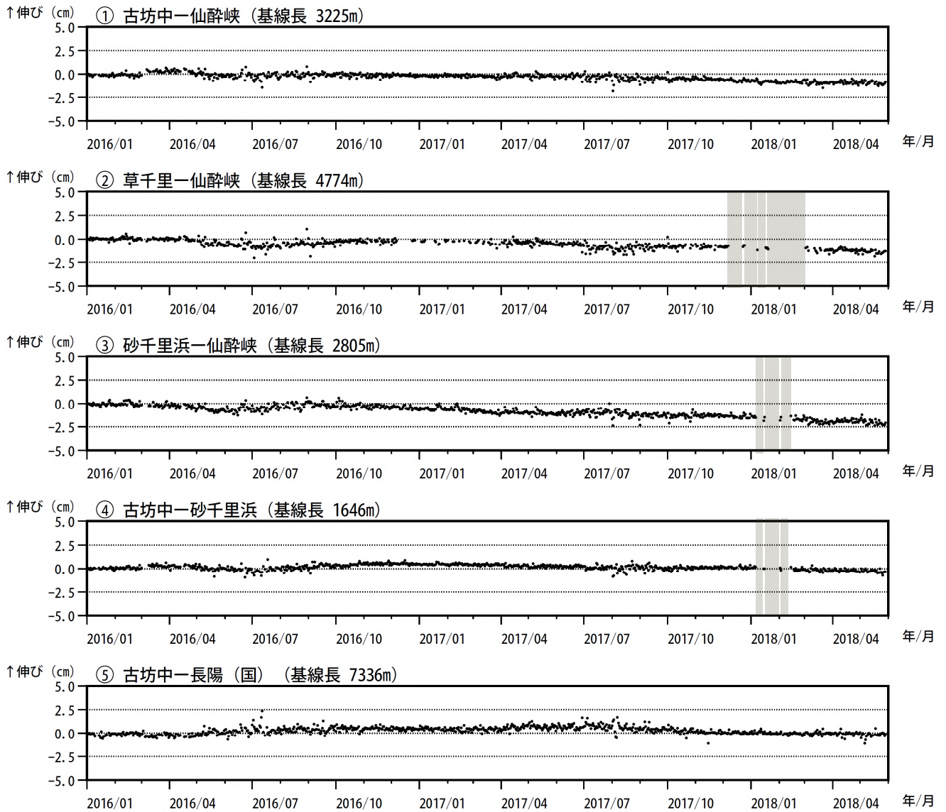
図 9-2 阿蘇山 GNSS 観測による短期の基線長変化（2016 年 1 月～2018 年 5 月） GNSS 連続観測では、火山活動に伴う特段の変化は認められません。
