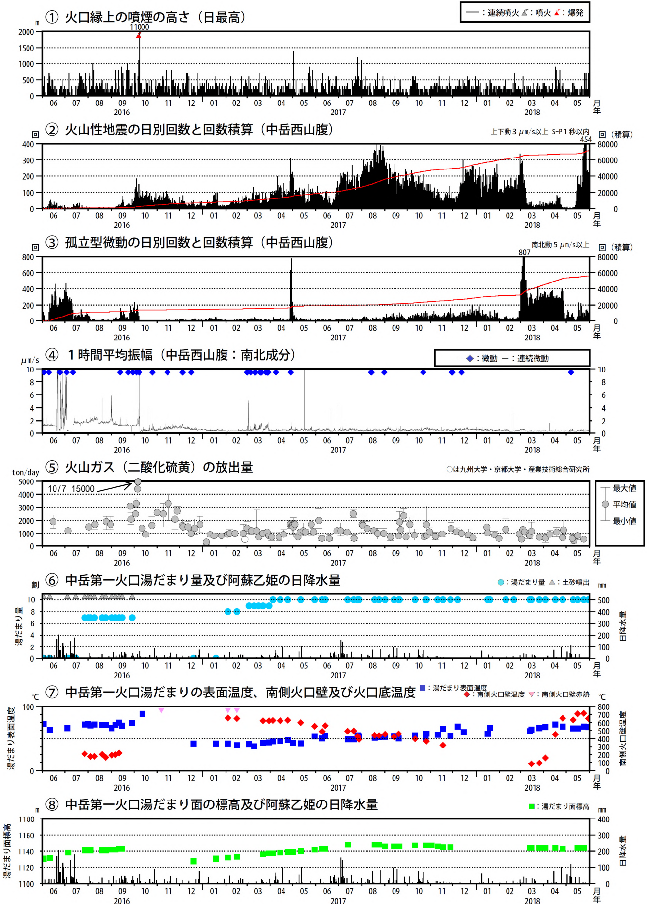
図5 阿蘇山 火山活動経過図（2016年6月～2018年5月）
