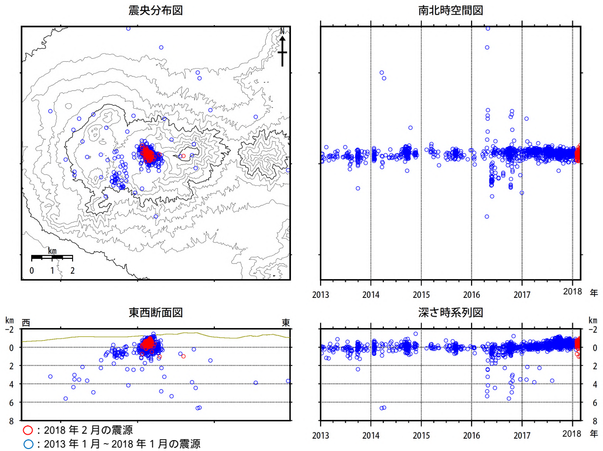
図 8 阿蘇山 火山性地震の震源分布（2013 年 1 月 ~ 2018 年 2 月）
