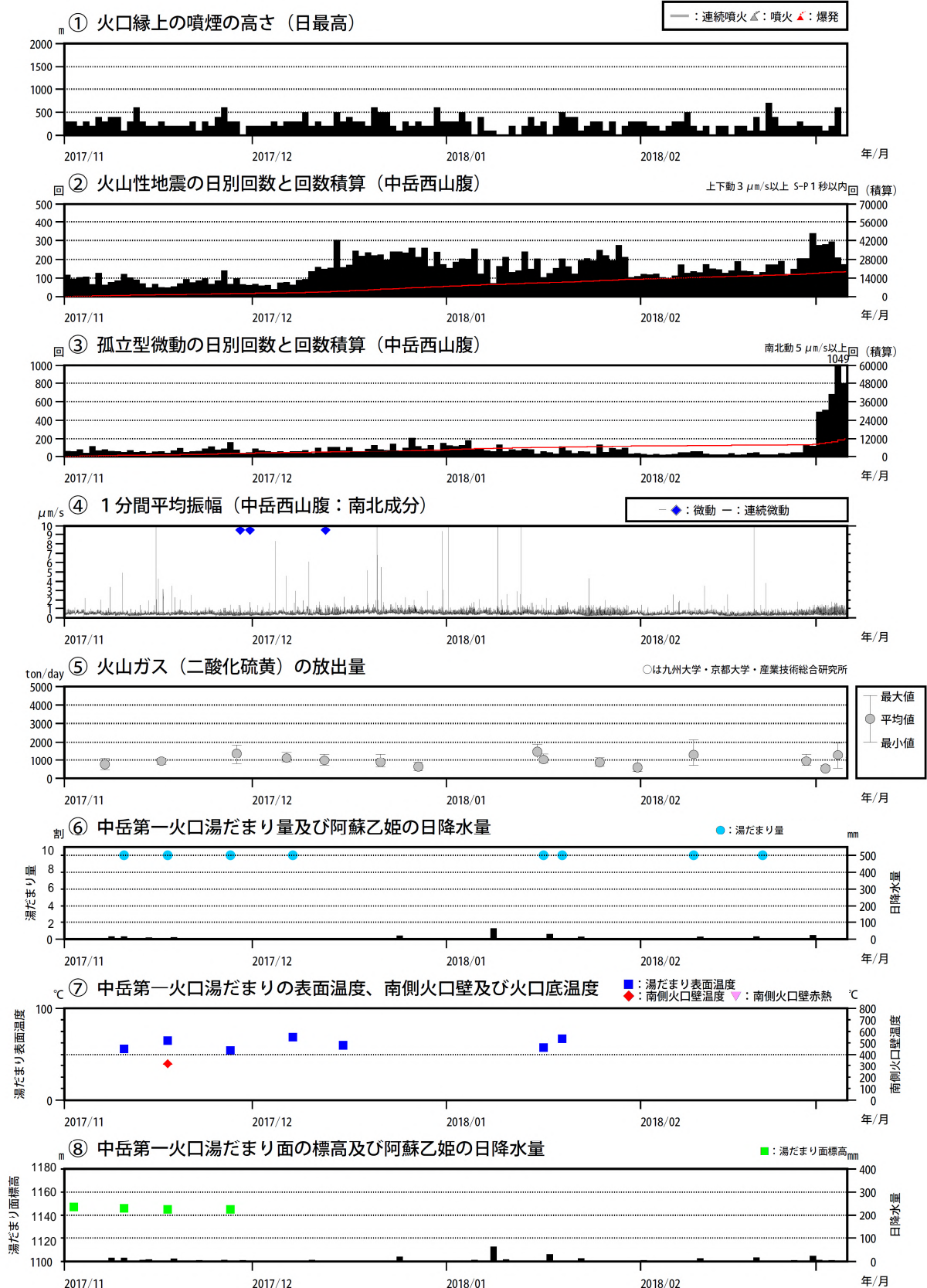
図 7 阿蘇山 火山活動経過図（2017 年 11 月～2018 年 3 月 5 日（期間外））
