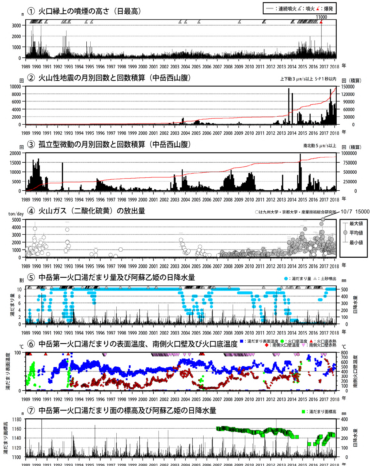
図 6 阿蘇山 火山活動経過図（1989 年 1 月～2018 年 2 月）
