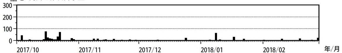
図 9 阿蘇山 古坊中観測点の傾斜変動（2017 年 10 月 ~ 2018 年 2 月）
