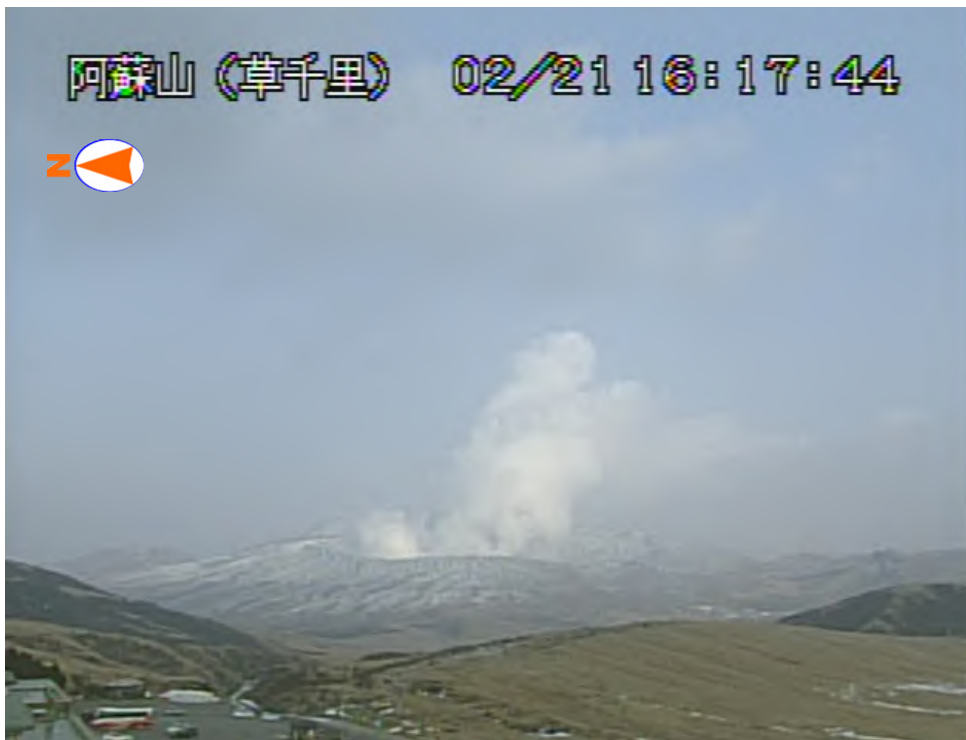
図1 阿蘇山 噴煙の状況（2月21日、草千里監視カメラによる）
