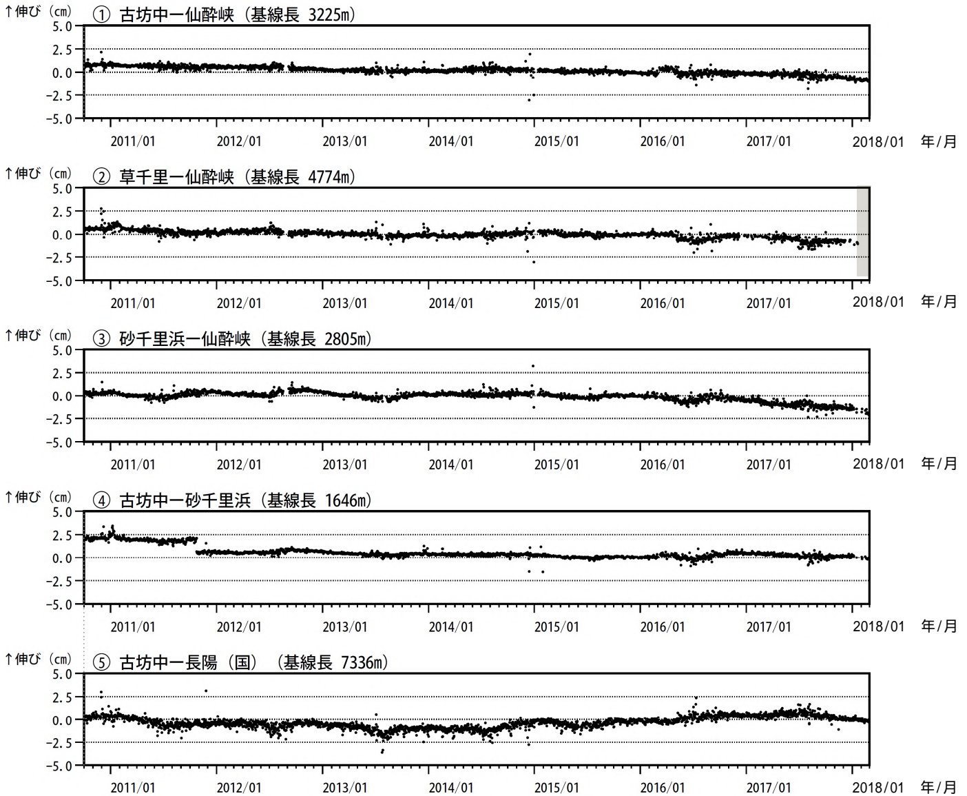
図 10-1 阿蘇山 GNSS連続観測による長期の基線長変化(2010年10月~2018年2月)
