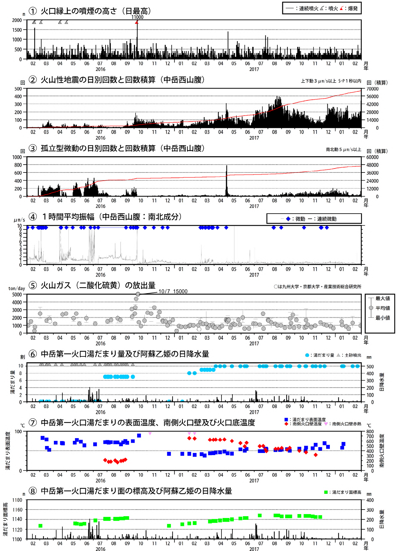
図5 阿蘇山 火山活動経過図（2016年2月～2018年2月）
