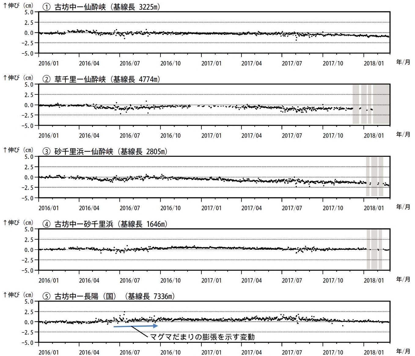
図 10-2 阿蘇山 GNSS 観測による短期の基線長変化（2016 年 1 月～2018 年 2 月） GNSS 連続観測では、火山活動に伴う特段の変化は認められません。
