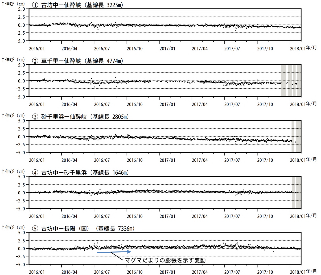
図 9-2 阿蘇山 GNSS 観測による短期の基線長変化（2016 年 1 月～2018 年 1 月） GNSS 連続観測では、火山活動に伴う特段の変化は認められません。
