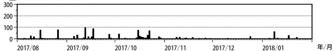
図8 阿蘇山 古坊中観測点の傾斜変動(2017年8月~2018年1月)
