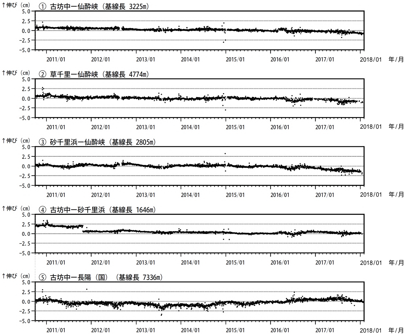
図 9-1 阿蘇山 GNSS連続観測による長期の基線長変化（2010 年 10 月～2018 年 1 月）
