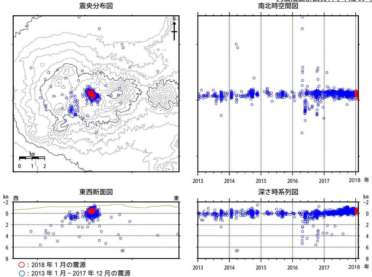
図7 阿蘇山 火山性地震の震源分布(2013年1月~2018年1月)
