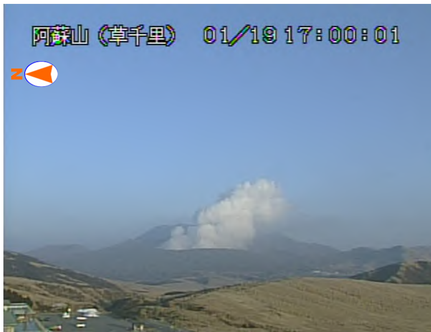
図 1 阿蘇山 噴煙の状況（1 月 19 日、草千里監視カメラによる）
