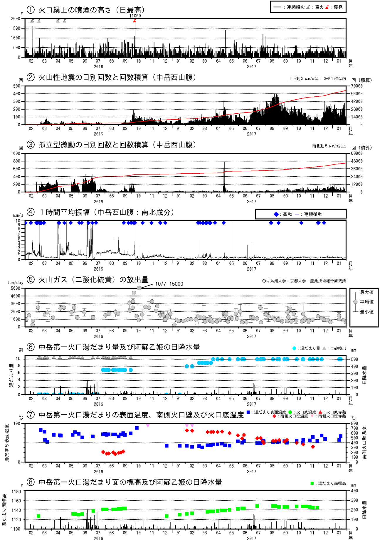
図5 阿蘇山 火山活動経過図(2016年2月~2018年1月)
