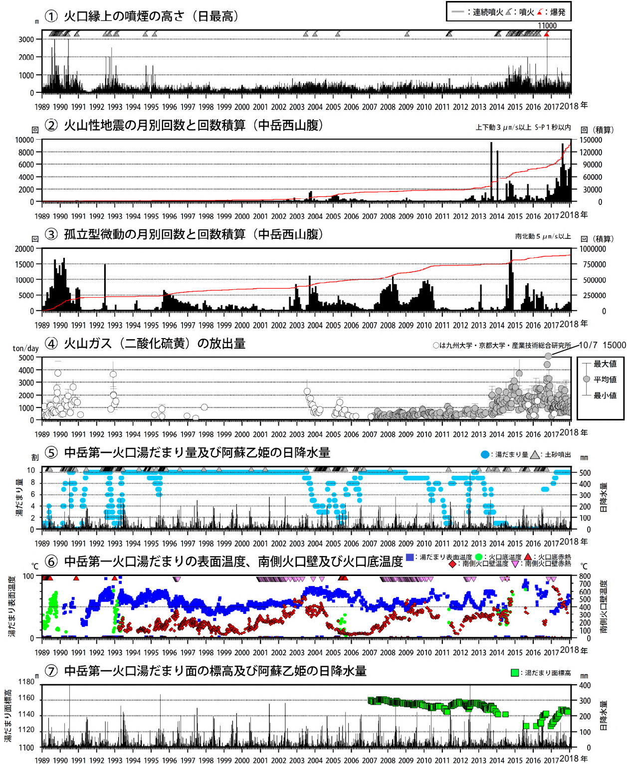
図 6 阿蘇山 火山活動経過図（1989年1月～2018年1月）
