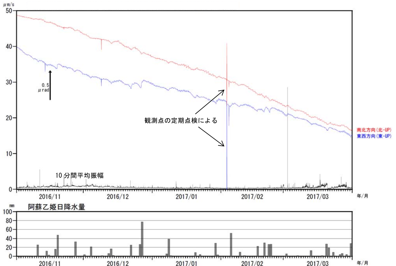
図 7 阿蘇山 古坊中観測点の傾斜変動（時間値）と地震計上下動の 10 分間平均振幅（2016 年 11 月～2017 年 3 月）
