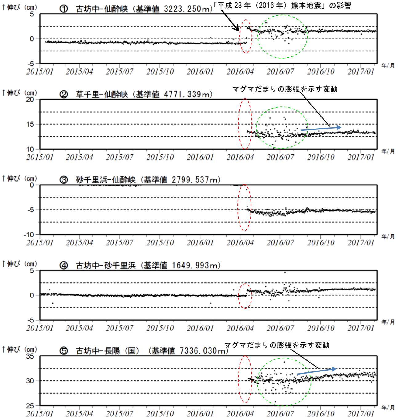
図 10-2 阿蘇山 GNSS 観測による短期の基線長変化 (2015 年 1 月~2017 年 2 月 6 日)
