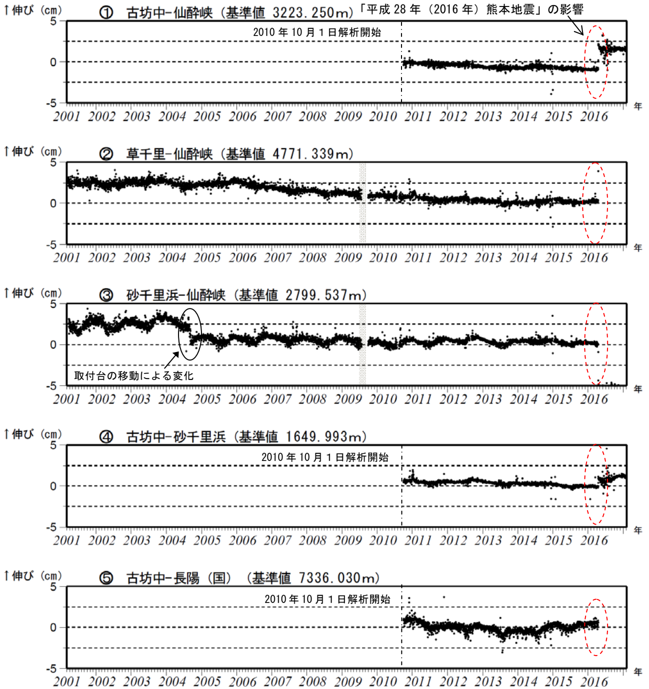
図 10-1 阿蘇山 GNSS連続観測による長期の基線長変化 (2001 年 3 月～2017 年 2 月 6 日)
