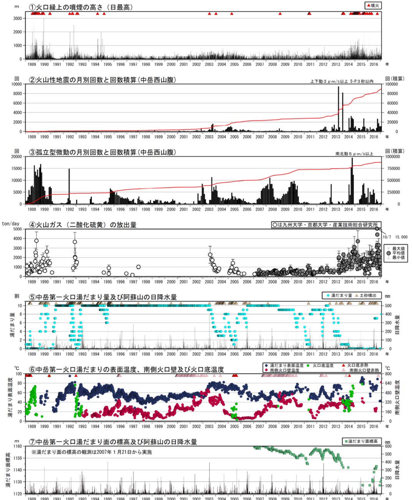
図6 阿蘇山 火山活動経過図（1989年1月～2017年2月6日）
