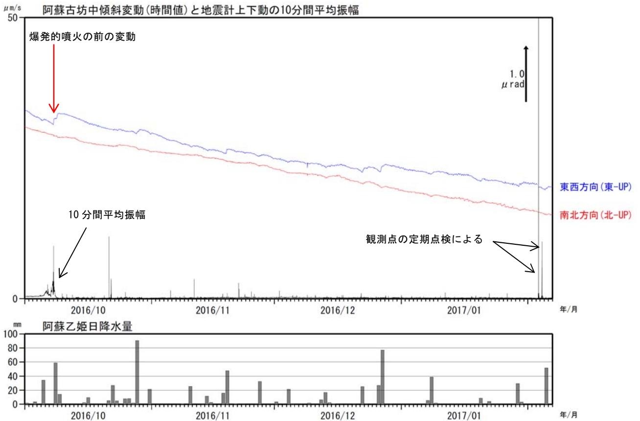
図 9 阿蘇山 古坊中傾斜変動と地震計上下動の 10 分間平均振幅 (2016 年 10 月～2017 年 2 月 6 日)
