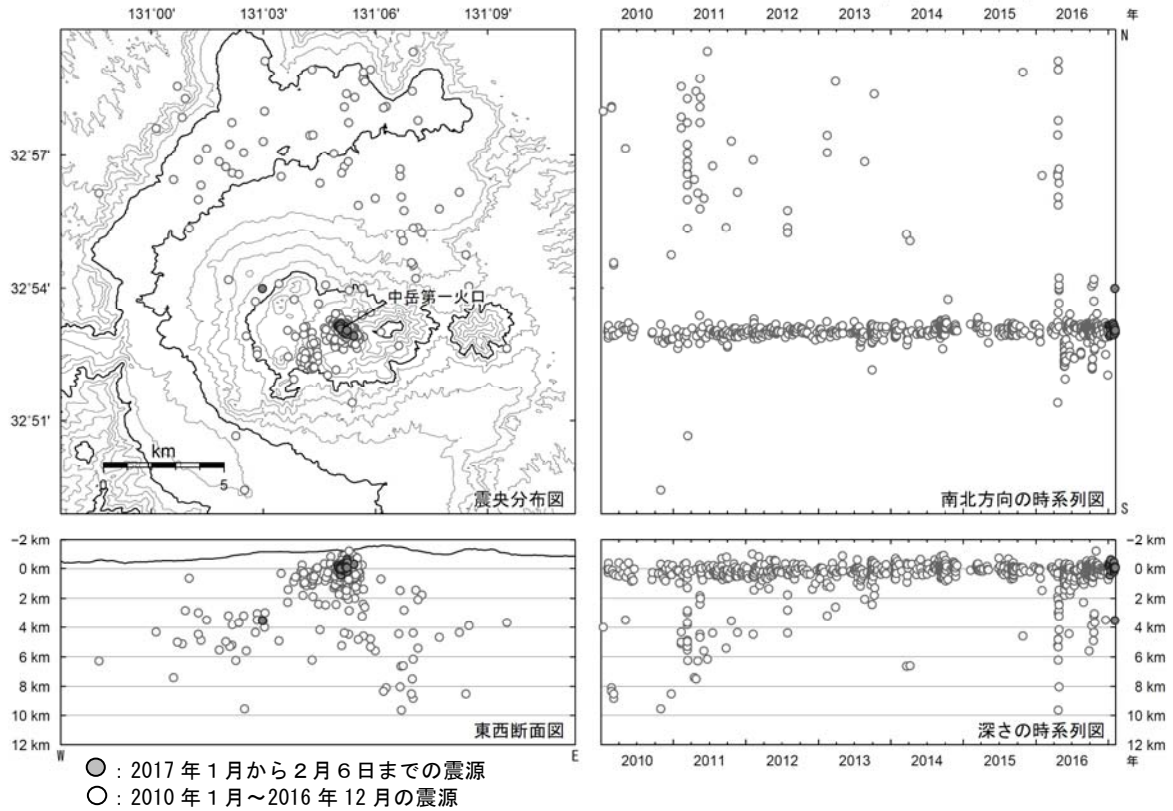
図 8 阿蘇山 火山性地震の震源分布 (2010 年 1 月～2017 年 2 月 6 日)
