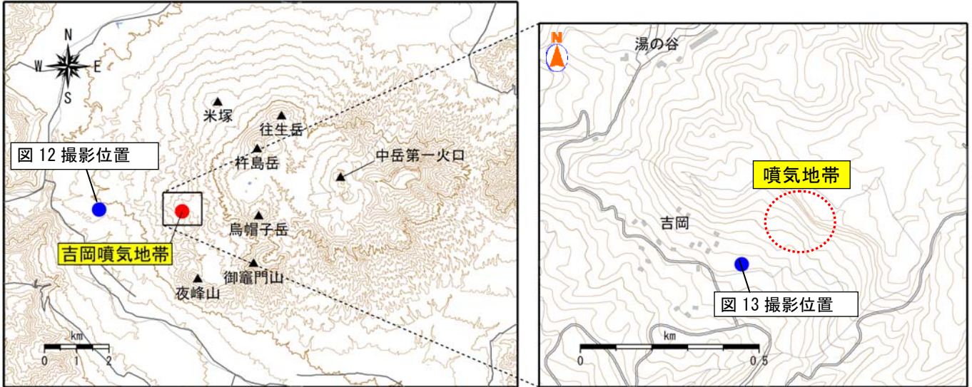
図14 阿蘇山 南阿蘇村吉岡の噴気地帯位置図
