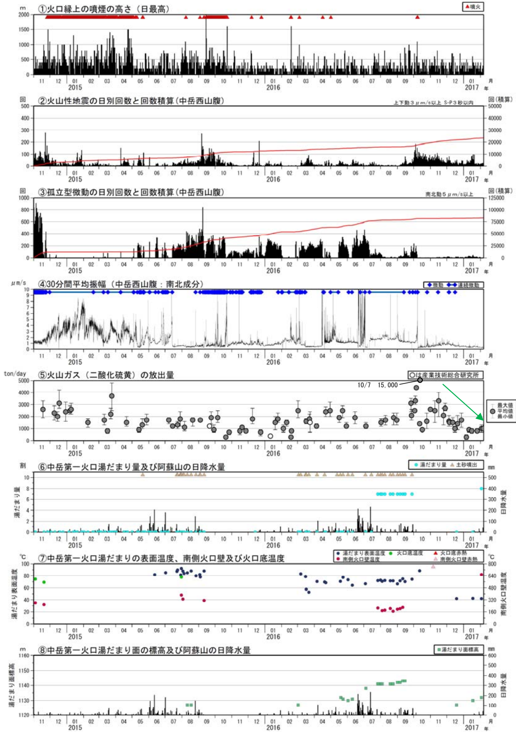
図7 阿蘇山 火山活動経過図（2014年11月～2017年2月6日）
