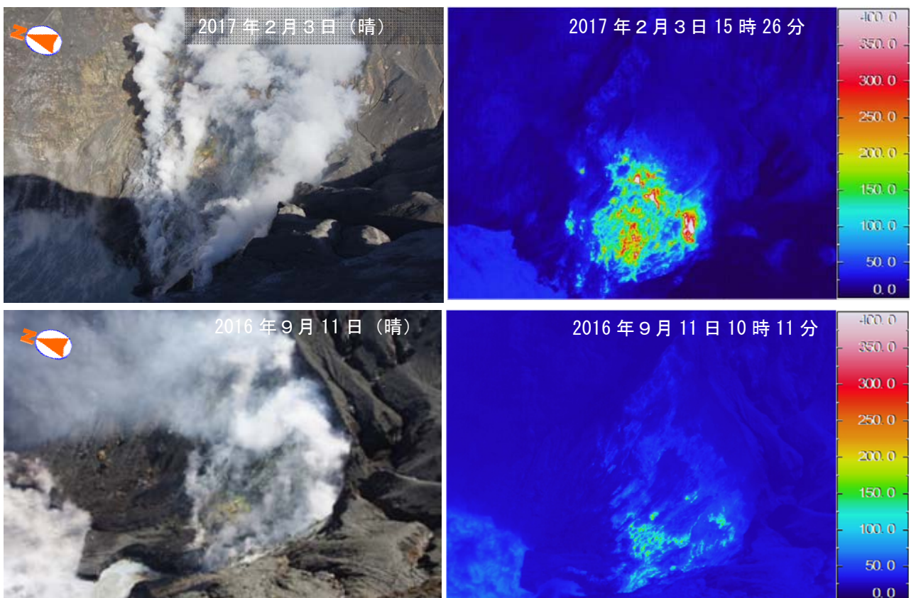
図 5 阿蘇山 中岳第一火口南側火口壁の温度分布（中岳第一火口南西側から撮影）
