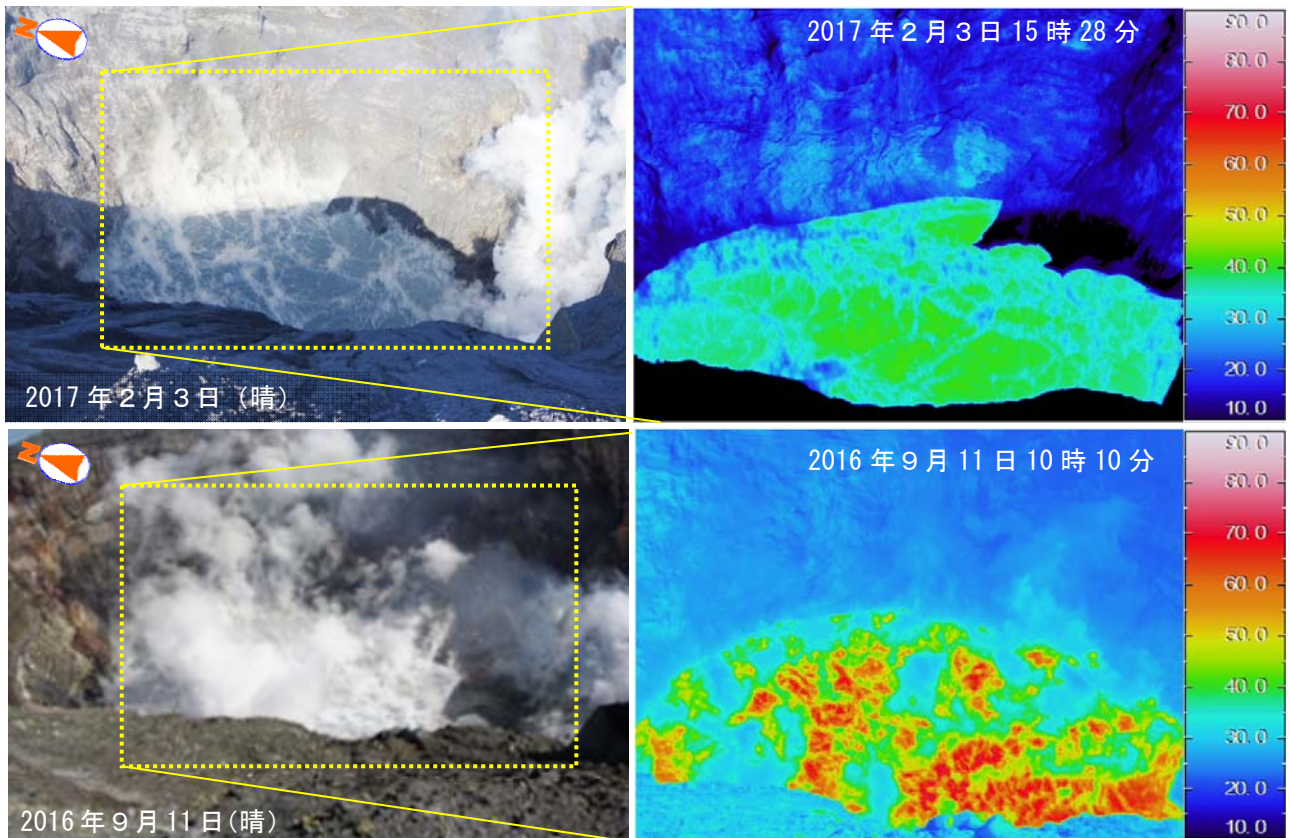
図 4 阿蘇山 中岳第一火口の状況と赤外熱映像装置による地表面温度分布（中岳第一火口南西側から撮影）
