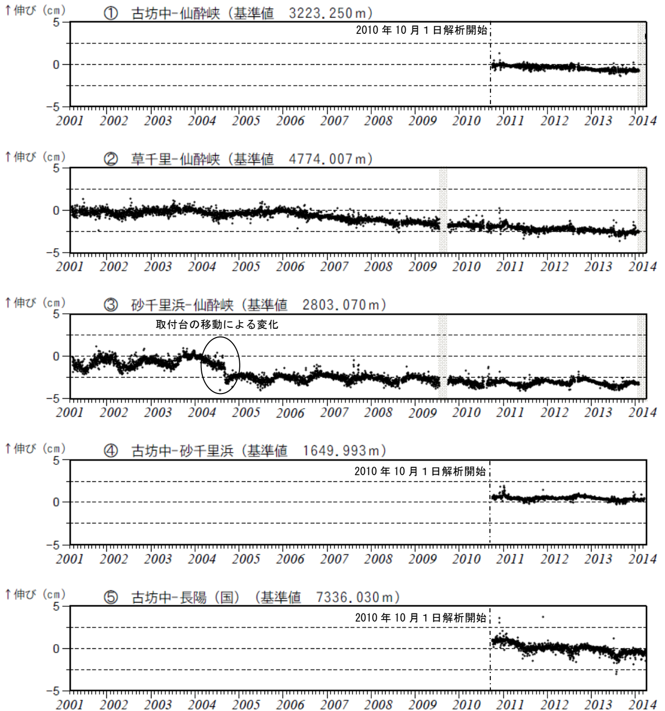
図 7 阿蘇山 GNSS連続観測による基線長変化（2001年3月～2014年3月）
