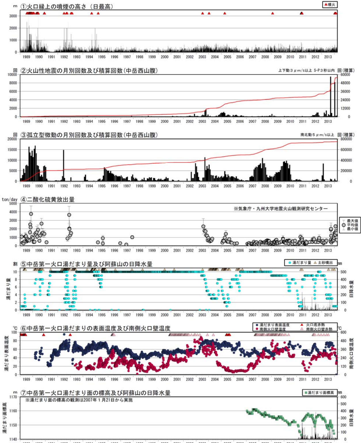
図3 阿蘇山 火山活動経過図（1989年1月～2014年3月）
