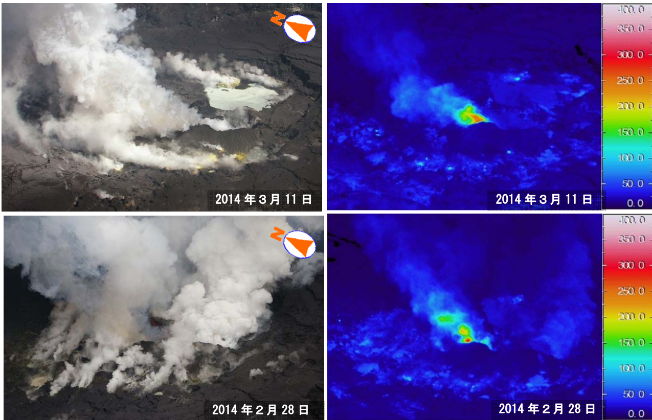
図 9 阿蘇山 赤外熱映像装置による中岳第一火口中央部の地表面温度分布
