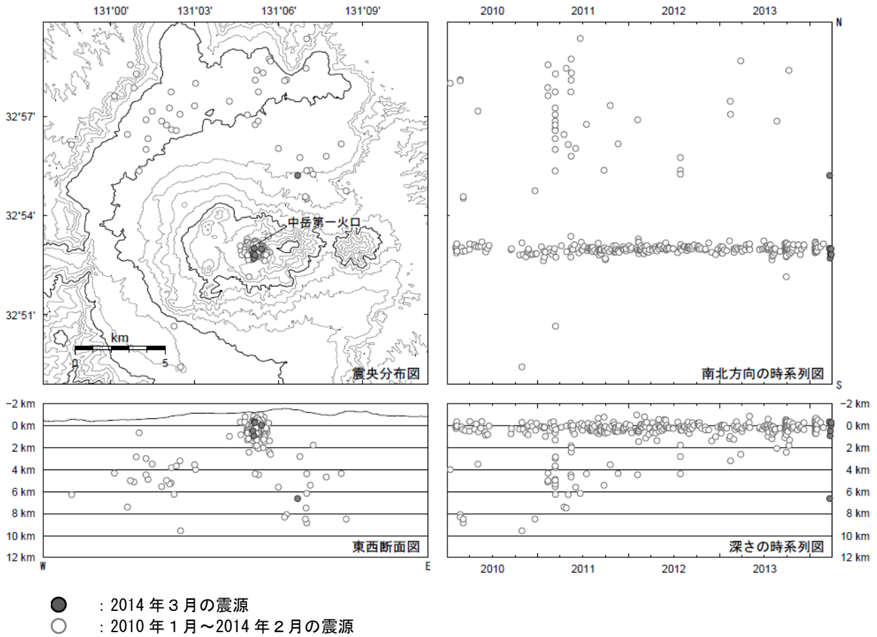
図5 阿蘇山 震源分布図（2010年1月～2014年3月）
