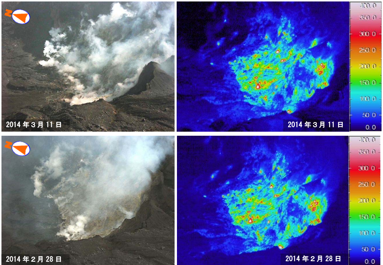
図 10 阿蘇山 赤外熱映像装置による中岳第一火口南側火口壁の地表面温度分布
