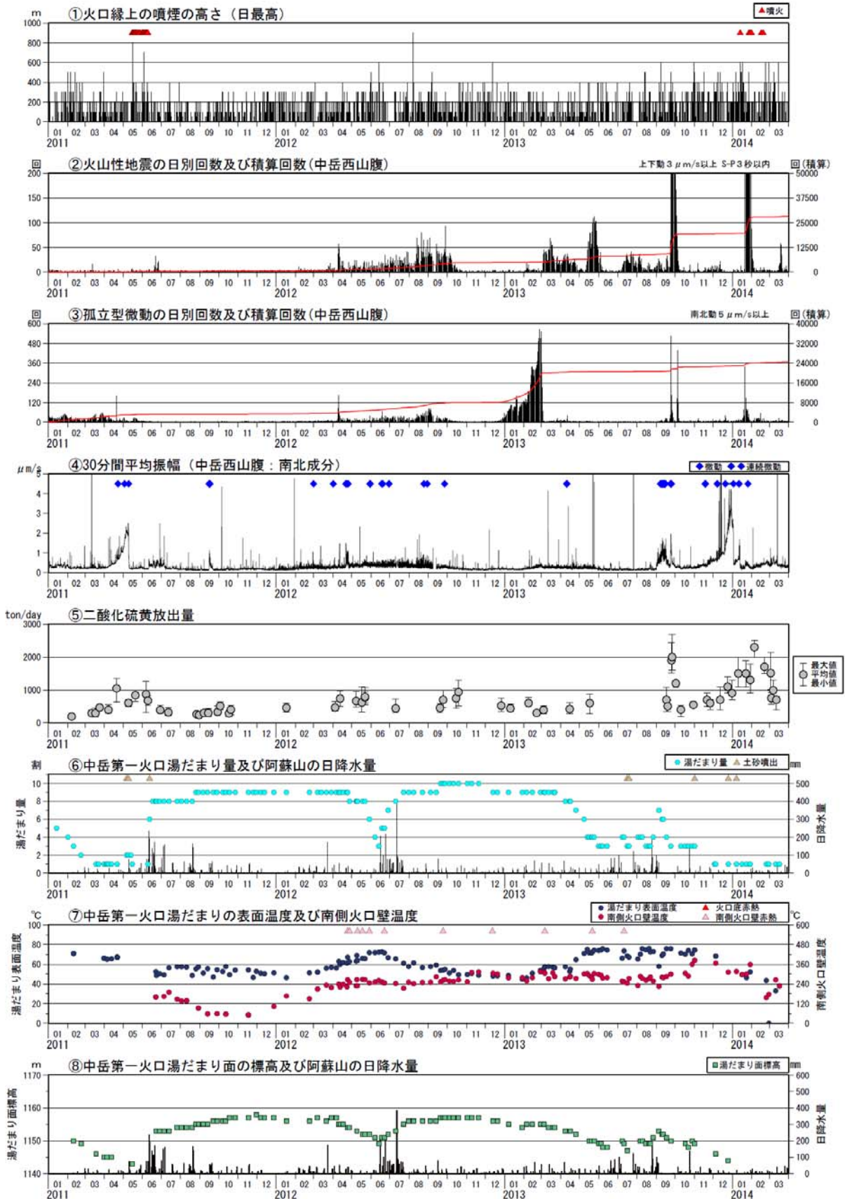
図 4 阿蘇山 火山活動経過図（2011 年 1 月～2014 年 3 月）
