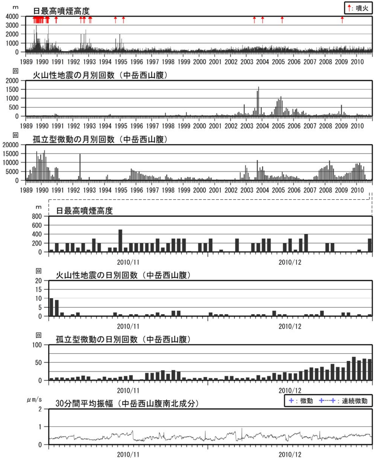
図 2 阿蘇山 噴煙、火山性地震、孤立型微動の状況（1989 年 1 月～2010 年 12 月）
