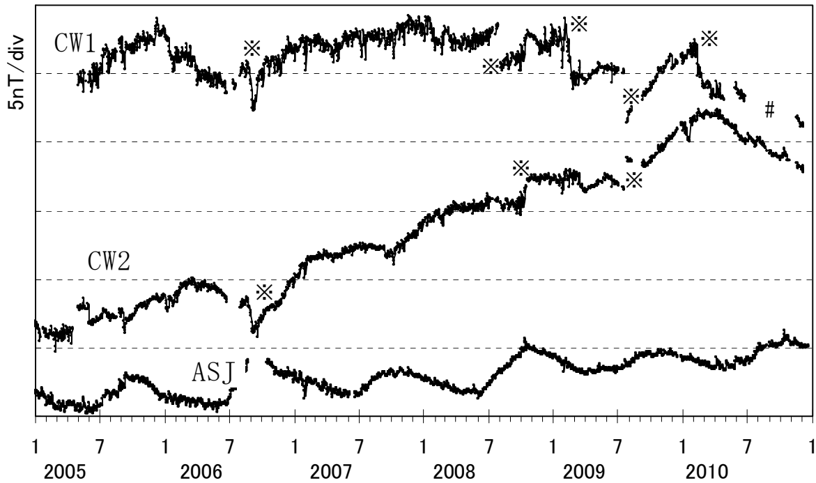
図 7 阿蘇山 全磁力連続観測による阿蘇山麓 (AHK) を基準とした中岳第一火口周辺の全磁力変化 (2005 年 1 月～2010 年 12 月)
