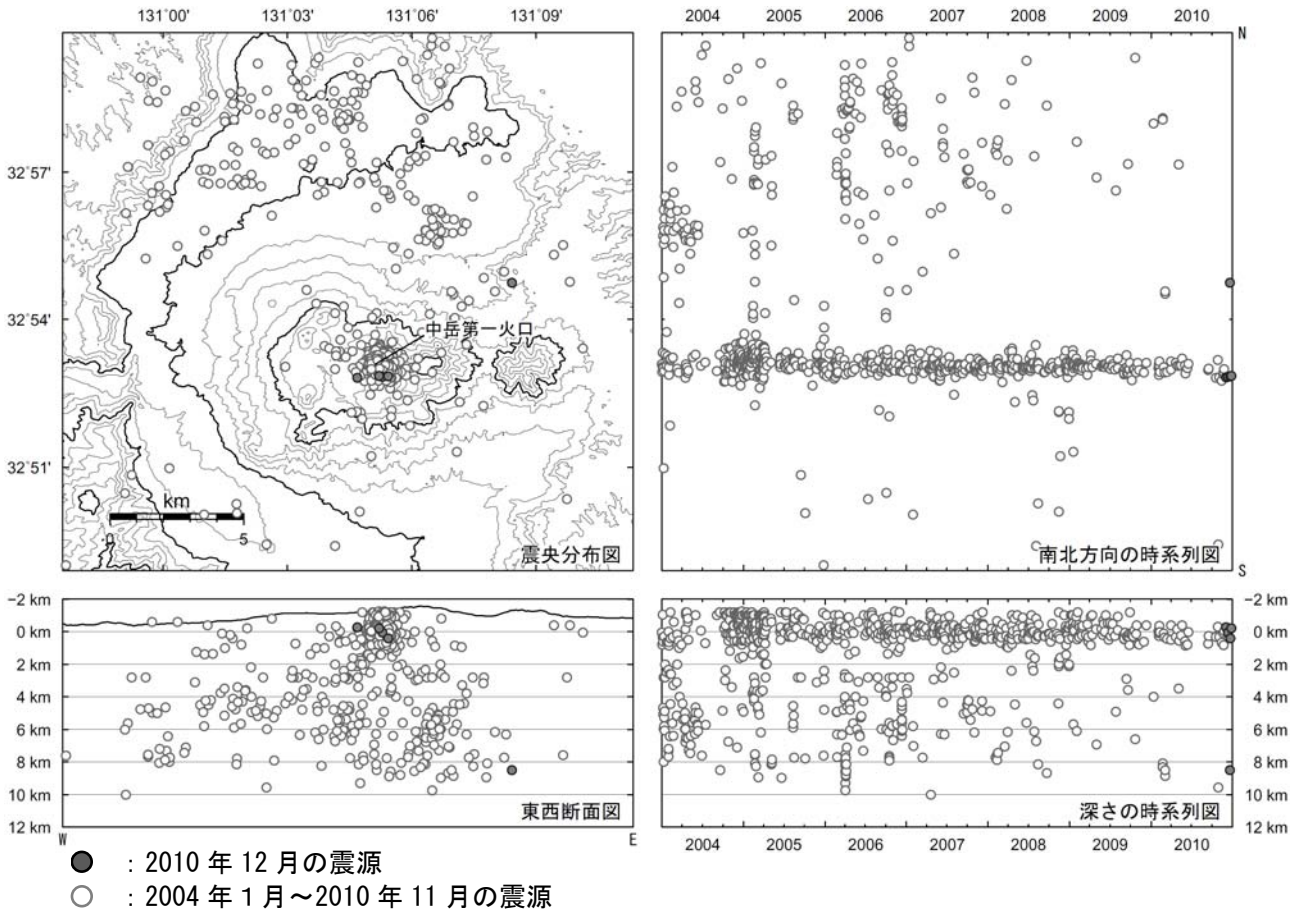
図 4※ 阿蘇山 震源分布図 (2004 年 1 月～2010 年 12 月) <12 月の状況>
