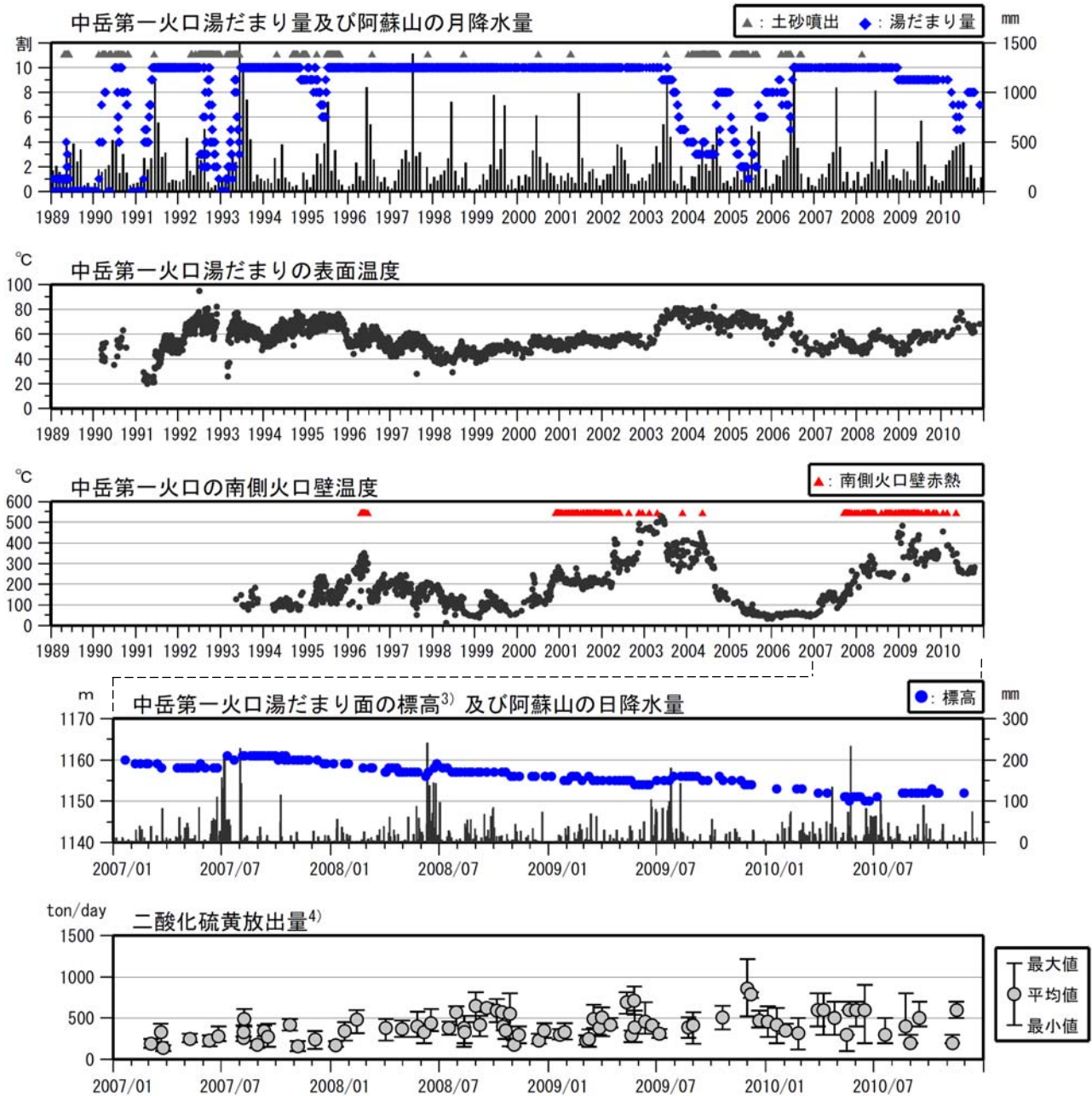
図 3※ 阿蘇山 湯だまり、火口壁、二氧化硫黄放出量の状況（1989 年 1 月～2010 年 12 月） <12 月の状況>
