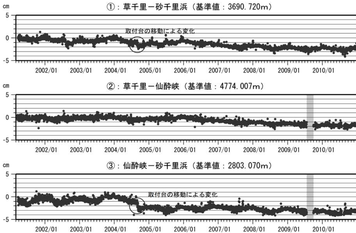
図 5 阿蘇山 GPS連続観測による基線長変化 (2001 年 3 月～2010 年 12 月)
