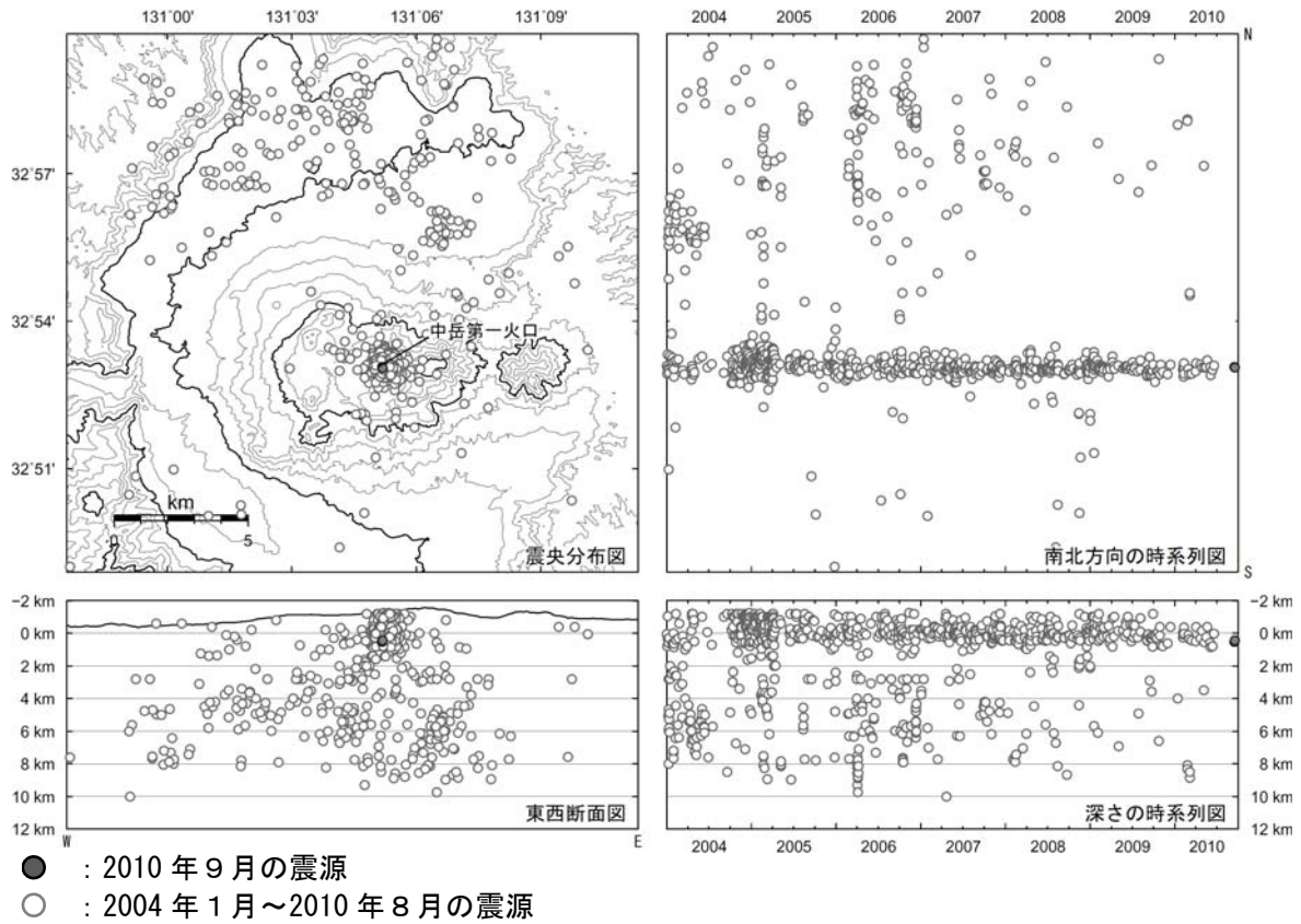
図 4 ※ 阿蘇山 震源分布図 (2004 年 1 月～2010 年 9 月)
