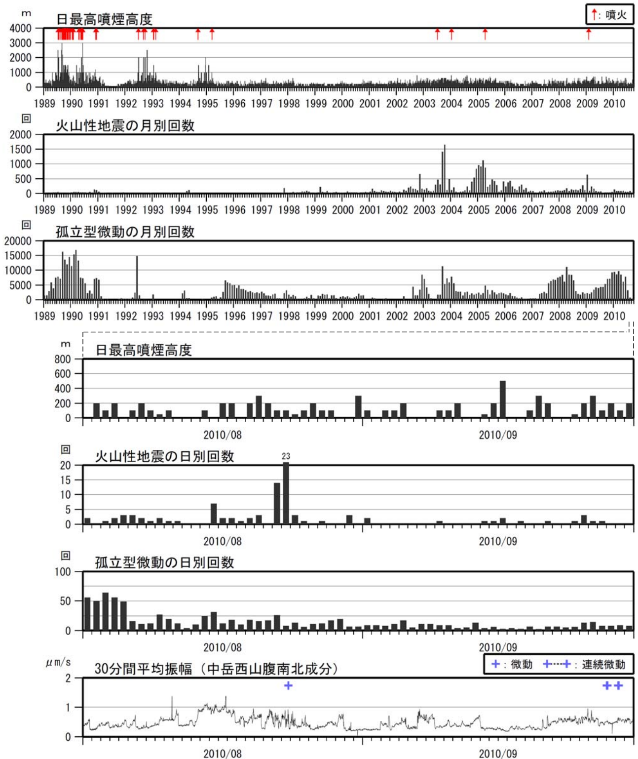
図 2 阿蘇山 噴煙、火山性地震、孤立型微動の状況（1989 年 1 月～2010 年 9 月）
