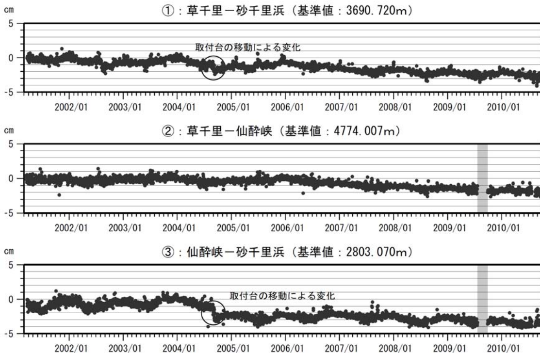
図 5 阿蘇山 GPS連続観測による基線長変化 (2001 年 3 月～2010 年 9 月)
