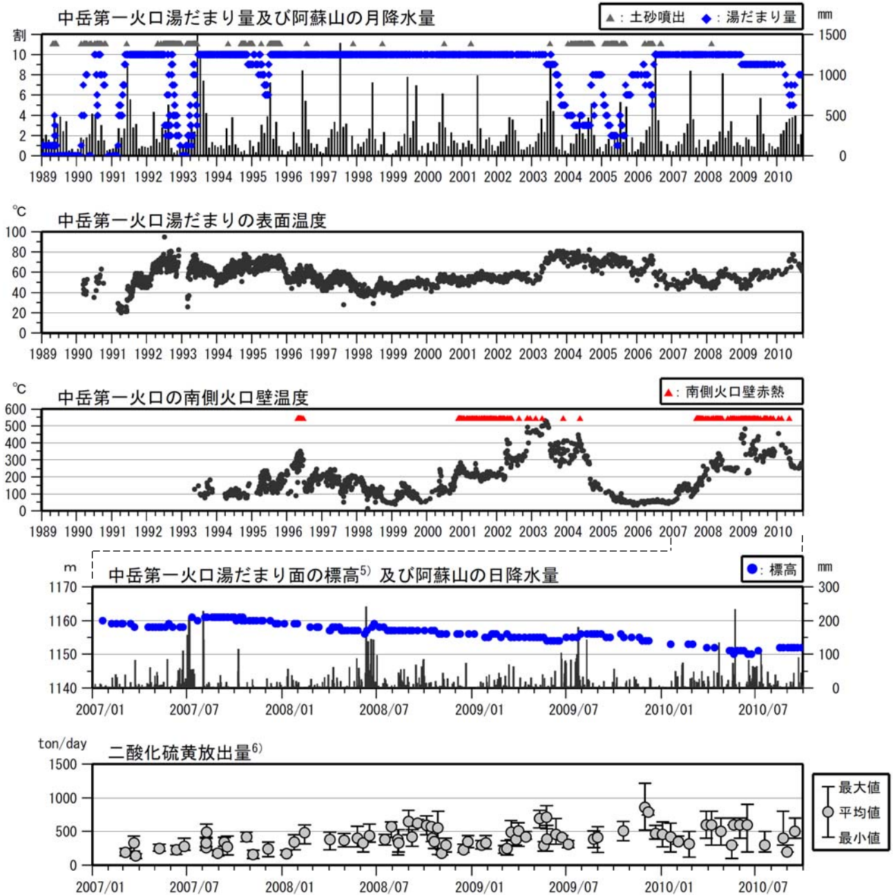
図 3※ 阿蘇山 湯だまり、火口壁、二氧化硫黄放出量の状況（1989 年 1 月～2010 年 9 月） < 9 月の状況 >
