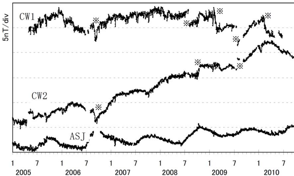
図 7 阿蘇山 全磁力連続観測による阿蘇山麓 (AHK) を基準とした中岳第一火口周辺の全磁力変化 (2005 年 1 月 ~ 2010 年 9 月)
