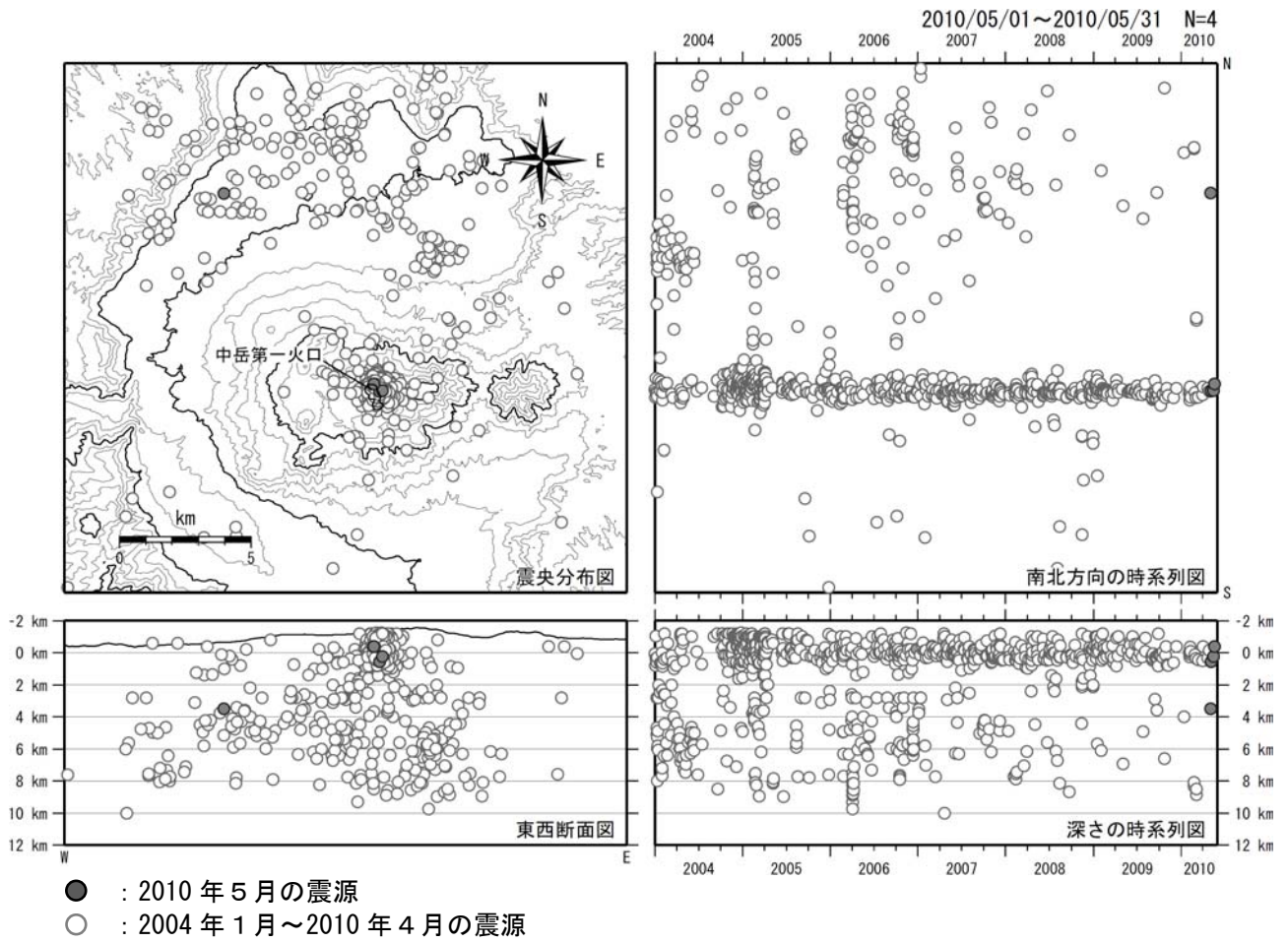
図 4※ 阿蘇山 震源分布図（2004 年 1 月～2010 年 5 月）
