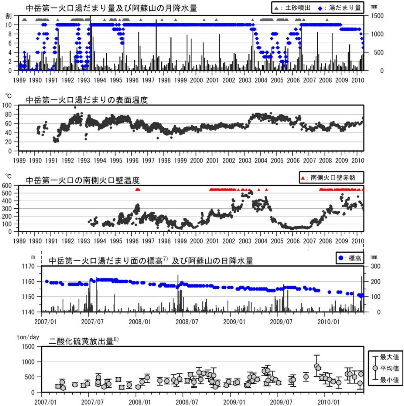
図 3※ 阿蘇山 火山活動経過図（1989 年 1 月～2010 年 5 月）
