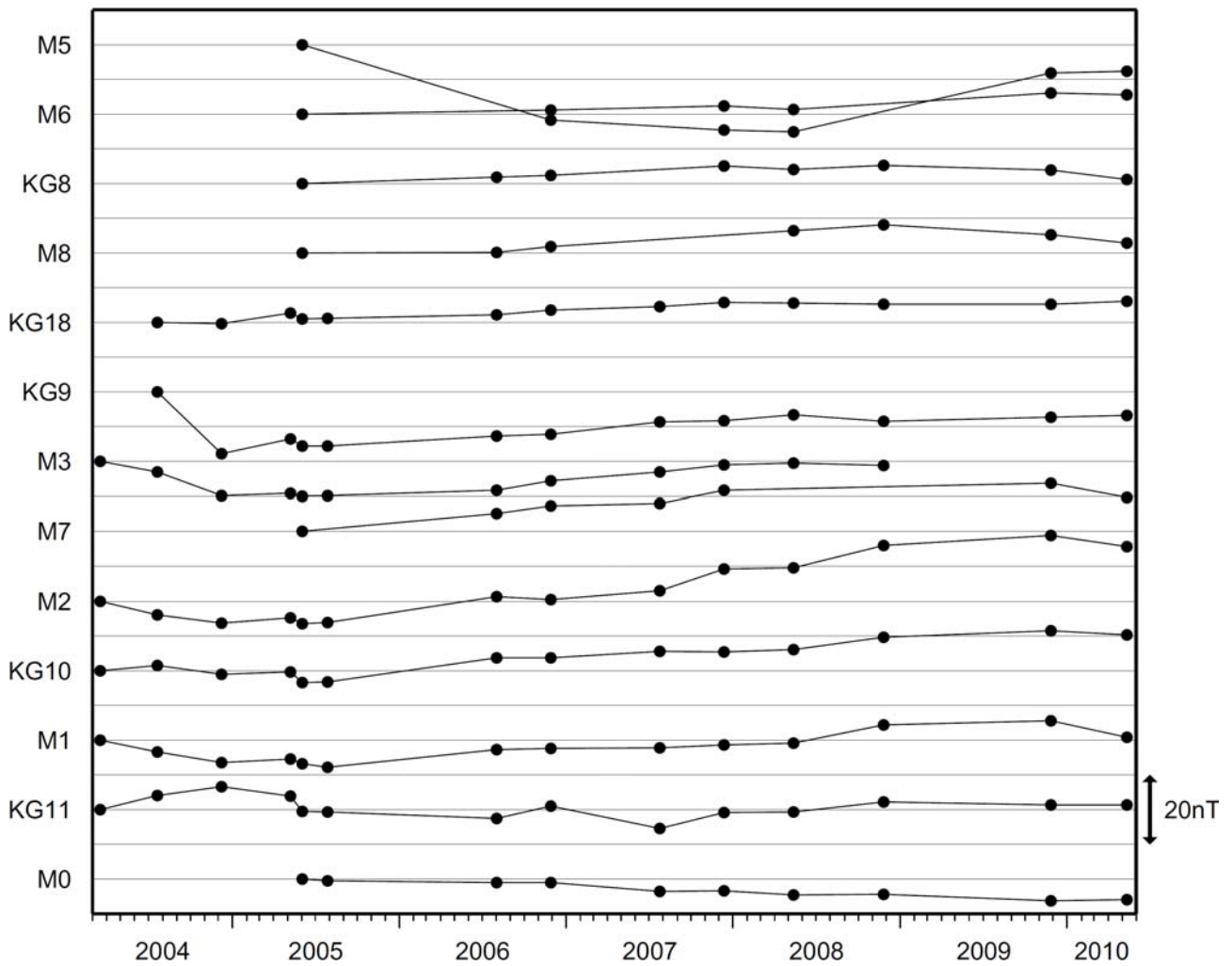
図7 阿蘇山 全磁力繰り返し観測による参照点 (M00) を基準とした中岳第一火口周辺の全磁力変化 (2004年3月~2010年5月)
