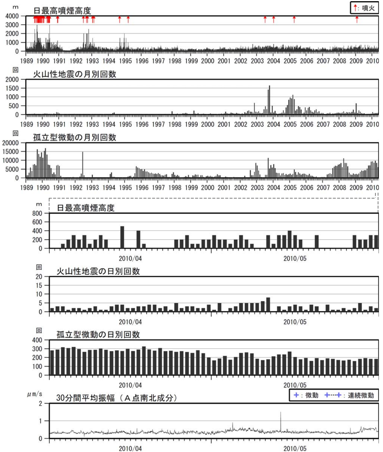
図 2 阿蘇山 火山活動経過図（1989 年 1 月～2010 年 5 月）
