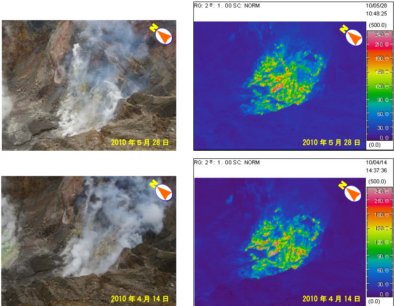
図 10 阿蘇山 赤外熱映像装置 9) による中岳第一火口南側火口壁の地表面温度分布 熱異常域の分布は前期間と比べて大きな変化はありませんでした。
