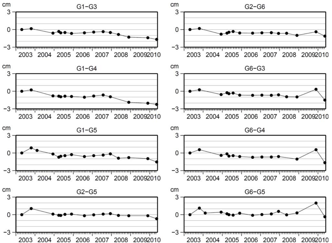
図9 阿蘇山 GPS繰り返し観測による基線長変化 (2003年4月～2010年5月) 火山活動によると考えられる変化は認められませんでした。
