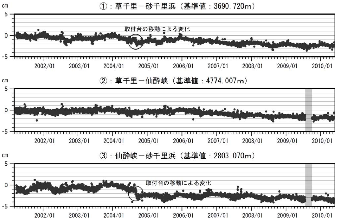
図 8 阿蘇山 GPS連続観測による基線長変化（2001 年 3 月～2010 年 5 月） 中岳第一火口を囲むいずれの基線においても長期的な縮みの傾向が続いています。 < 5 月の状況 > 火山活動によると考えられる変化は認められませんでした。
