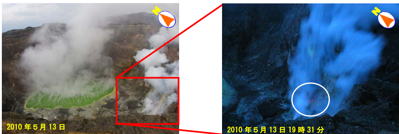
図 11 阿蘇山 夜間に実施した現地調査の状況 南側火口壁の丸印部分で赤熱現象を観測しました。
