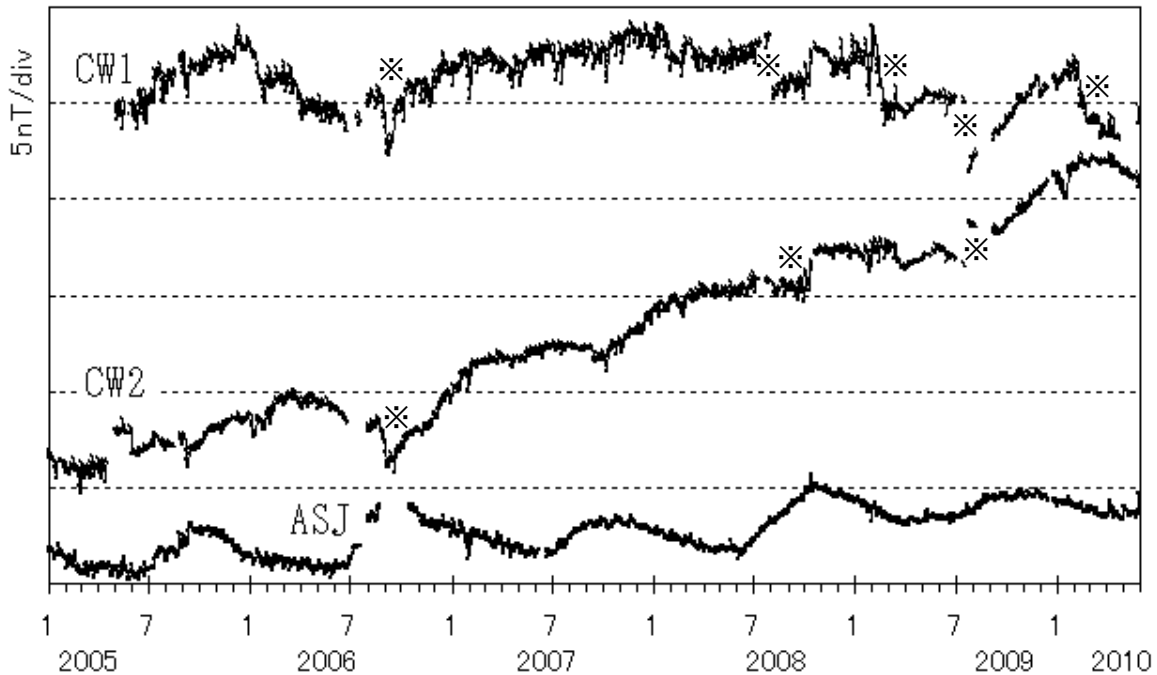
図 6 阿蘇山 全磁力連続観測による阿蘇山麓 (AHK) を基準とした中岳第一火口周辺の全磁力変化 (2005 年 1 月～2010 年 5 月)
