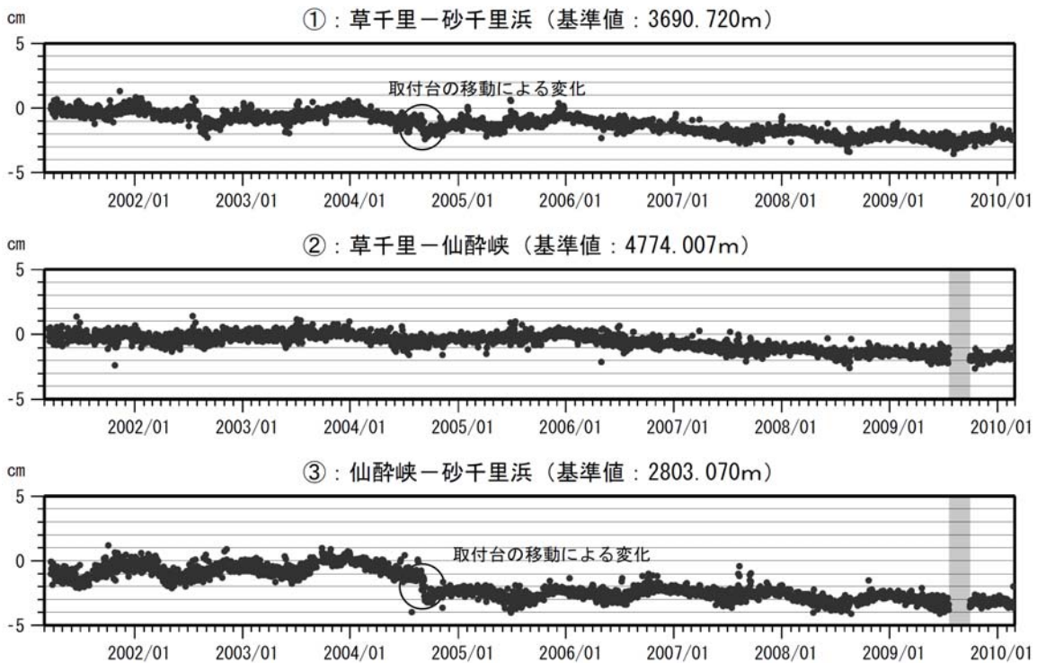
図 5 阿蘇山 GPS連続観測による基線長変化 (2001 年 3 月～2010 年 2 月)
