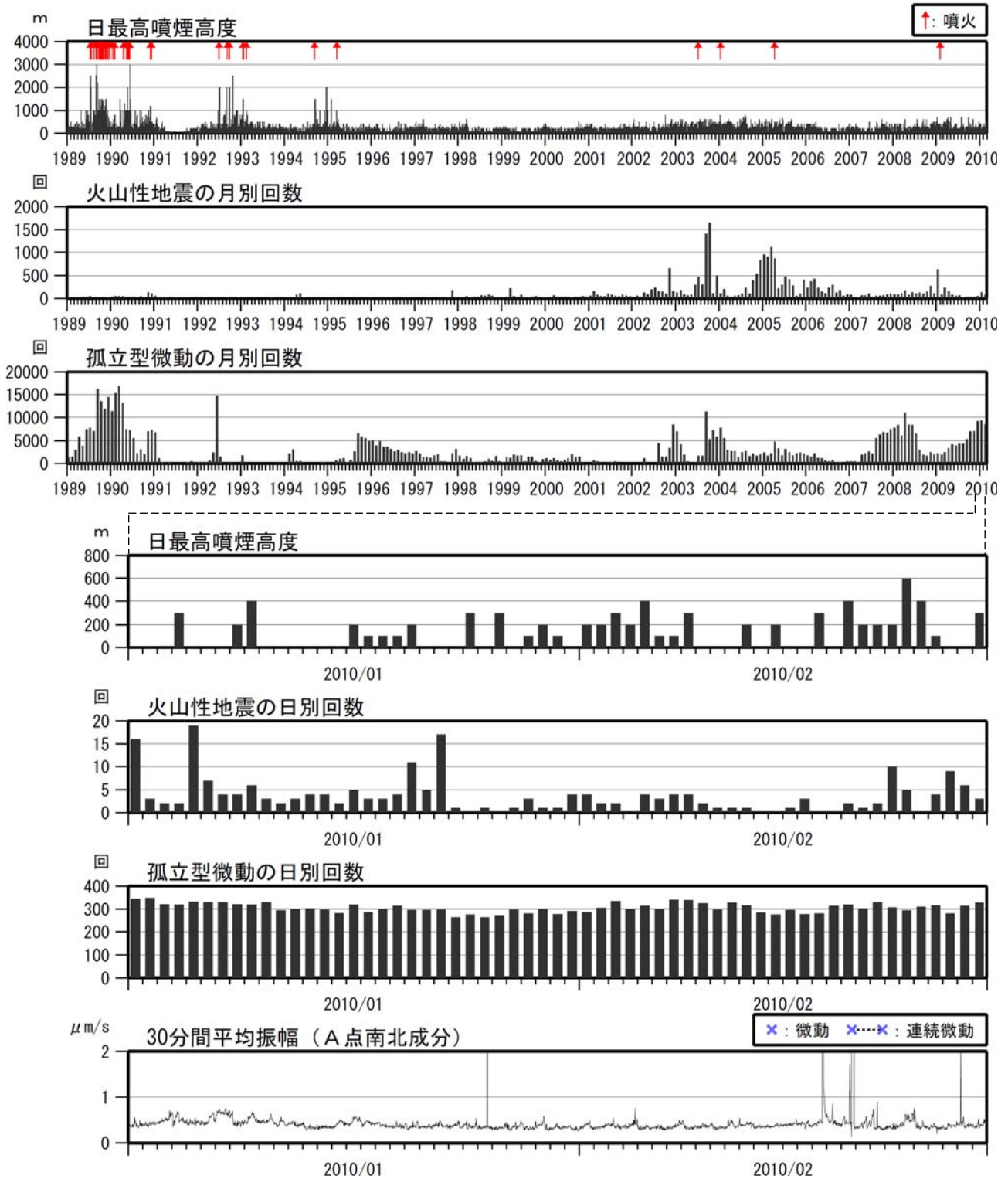
図 2 阿蘇山 火山活動経過図（1989 年 1 月～2010 年 2 月）
