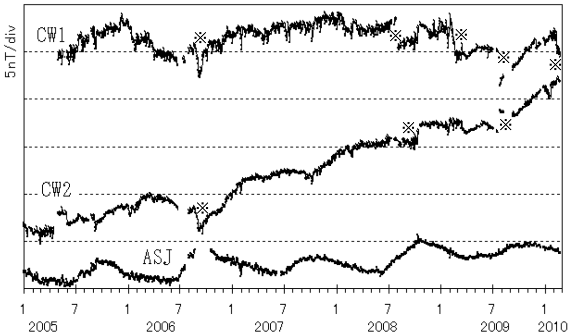
図 7 阿蘇山 阿蘇山麓 (AHK) を基準とした阿蘇山中岳火口周辺の全磁力変化
