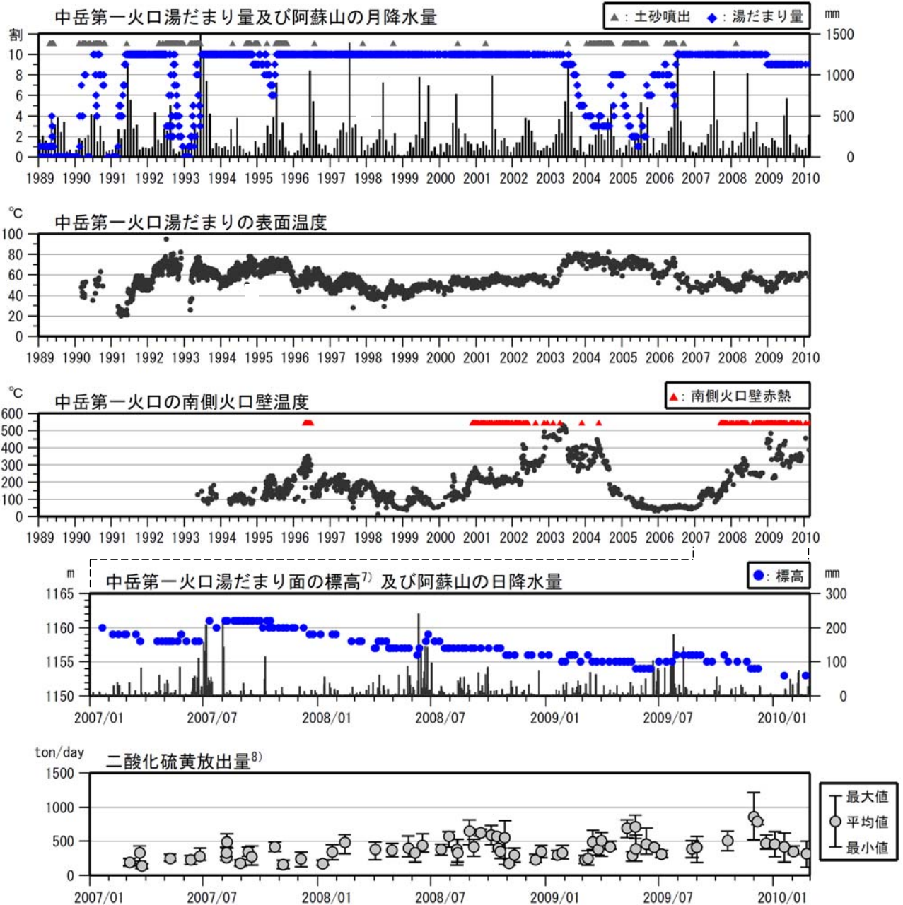
図 3 阿蘇山 火山活動経過図（1989 年 1 月～2010 年 2 月）
