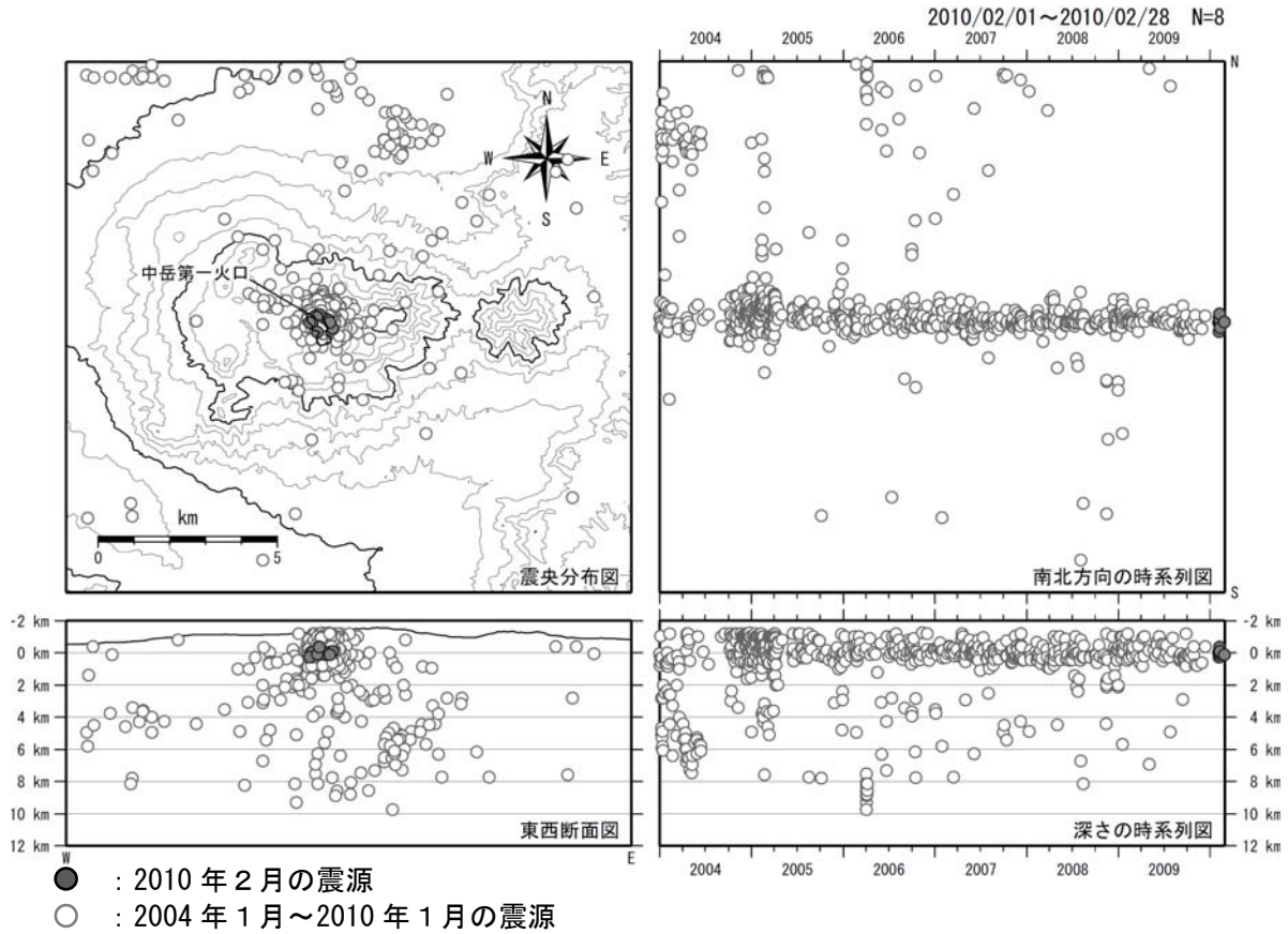
図 4※ 阿蘇山 震源分布図 (2004 年 1 月～2010 年 2 月)
