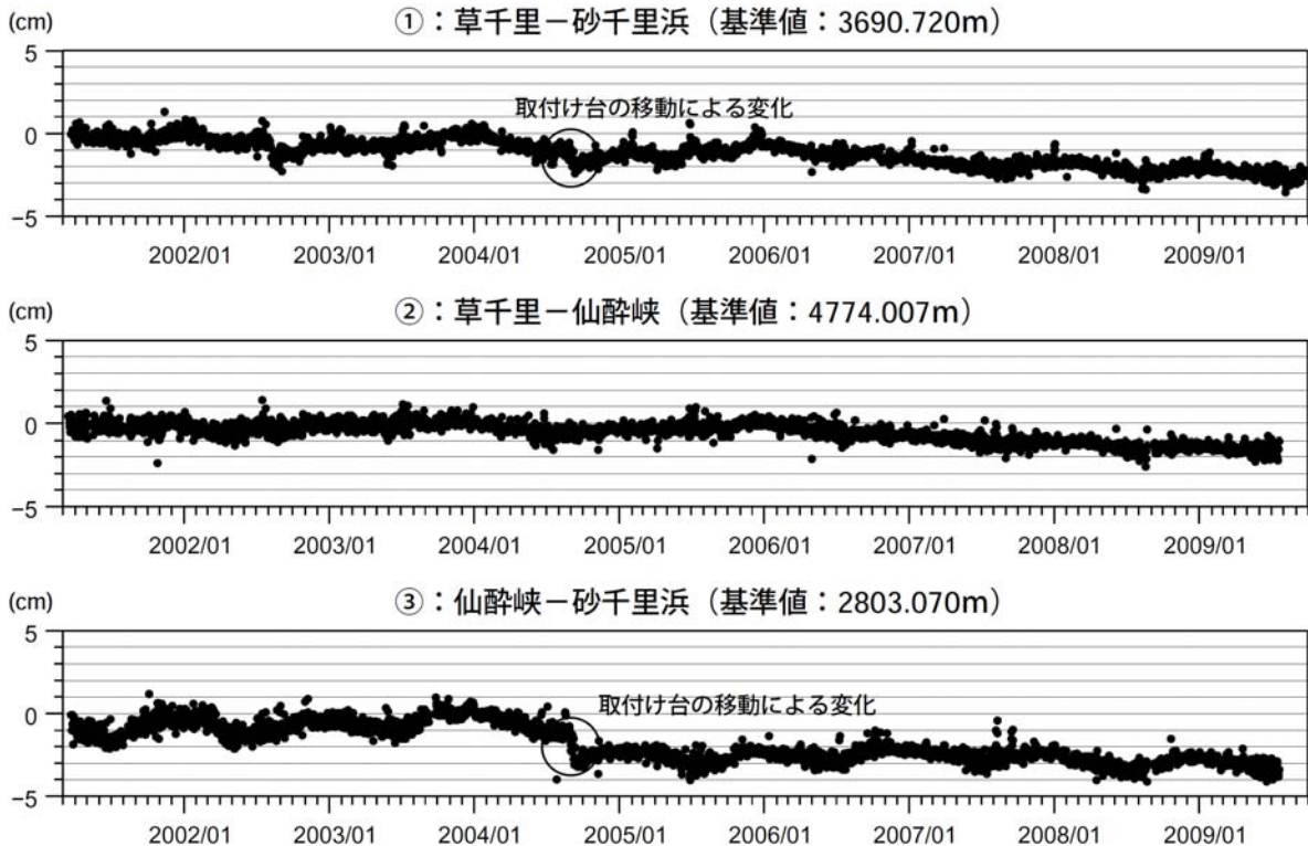
図 5 阿蘇山 GPS連続観測による基線長変化 (2001 年 3 月~2009 年 9 月)
