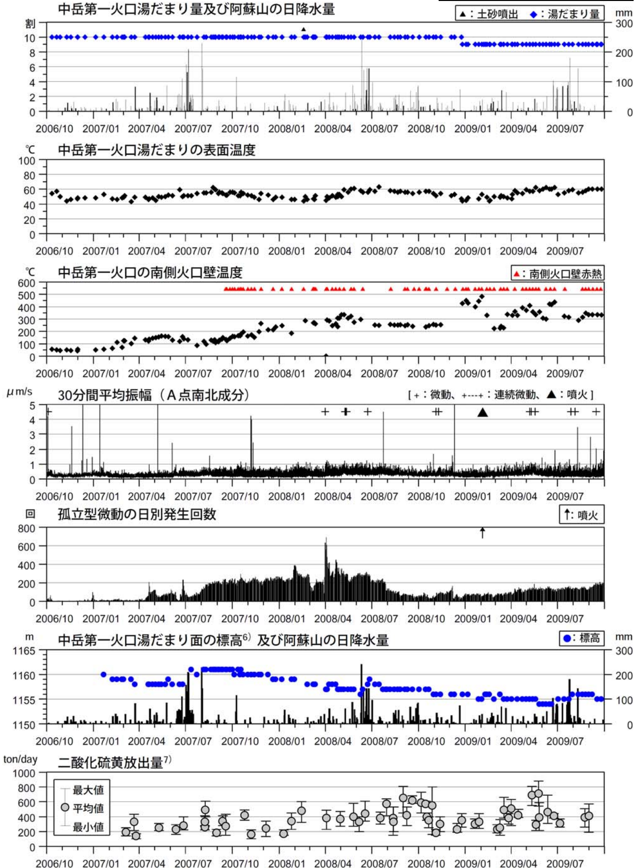
図3 阿蘇山 火山活動経過図（2006年7月～2009年9月）
