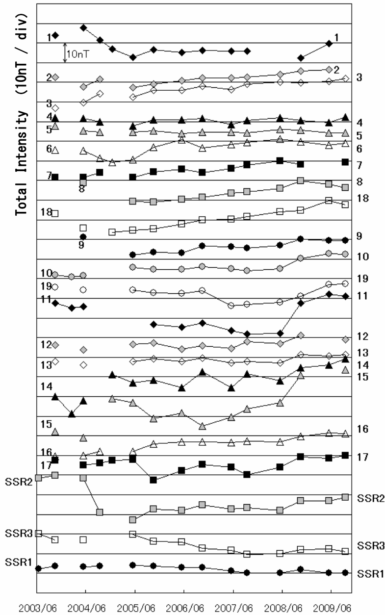
図 8 阿蘇山 阿蘇山麓 (AHK) を基準とした繰返し観測点における阿蘇中岳火口周辺の全磁力変化 (2003 年 6 月～2009 年 9 月)
