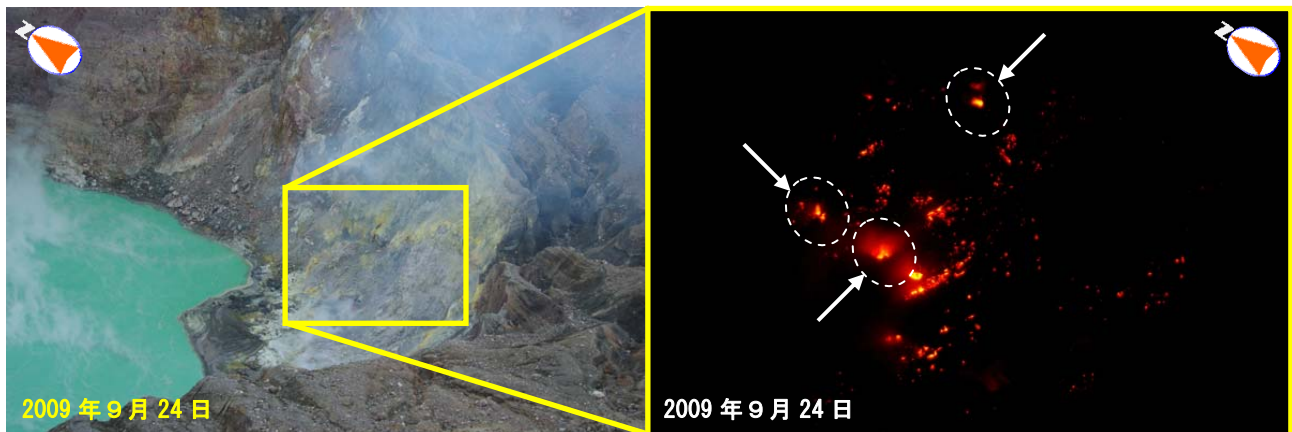
図 10 阿蘇山 夜間に実施した現地調査の状況 南側火口壁の矢印部分で高さ約 2 m の火炎現象を観測しました。
