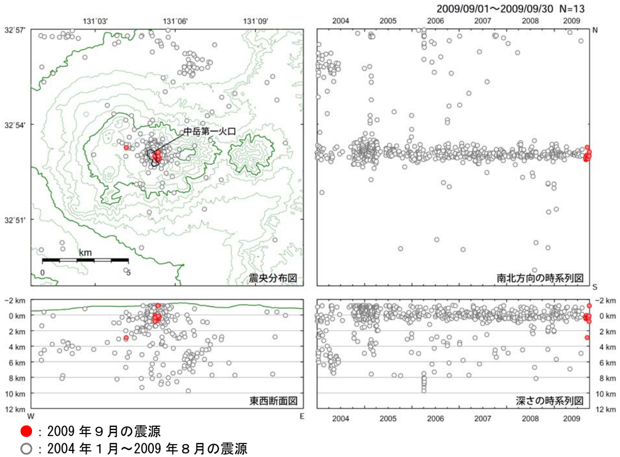
図 4 ※ 阿蘇山 震源分布図 (2004 年 1 月~2009 年 9 月)
