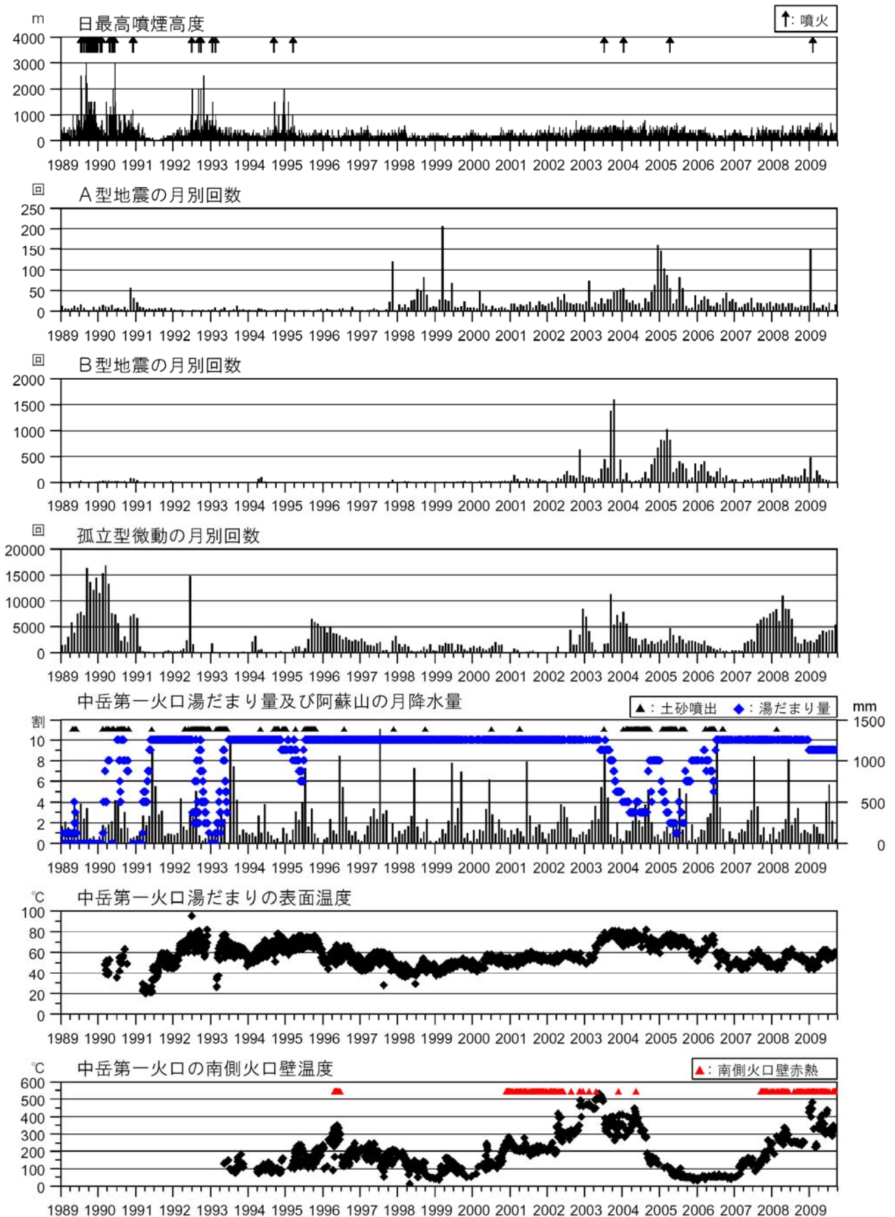
図2 阿蘇山 火山活動経過図（1989年1月～2009年9月）
