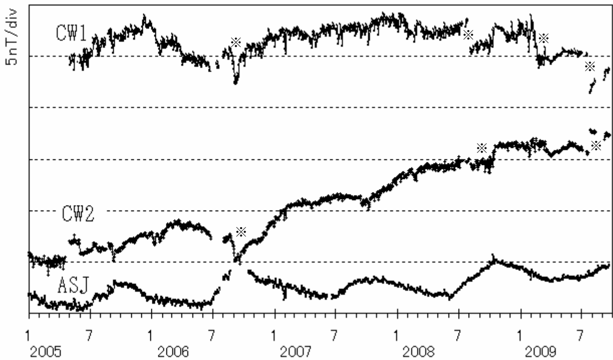
図 7 阿蘇山 阿蘇山麓 (AHK) を基準とした阿蘇中岳火口周辺の全磁力変化 (2005 年 1 月～2009 年 9 月)
