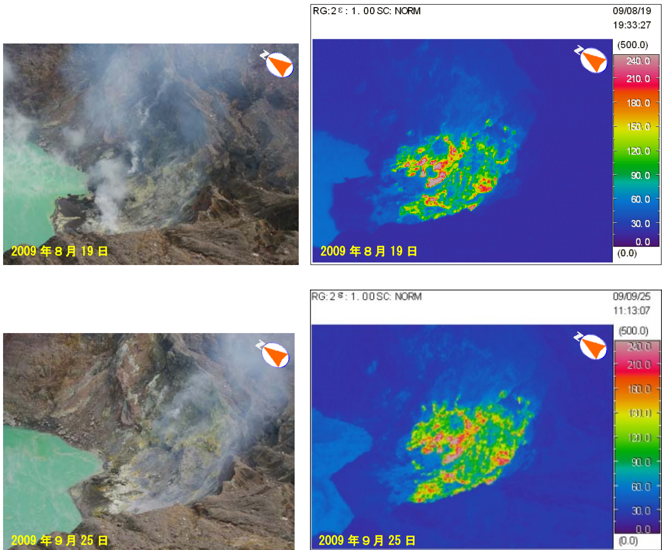
図 9 阿蘇山 赤外熱映像装置 8) による中岳第一火口南側火口壁の地表面温度分布 8月19日と比べて熱異常域の分布に大きな変化はありませんでした。
