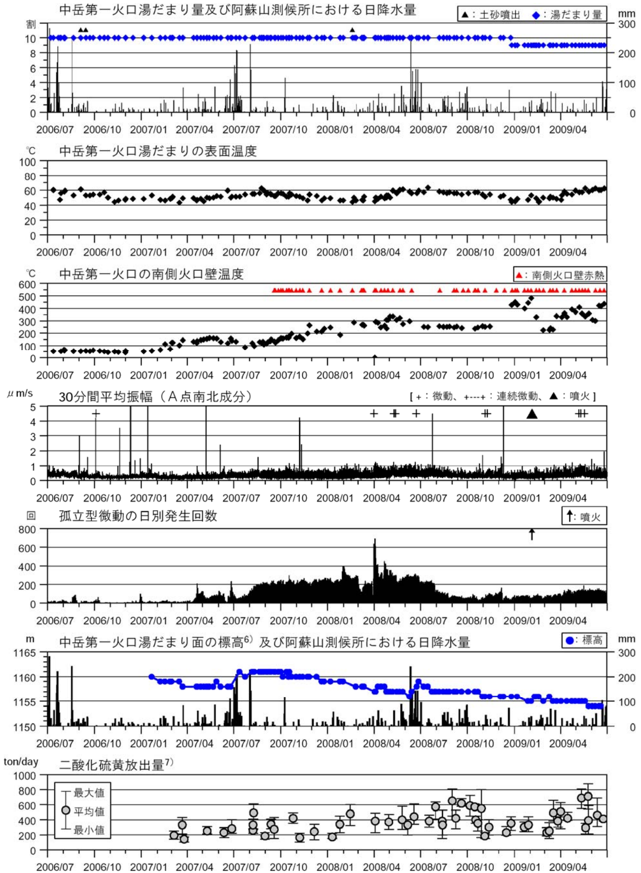
図3 阿蘇山 火山活動経過図（2006年7月～2009年6月） ・湯だまりの表面温度は60～62℃（5月：57～62℃）でした。 ・湯だまりの量は2007年10月頃から緩やかに減少しています。
