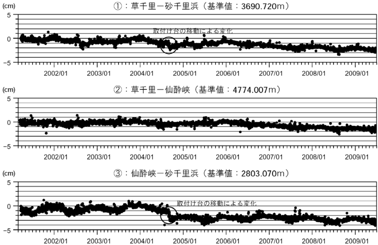
図 5 阿蘇山 GPS連続観測による基線長変化（2001 年 3 月～2009 年 6 月） 基線の長期的な収縮傾向が続いています。
