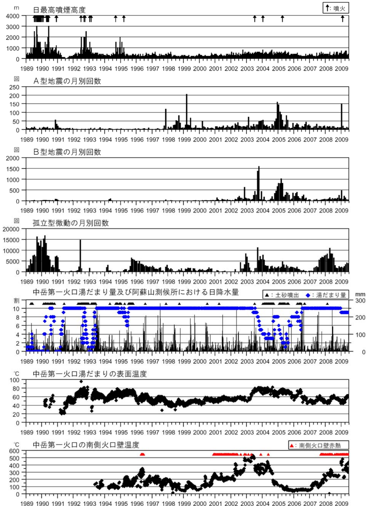
図2 阿蘇山 火山活動経過図（1989年1月～2009年6月）
