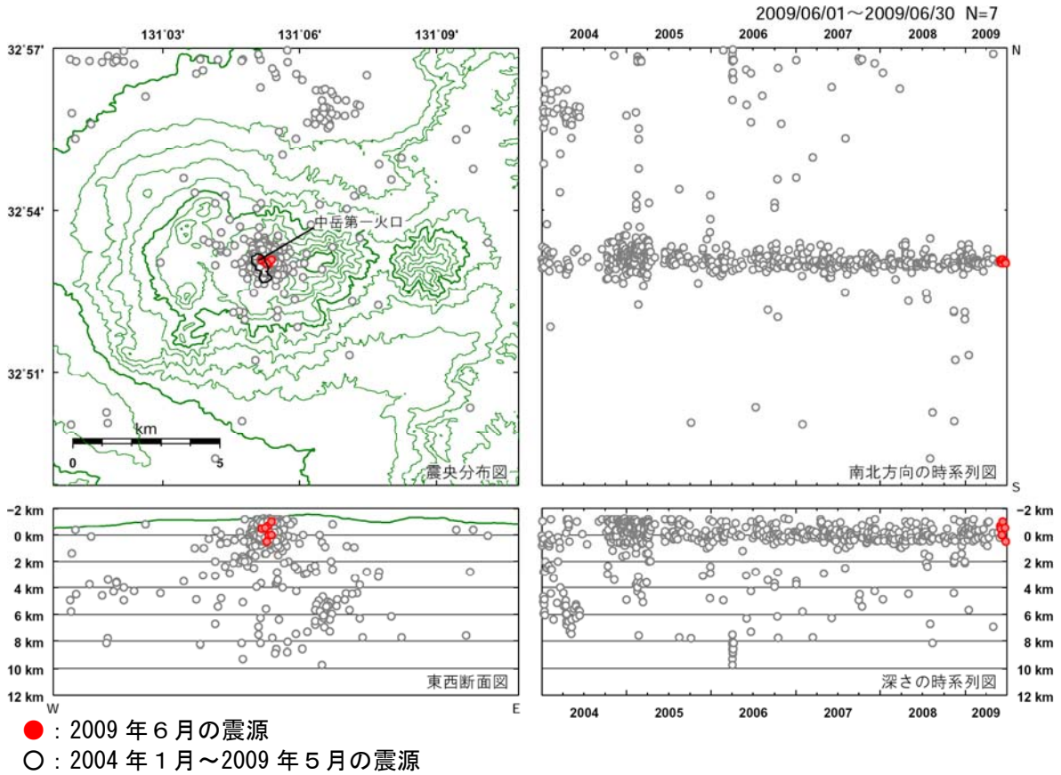
図 4※ 阿蘇山 震源分布図（2004 年 1 月～2009 年 6 月） 火山性地震の震源は中岳第一火口付近のごく浅いところに分布しました。
