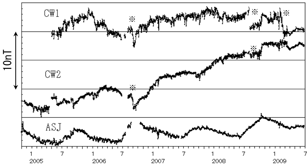
図 7 阿蘇山 阿蘇山麓 (AHK) を基準とした阿蘇中岳火口周辺の全磁力変化 (2004 年 11 月～2009 年 6 月)
