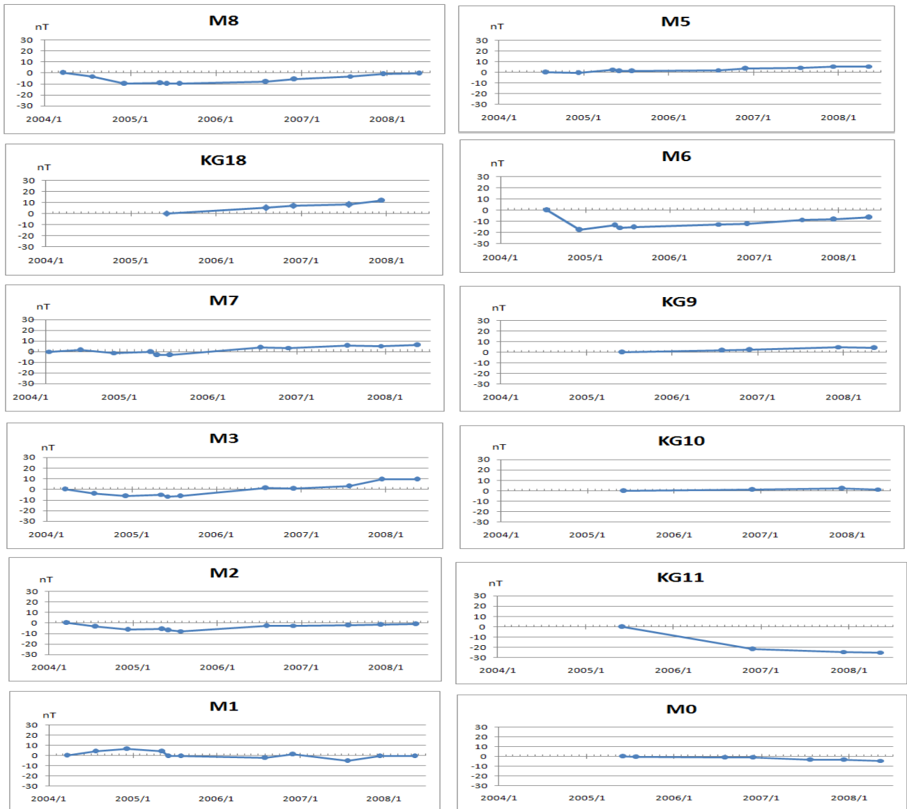
図12 全磁力繰返し観測結果(2004年3月~2008年5月)
