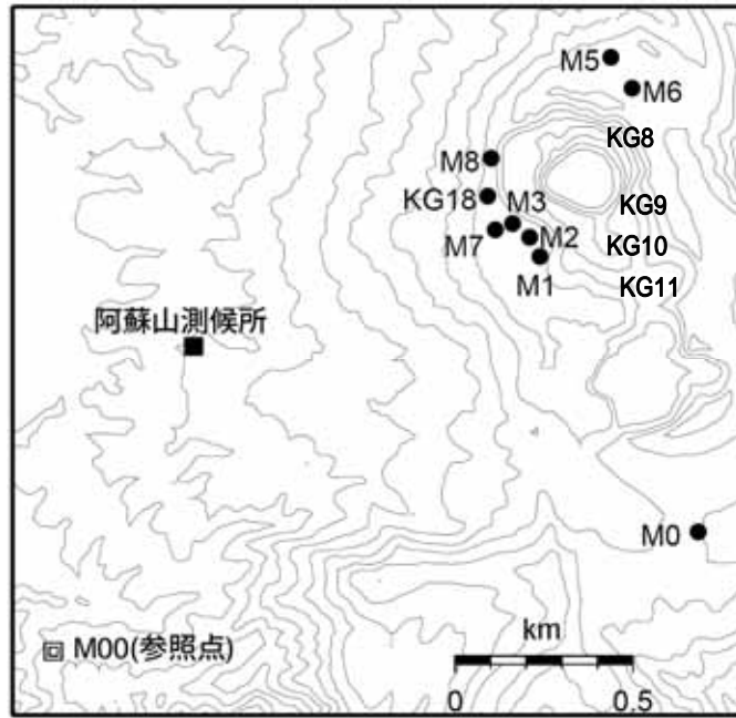
図11 阿蘇山 全磁力繰返観測点配置図
