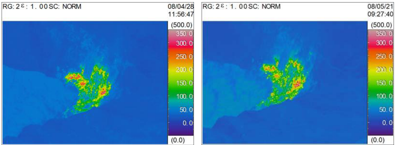
図14 阿蘇山 中岳第一火口南側火口壁の状況(左:2008年4月28日、右:2008年5月21日南西側より撮影) ・赤外熱映像装置 8) では熱領域の拡がりに大きな変化はありません。
