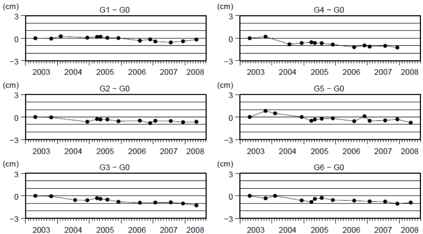
図8 阿蘇山のGPS繰返し観測による基線長変化(2003年4月1日~2008年5月)
