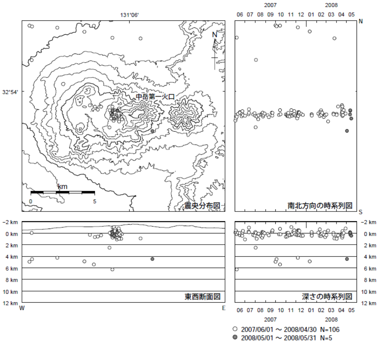
図1 阿蘇山 震源分布図(2007年6月~2008年5月)
