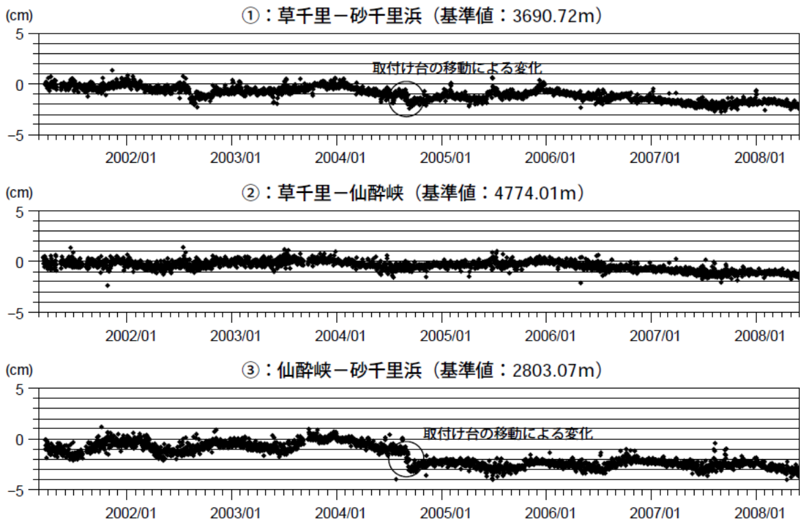
図5 阿蘇山 GPS連続観測による基線長変化(2001年3月15日~2008年5月31日)
