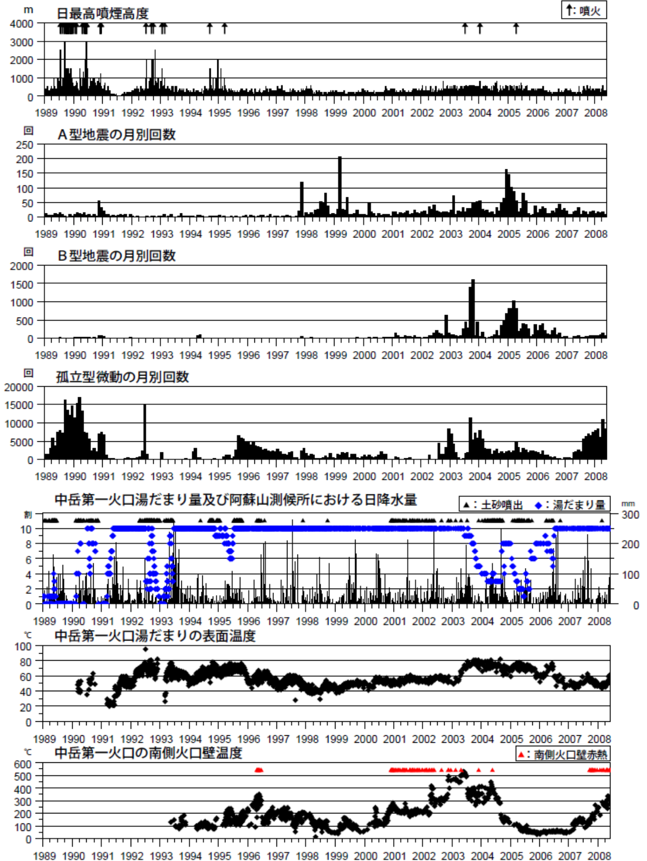
図2 阿蘇山 火山活動経過図(1989年1月～2008年5月)
