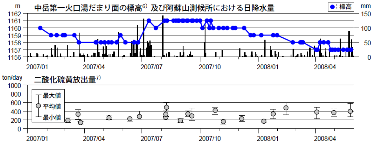
図4 阿蘇山 火山活動経過図(2007年1月～2008年5月)
