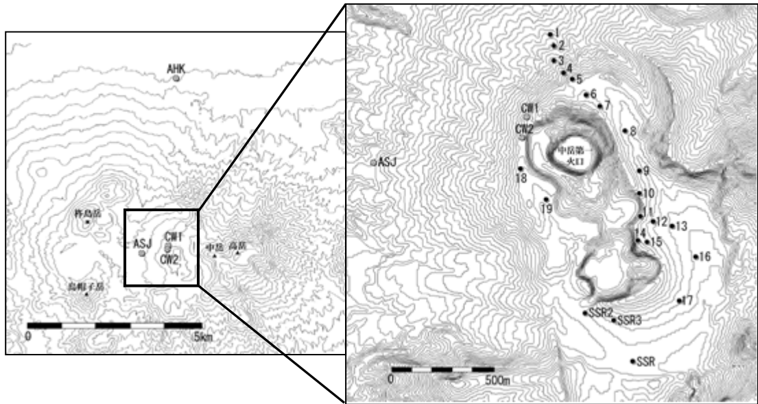
図9 阿蘇山の全磁力観測点配置図( ○ : 連続観測点 ● : 繰返し観測点)
