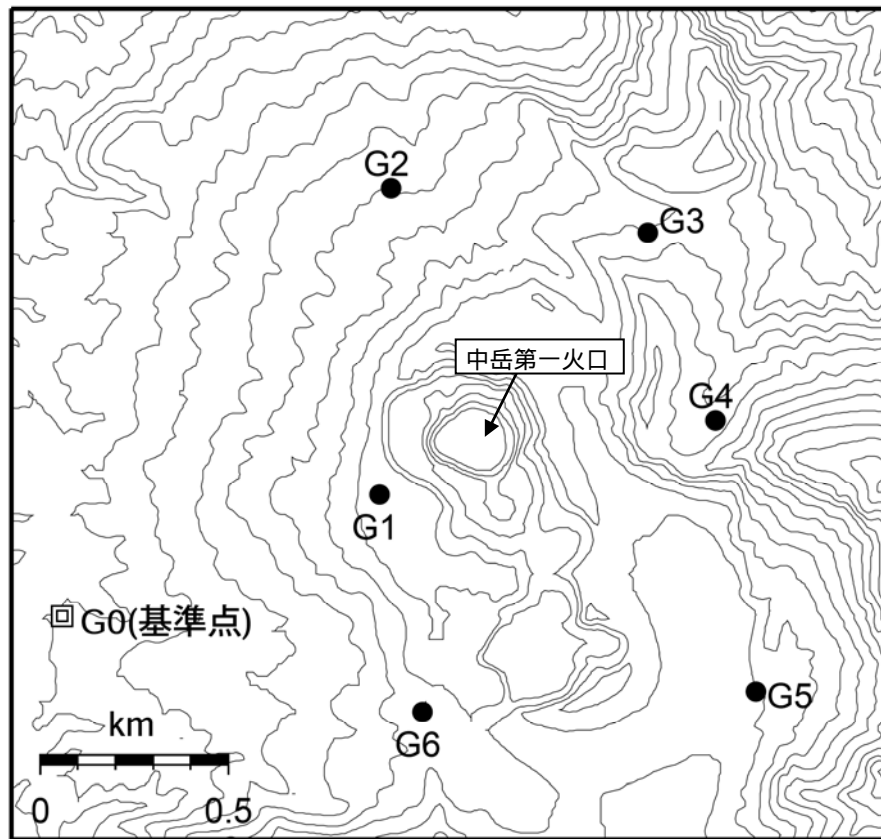
図7 阿蘇山 GPS 繰返し観測点配置図
