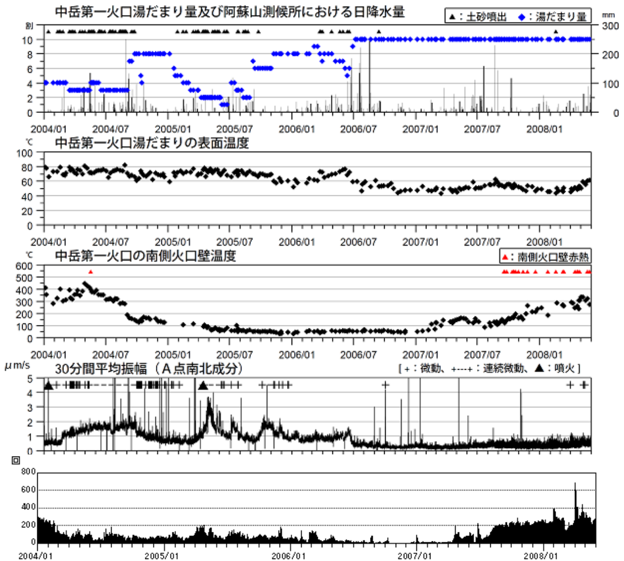
図3 阿蘇山 火山活動経過図(2004年1月～2008年5月)
