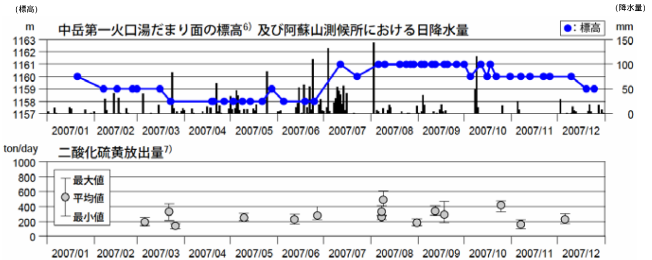
図4 阿蘇山 火山活動経過図(2007年1月～2007年12月)
