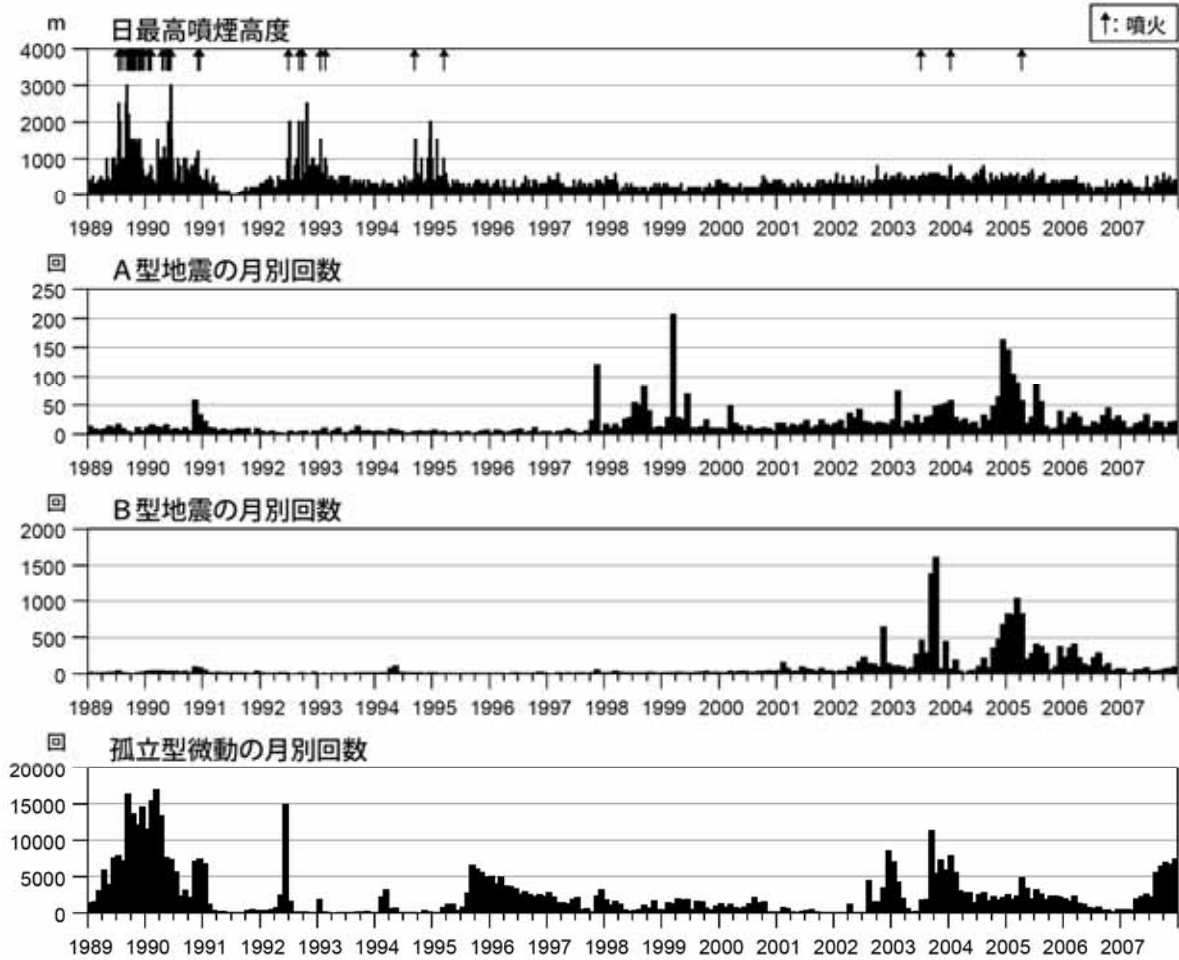
図1 阿蘇山 火山活動経過図(1989年1月1日～2007年12月31日)
