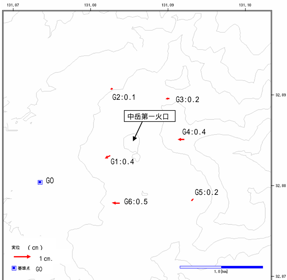
図 7 阿蘇山 GPS 観測点 G 0 を固定点としたベクトル図(2005 年 11 月 ~ 2007 年 12 月)
