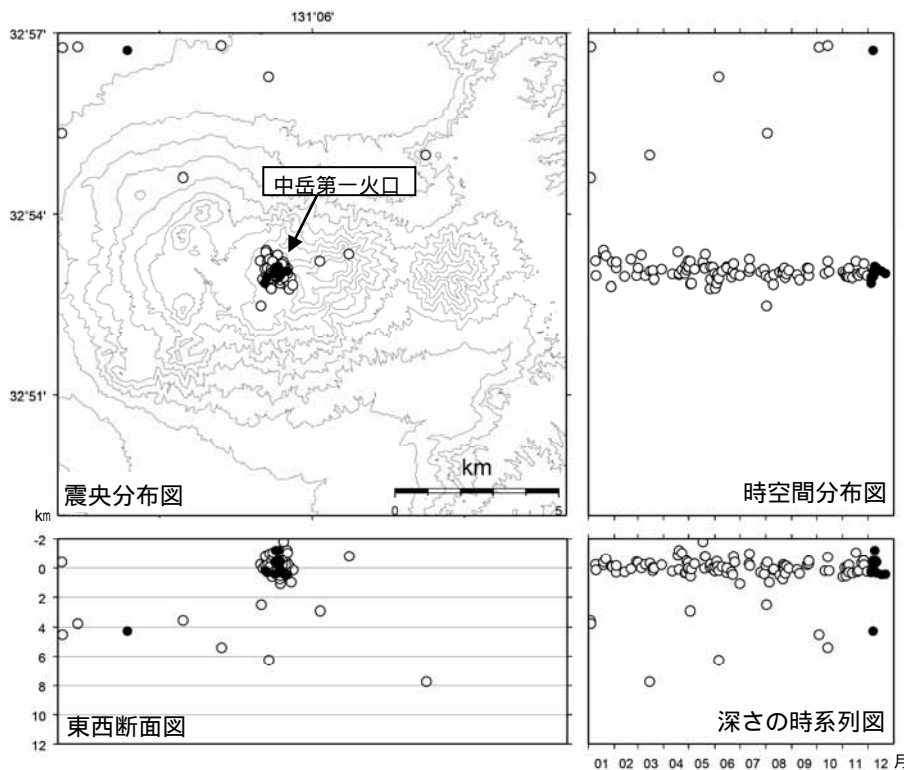
図2 阿蘇山 震源分布図 (2007年1月～2007年12月) 火山性地震の震源は、主に中岳第一火口付近のごく浅い所に分布しました。
