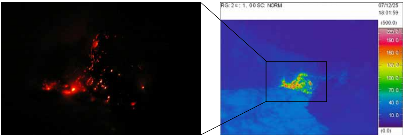
図13 阿蘇山 中岳第一火口南側火口壁の赤熱状況 (2007年12月25日、北側より撮影)
