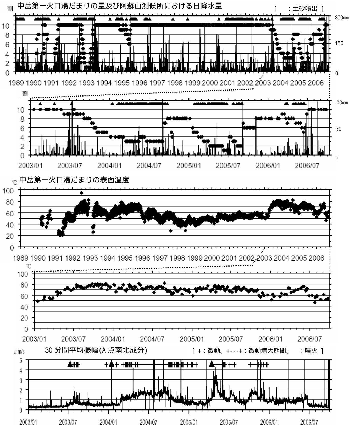
図3 火山活動経過図(1989年1月1日~2006年9月30日)
