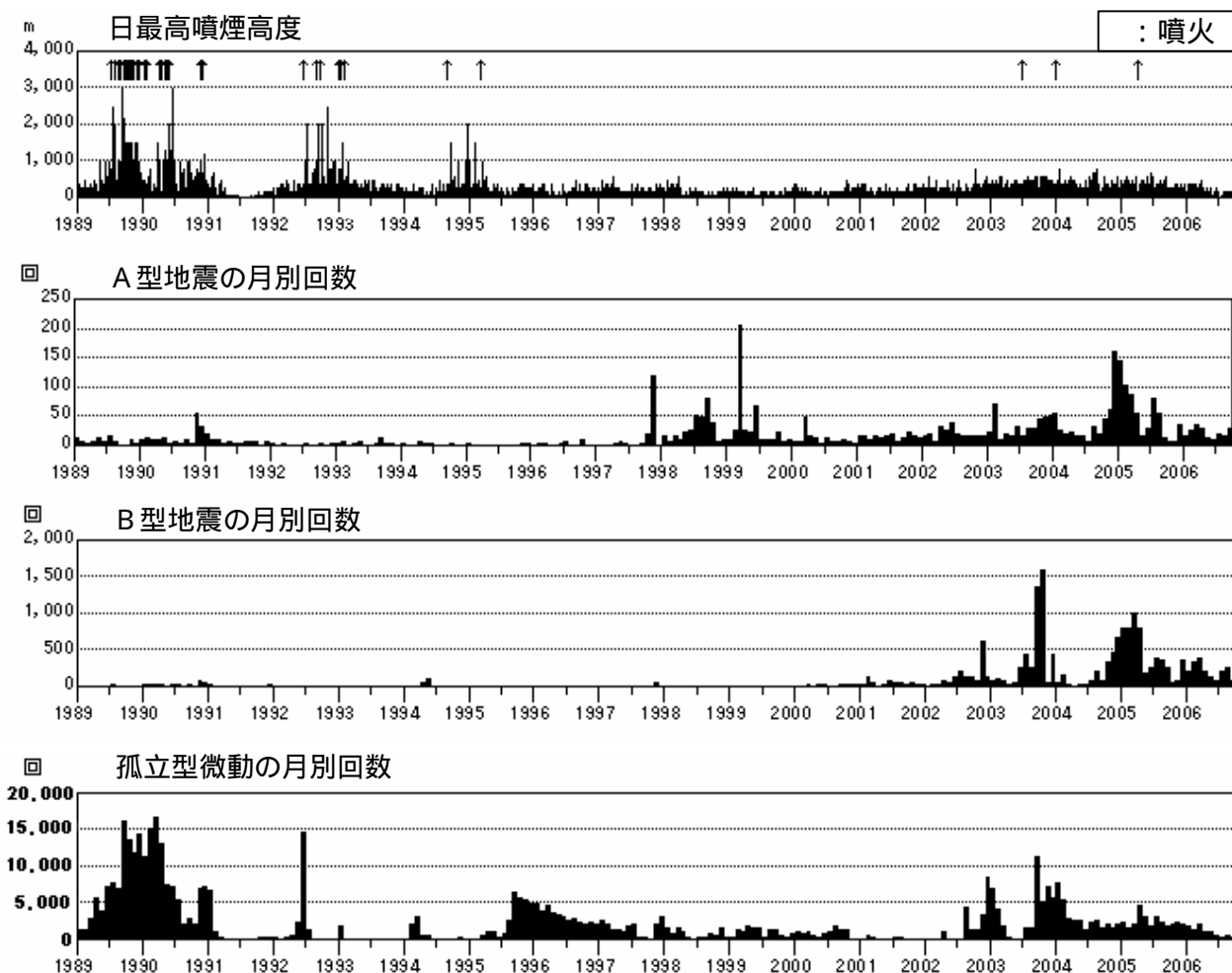
図 1 火山活動経過図(1989年1月1日～2006年9月30日)
