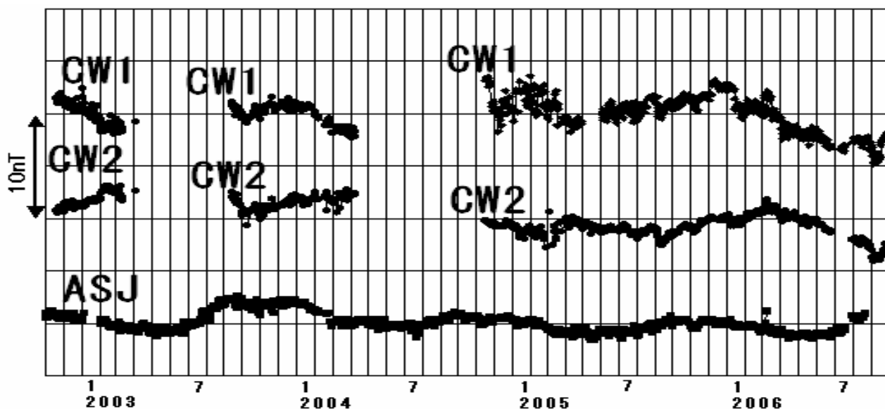
図7 全磁力連続観測の結果(2002年11月～2006年9月)
