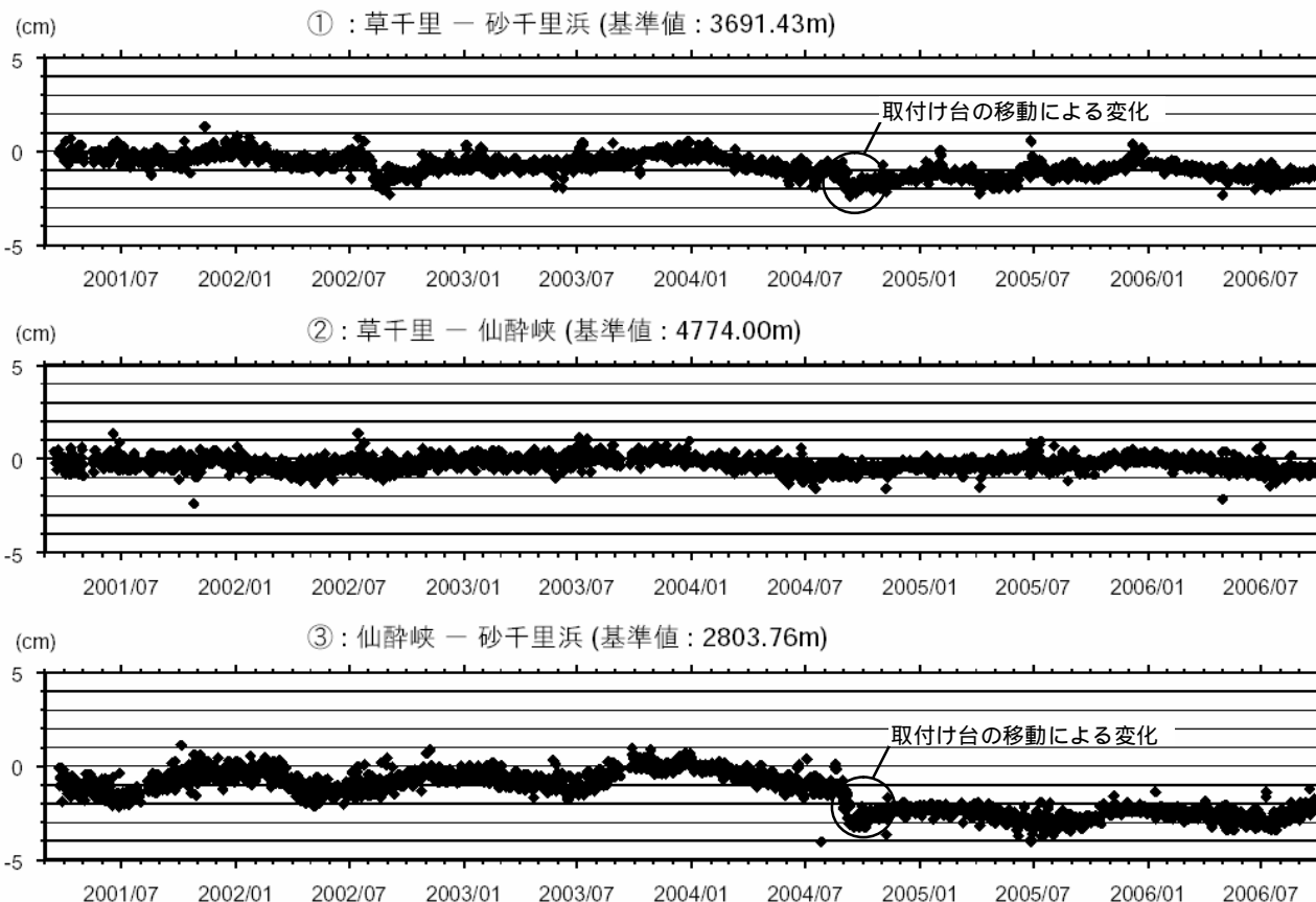
図5 GPS 連続観測による基線長変化(2001 年 3 月 15 日 ~ 2006 年 9 月 30 日) 各観測点間の基線長には、火山活動に起因するとみられる変化はありませんでした。 基線の番号は図 10 の ~ に対応しています。
