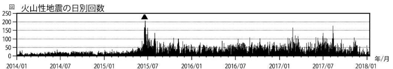
図2 浅間山 火山性地震の日別回数（2014年1月1日～2018年1月11日） （はごく小規模な噴火を示す）
