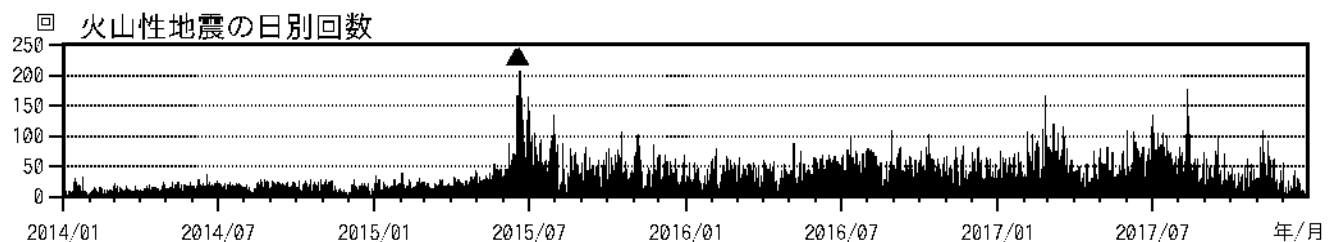
図2 浅間山 火山性地震の日別回数（2014年1月1日～2017年12月28日） （▲はごく小規模な噴火を示す）
