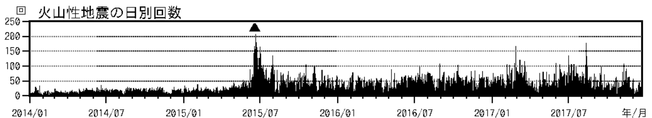
図2 浅間山 火山性地震の日別回数（2014年1月1日～2017年12月21日） （ はごく小規模な噴火を示す）
