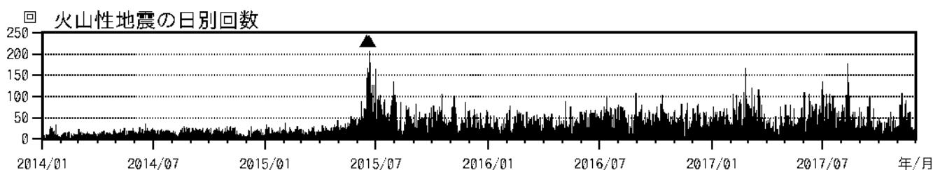
図2 浅間山 火山性地震の日別回数（2014年1月1日～2017年11月30日） （はごく小規模な噴火を示す）
