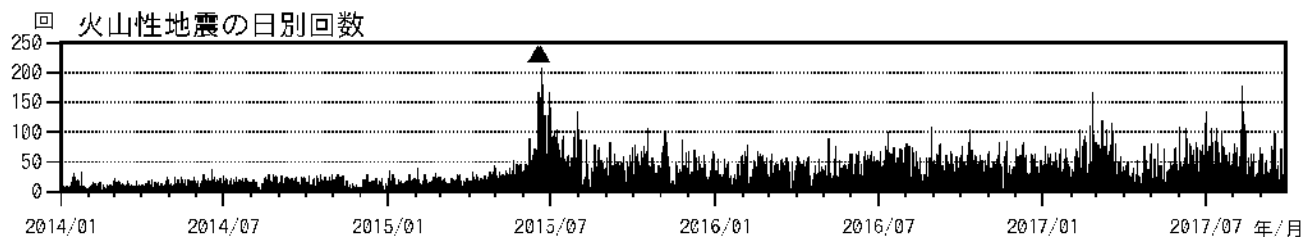
図2 浅間山 火山性地震の日別回数（2014年1月1日～2017年9月28日） （はごく小規模な噴火を示す）
