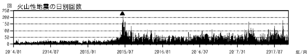
図2 浅間山 火山性地震の日別回数（2014年1月1日～2017年9月7日） （はごく小規模な噴火を示す）
