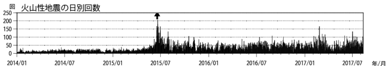
図2 浅間山 火山性地震の日別回数（2014年1月1日～2017年8月10日） （矢印はごく小規模な噴火を示す）
